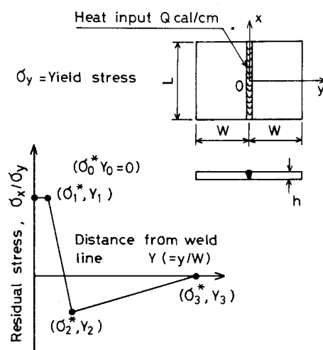
図4-12 平板の突合せ溶接継手の 残留応力分布特性
