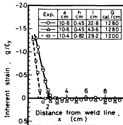
図3-6 鋼管寸法が全周溶接による固有歪におよぼす影響
