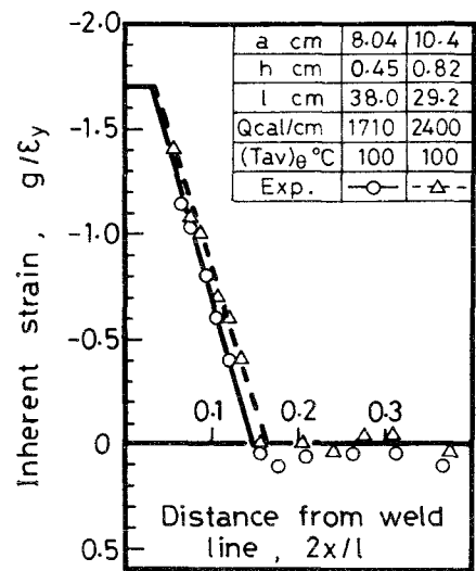
図4-13 全周溶接による固有歪分布と平均温度上昇量 (T_{av})_\theta の関係
