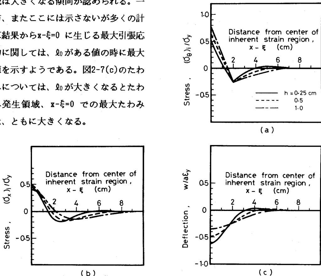
図2-8 板厚 h が応力と変形におよぼす影響 [(a), (b) 内表面での周, 軸方向応力 (c) たわみ変形]
