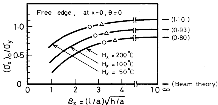
図6-8 中央断面の溶接線上の軸方向応力におよぼす寸法パラメータ \beta_x の影響
