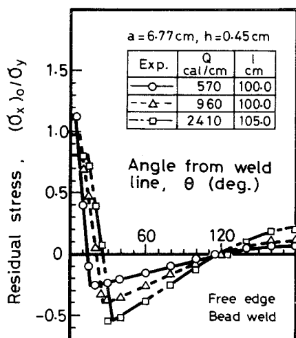
図3-17 溶接入熱が全長溶接による残留応力におよぼす影響
