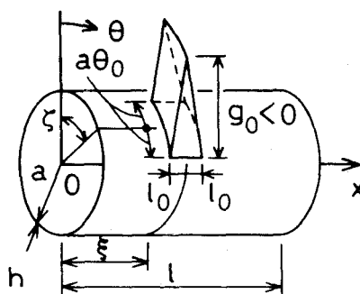
図2-5 長方形領域 2a\theta_0 \times 2l_0 に三角形 状固有歪が存在する薄肉円筒殻 (三角形モデル)
