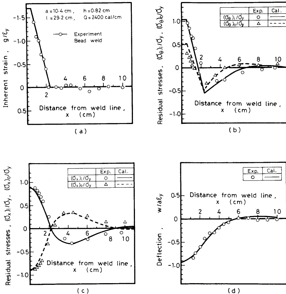
図4-5 全周溶接による応力・変形の計算結果と実験結果の比較
