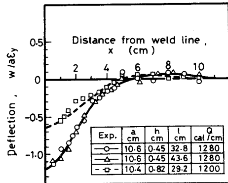
図3-10 鋼管寸法が全周溶接による 溶接変形におよぼす影響
