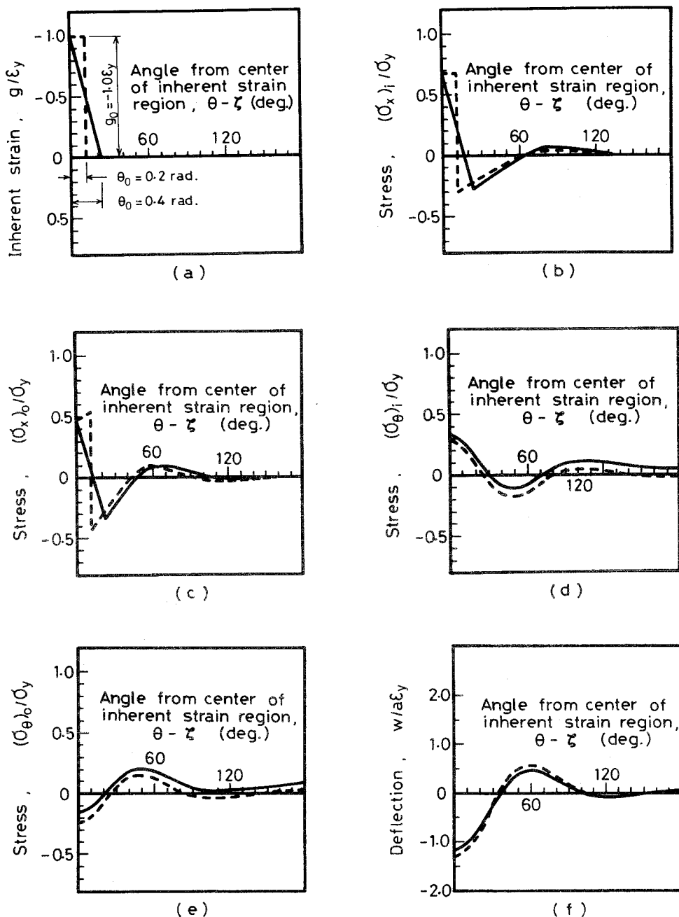
図2-13 固有歪分布形状が応力と変形におよぼす影響 [(a) 固有歪分布、(b),(c) 軸方向内外表面応力、(d),(e) 周方向内外表面応力、(f) たわみ変形]
