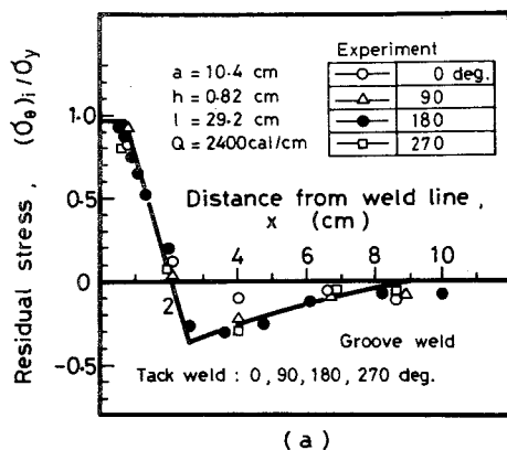
図3-11 全周溶接による残留応力と変形の軸対称性についての検討
