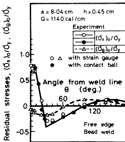
図3-16 中央断面での全長溶接による残留応力測定例
