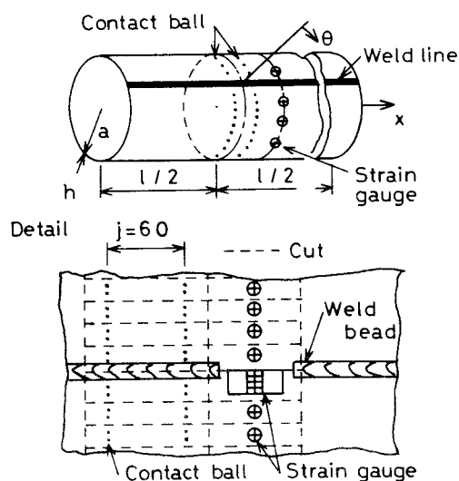
図3-4 軸方向溶接による固有歪と残留応力の測定法
