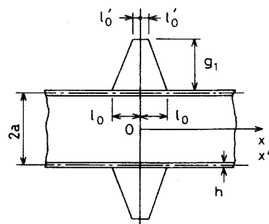
図6-2 軸対称の台形状固有歪が 作用する無限長円筒殻
