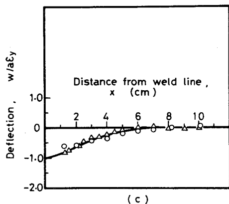
図3-12 全周溶接された鋼管のビード溶接とグループ溶接による固有歪、残留応力及び変形の差違
