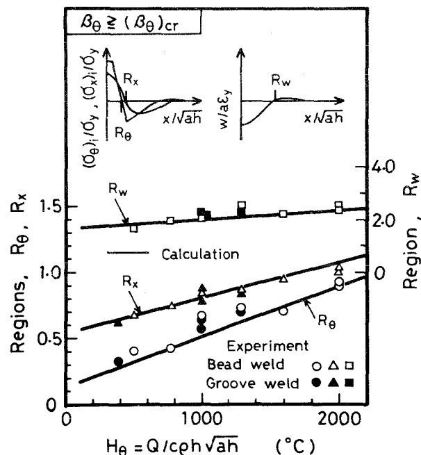
図6-6 引張残留応力及び負のたわみ変形の発生領域幅におよぼす入熱パラメータ H_0 の影響
