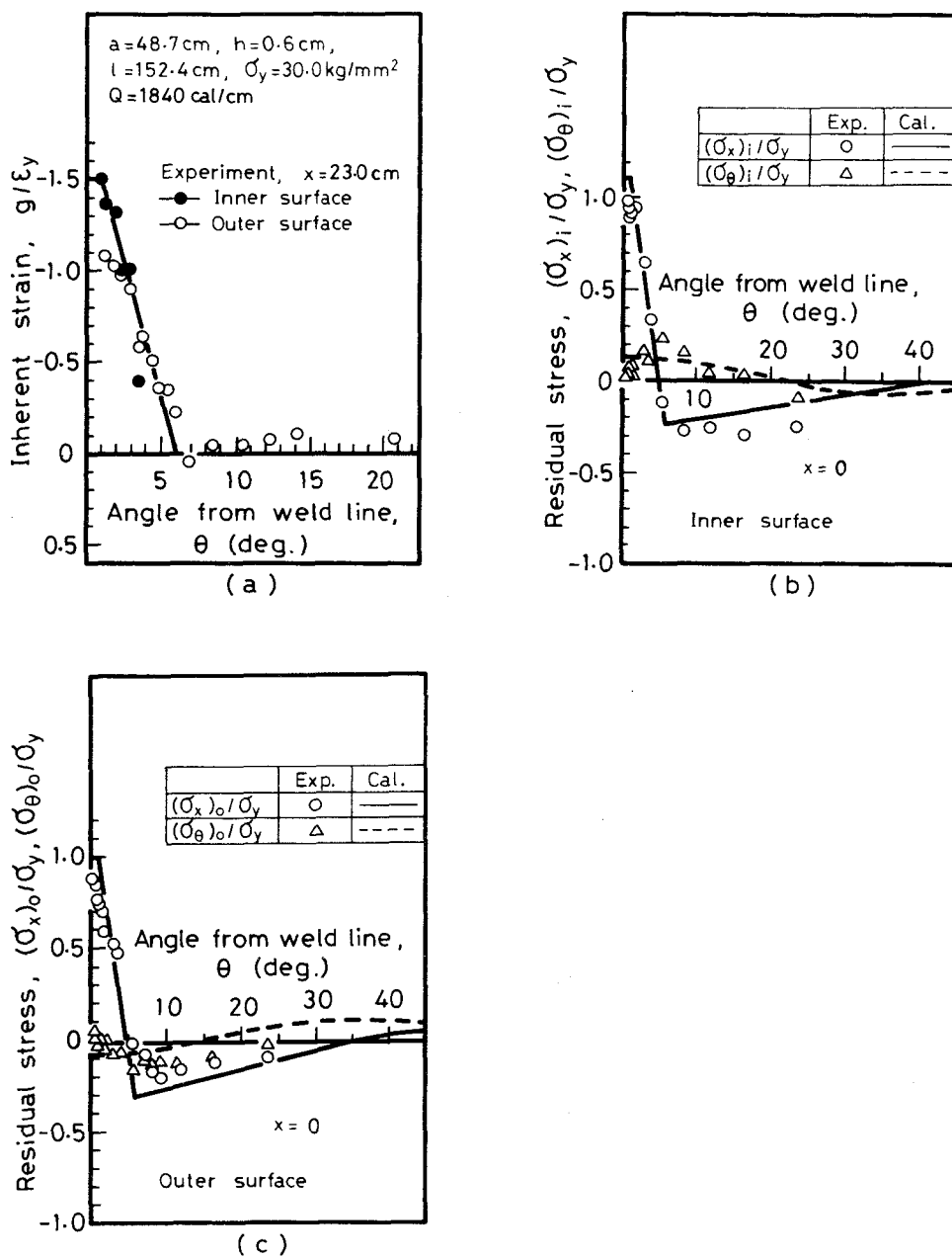
図4-10 全長溶接による応力・変形の計算結果と実験結果の比較
