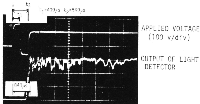
図 5-8 バンバン制御による応答波形 (ストッパなし) (横軸: 700 \mu s / div )
