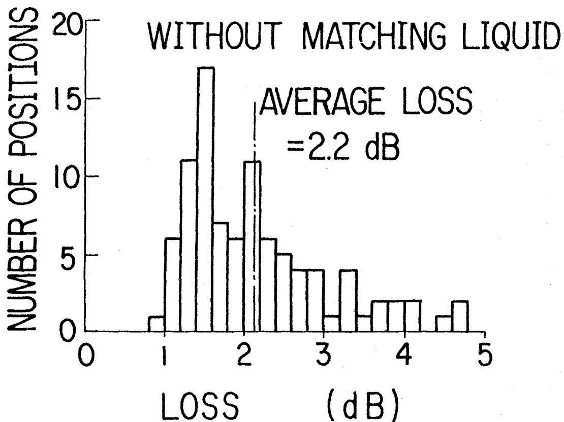
図 4-18 全接続点の損失分布 (マッティング液を用いない場合)
