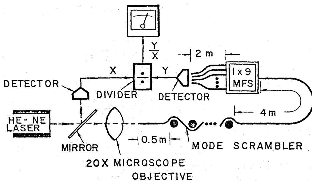
図 4 - 8 接続特性測定系
