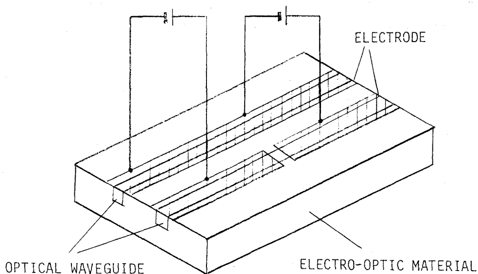
図6-1 2 \times 2 形スイッチの基本構成
