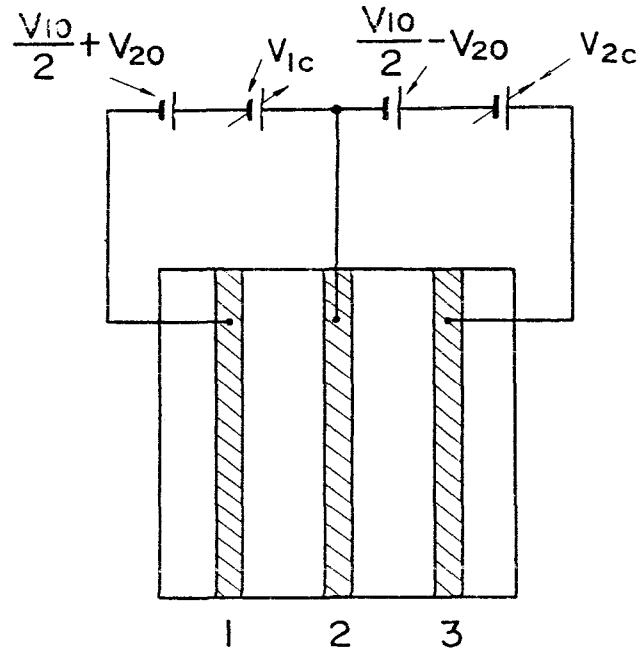
図 A - 5 伝搬定数差の補償電圧 V_{10} , V_{20} , 制御電圧 v_{1c} , v_{2c} の結線
