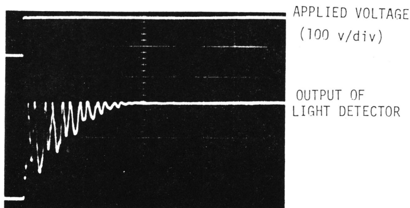
図 5-6 ±60 V のステップ電圧印加時の応答波形
