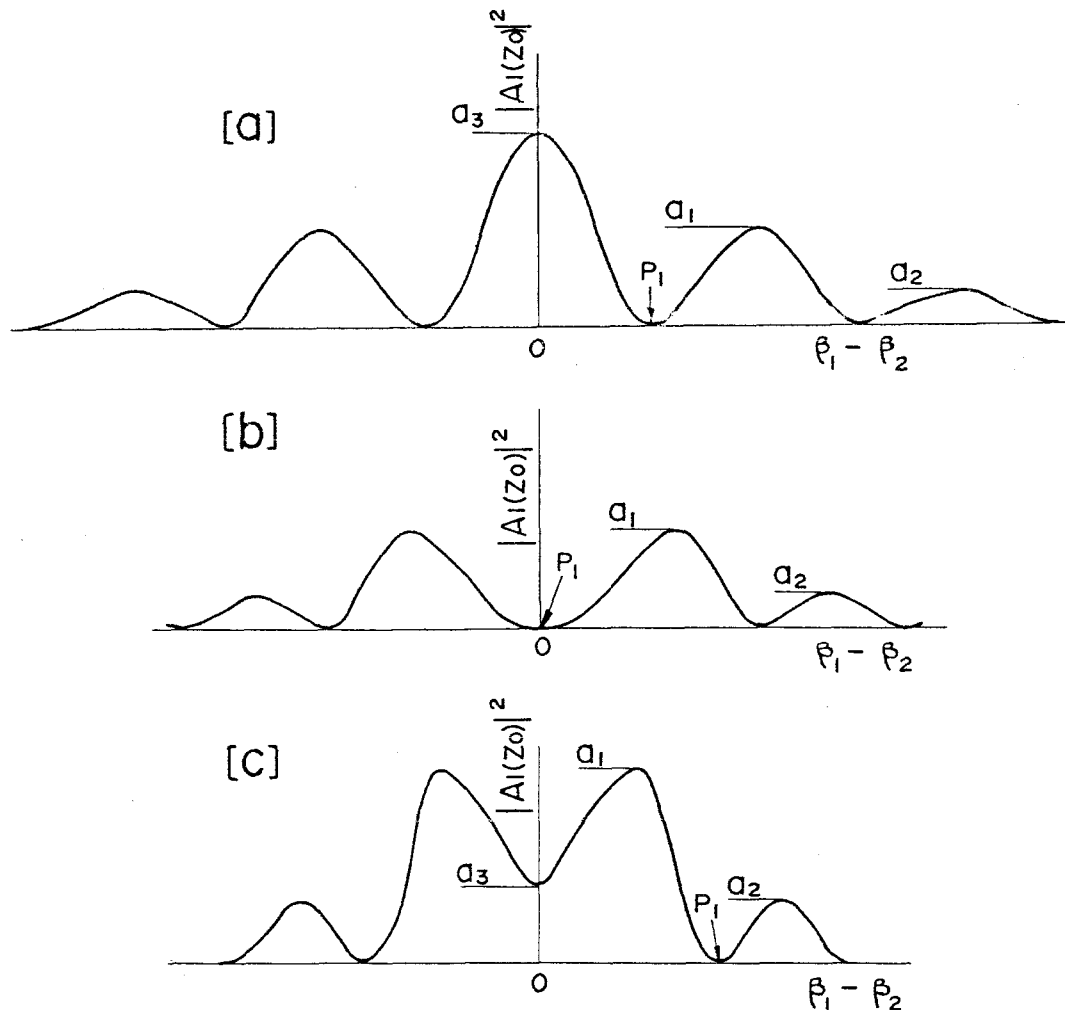
図 A - 4 (\beta_1 - \beta_2) と導波路 2 → 導波路 1 の伝達率
