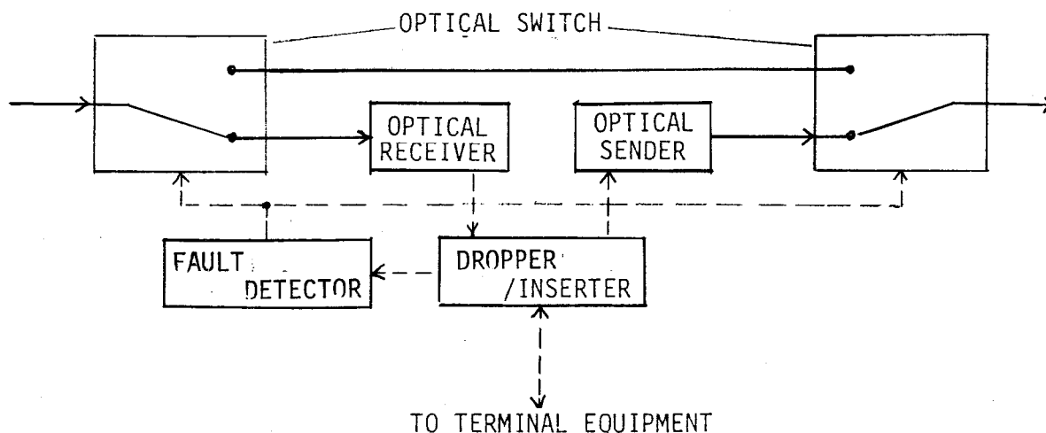
図 2-9 バイパス回路を有するアクティブノード
