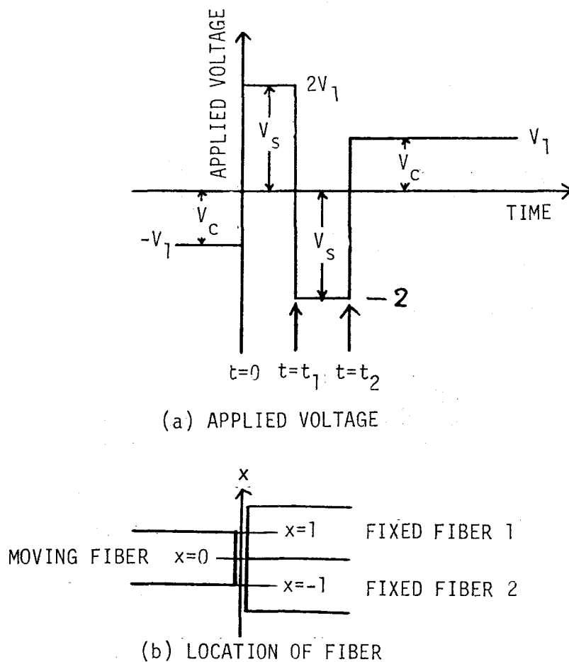
図5-7 バンバン制御による駆動
