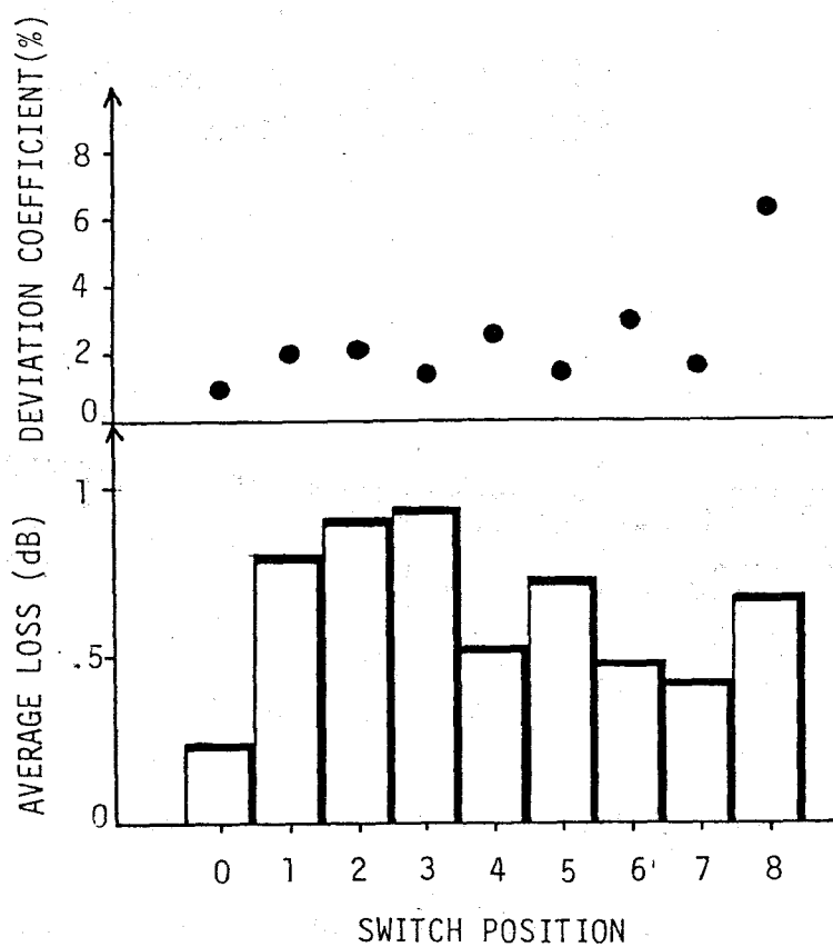
図 4 - 9 接続損失 (試作 1)
