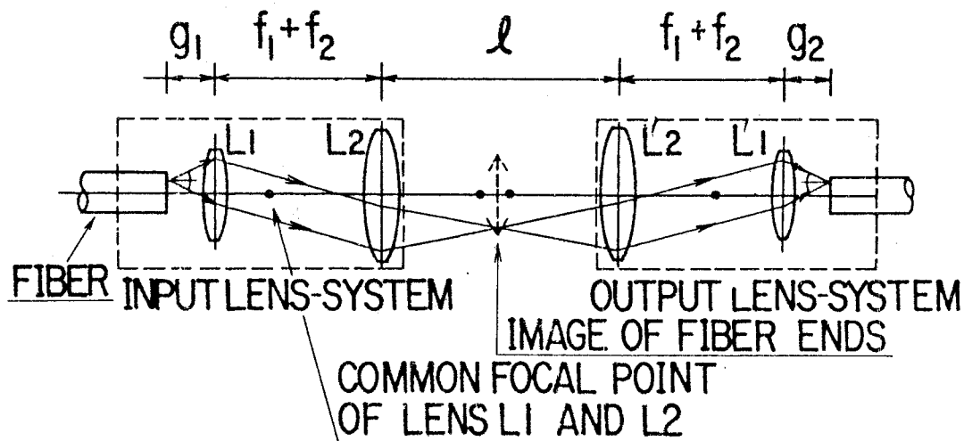
図 3-8 望遠光学系を用いた結合
