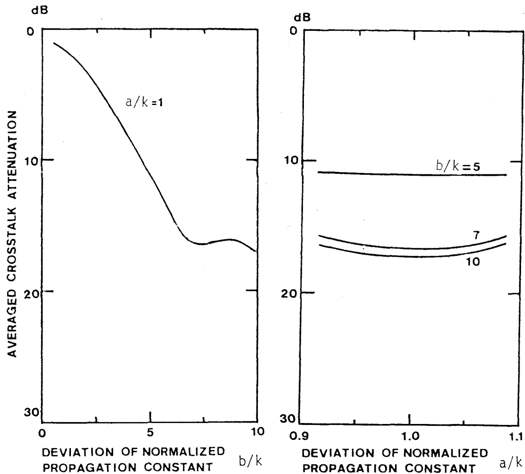
図6-7 伝搬定数差と平均クロストーク比
