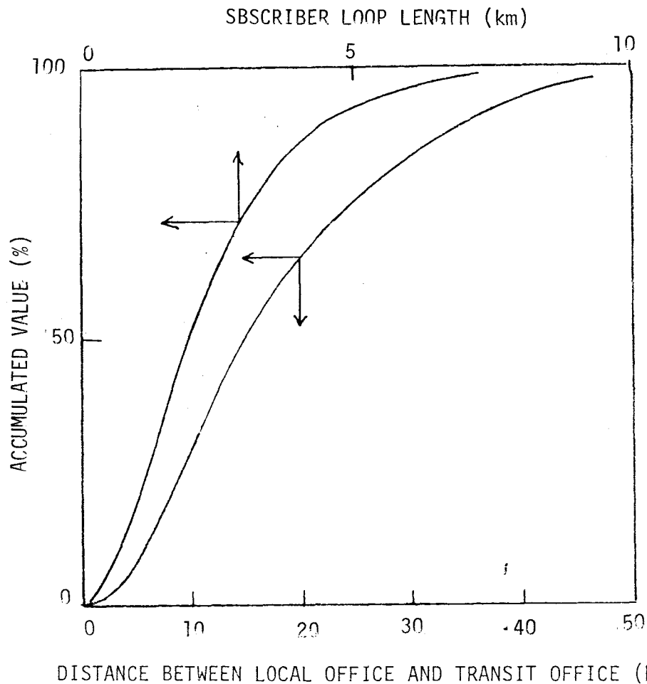
図 2-2 中継線および加入者線の距離の累積分布
