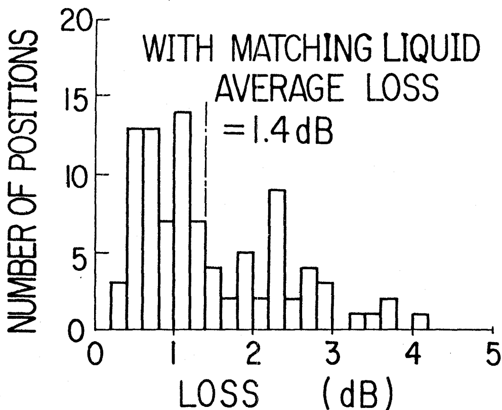
図 4-19 全接続点の損失分布 (マッティング液を用いた場合)
