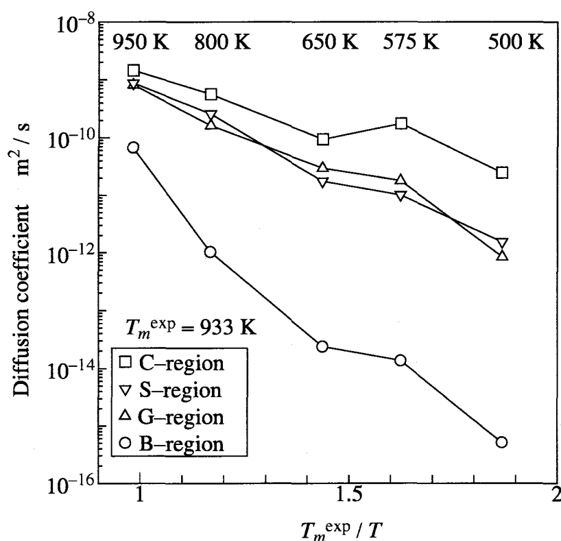
Fig. 5.12 Regional diffusion coefficient
