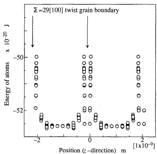
(d) \Sigma = 29[100] twist grain boundary
