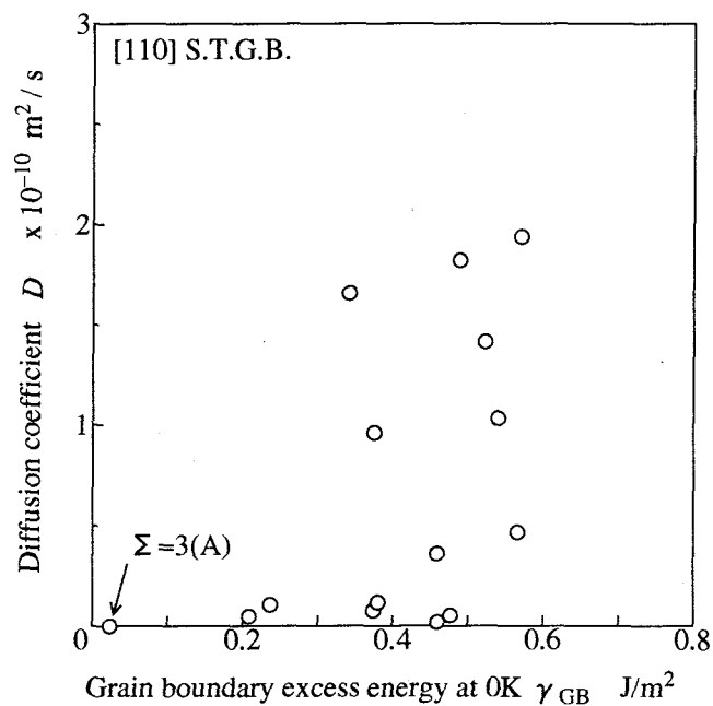
(a)[110] S.T.G.B.
