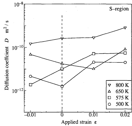
(b) S-region
