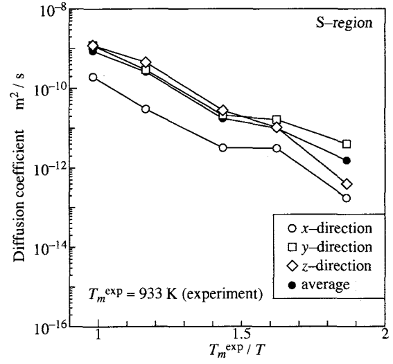
(b)S-region
