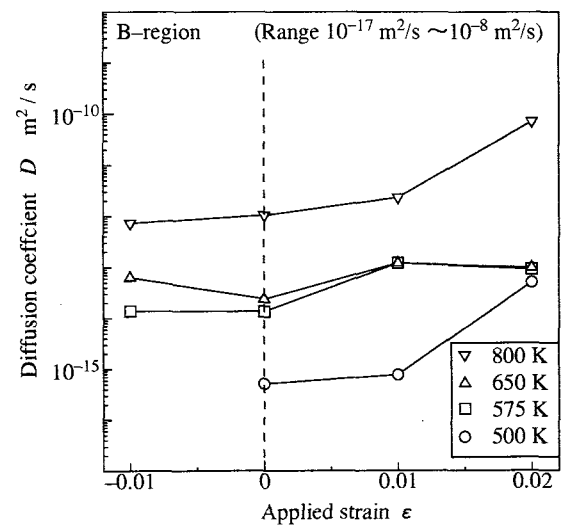
(d) B-region
