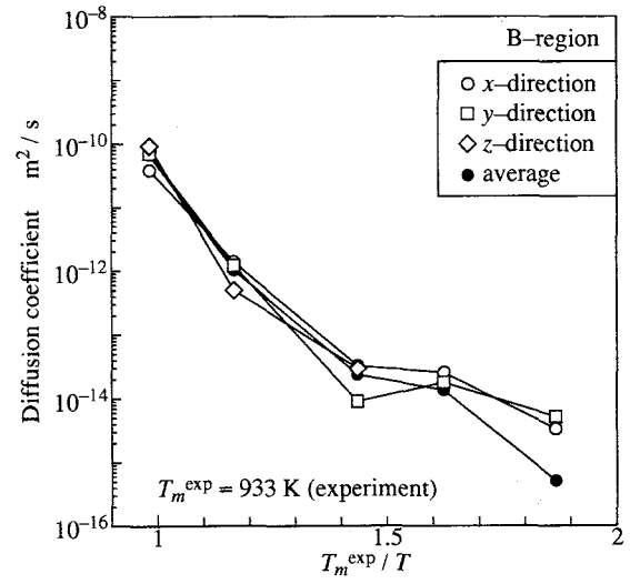
(d)B-region
