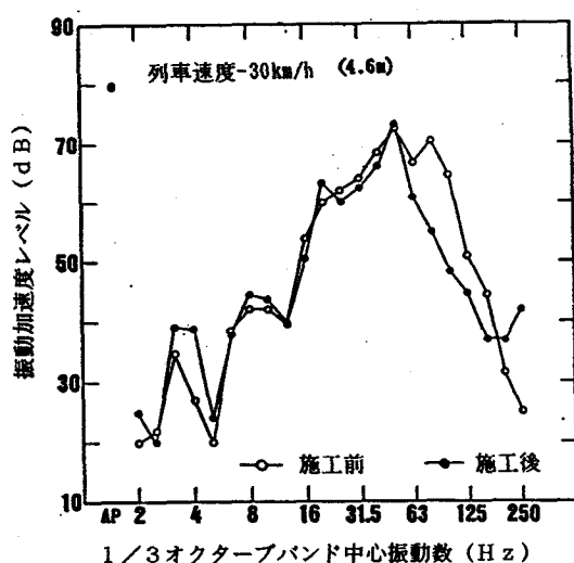
図7.76 地表の振動加速度スペクトル
