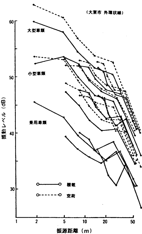
図5. 2 振動レベルの距離減衰 (2)
