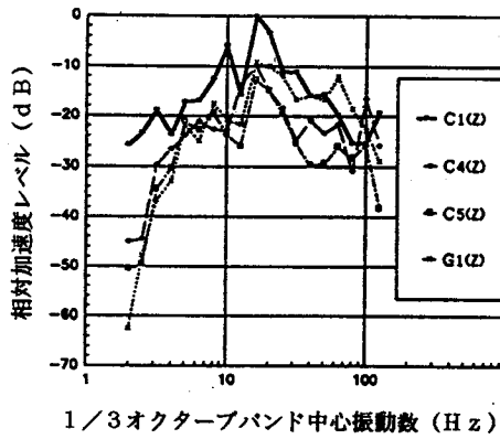
(b) EPS 盛土
