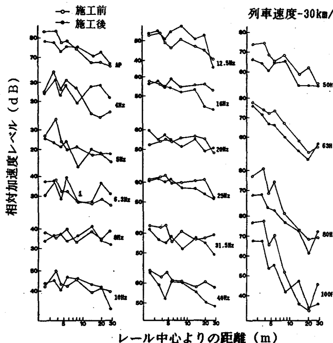
図6. 60 1/3オクターブバンド周波数ごとの距離減衰
