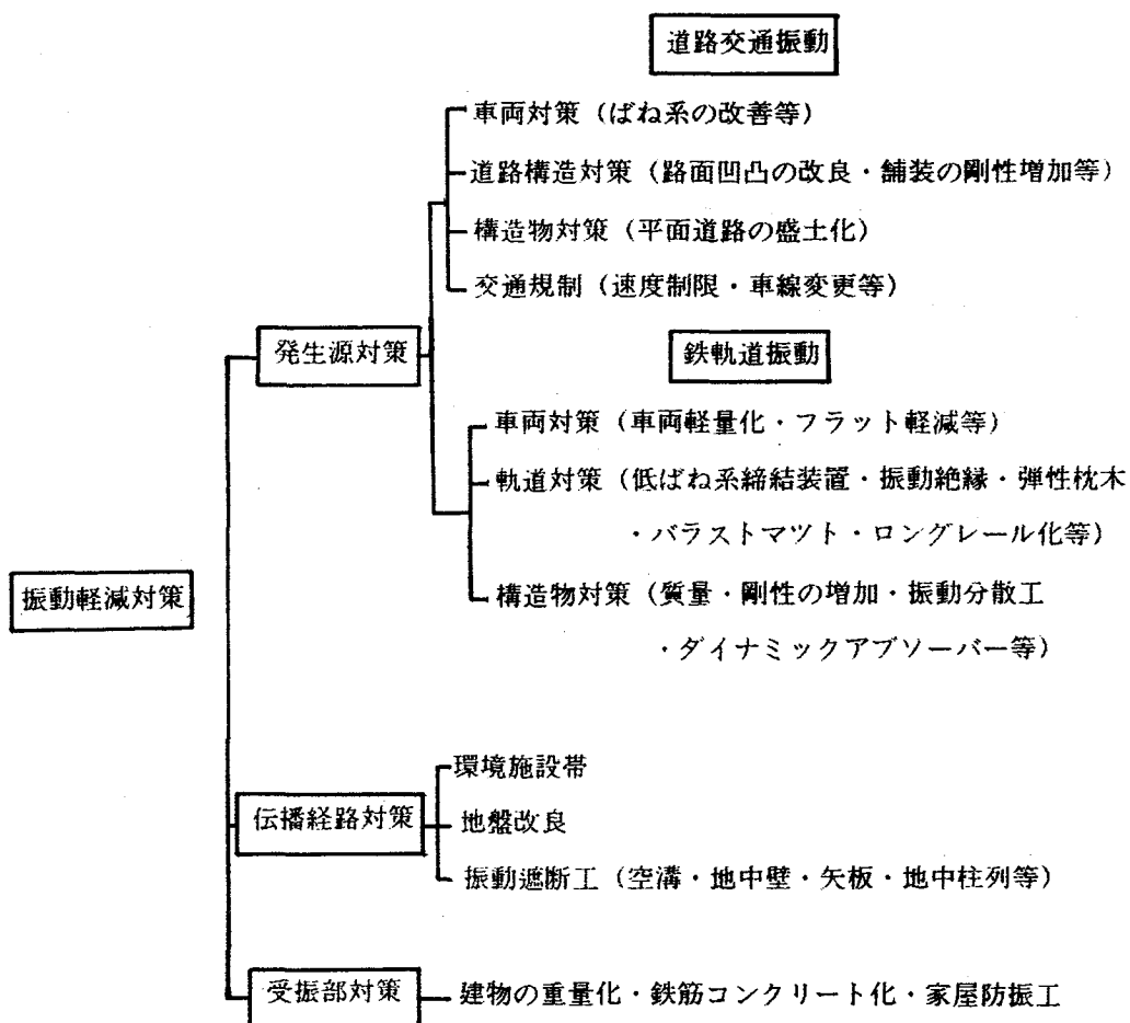
図 3. 2 交通機関による地盤振動の対策法
