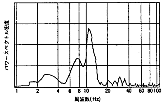
図4. 20 試験車のばね下加速度スペクトル（走行実験Ⅱ）
