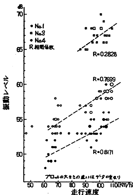
図4. 38 列車速度と振動レベル (2) (ケースⅠ)
