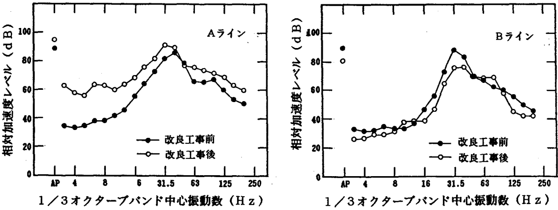
図4.50 地中振動の周波数分析結果
