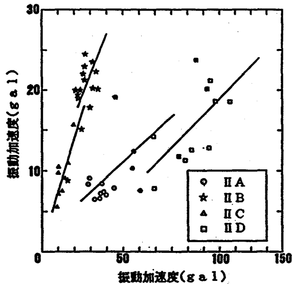
図6. 42 地表と地中の振動加速度の関係（ケースⅡ）
