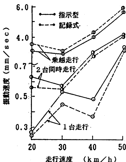
図4. 22 振動速度と走行速度の関係 (走行実験Ⅰ)
