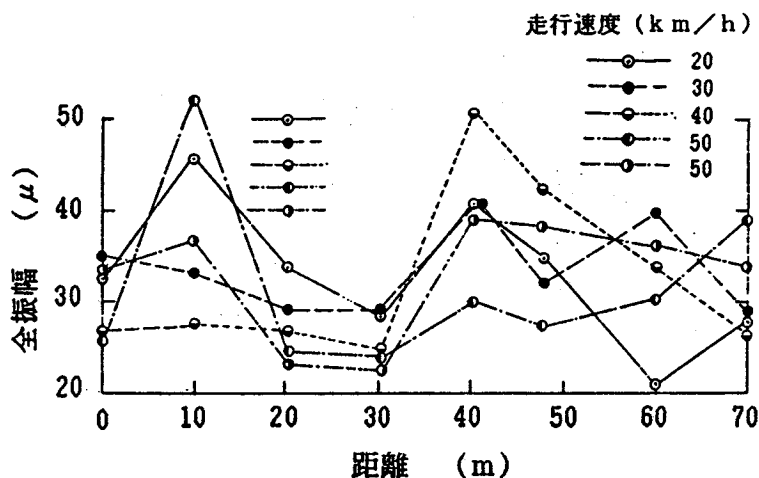
図4. 23 走行路線方向の振動程度の変化 (走行実験Ⅰ)
