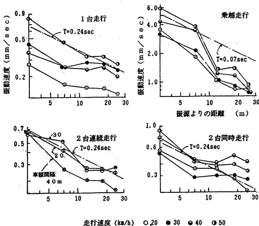
図4. 16 振動速度の距離減衰 (走行実験Ⅰ)
