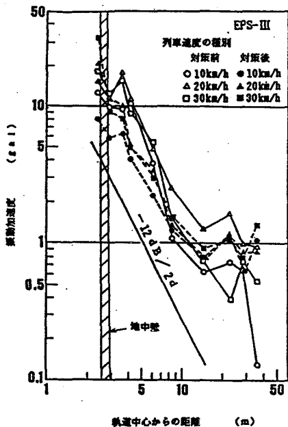
図7.69 振動加速度の距離減衰
