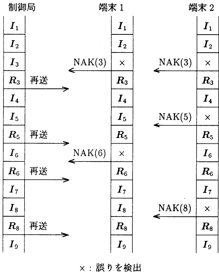
図 3.1 : 一対二同報通信に一対一通信用誤り制御方式を適用した例
