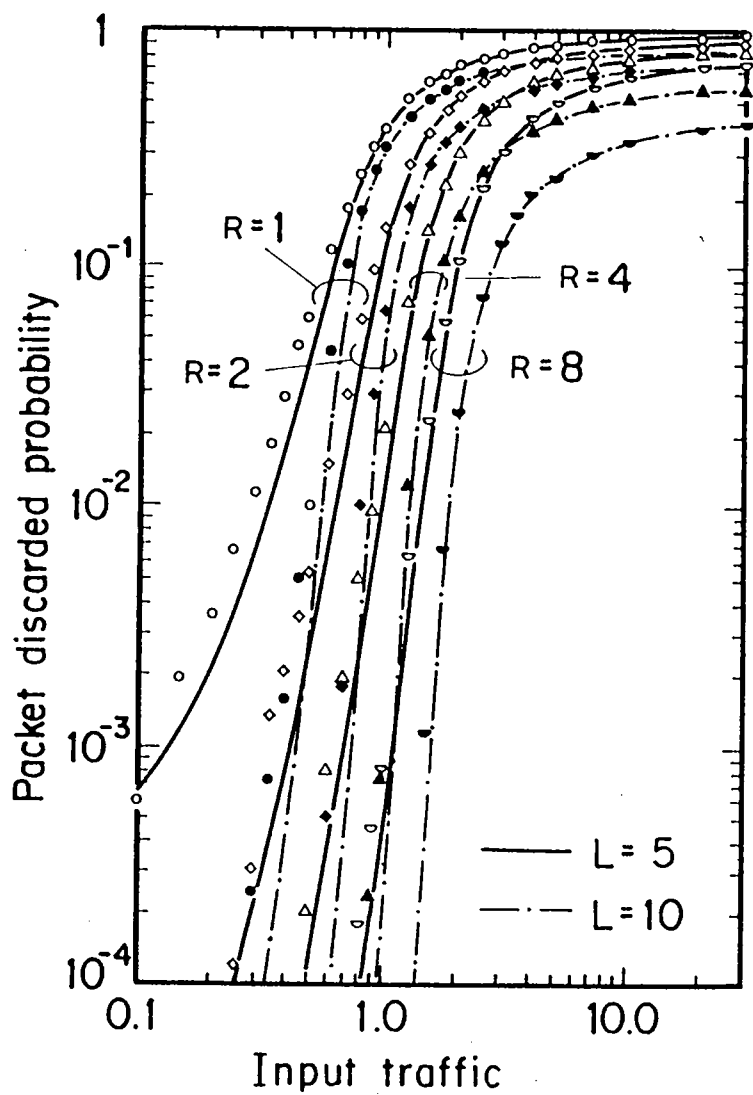
図 5.4 : パケット廃棄確率 ( M = 50 , r_\ell = 0.1 , z_0 = 3(\text{dB}) , \gamma = 10(\text{dB}) )
