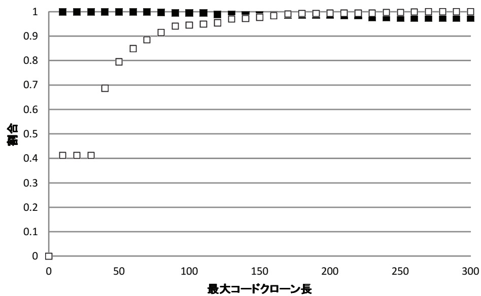
図 4.8: ソースコード再利用なしの場合でのコードクローン検出数と適合率，再現率の関係
