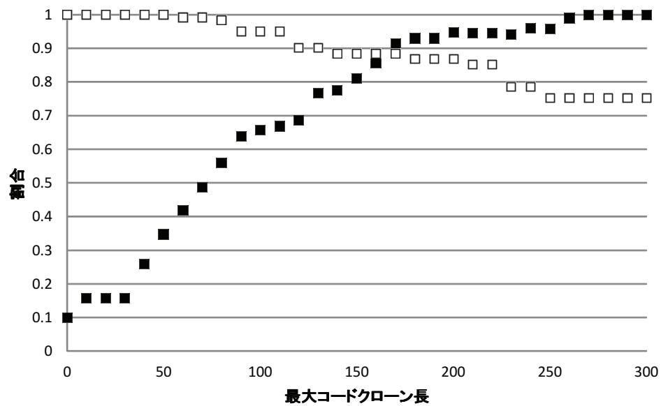
図 4.5: ソースコード再利用ありの場合でのコードクローン検出数と適合率，再現率の関係
