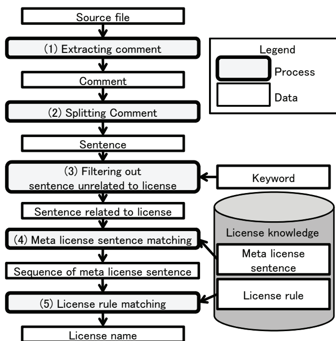
図 1.4: ライセンス特定ツール Ninka の構成
