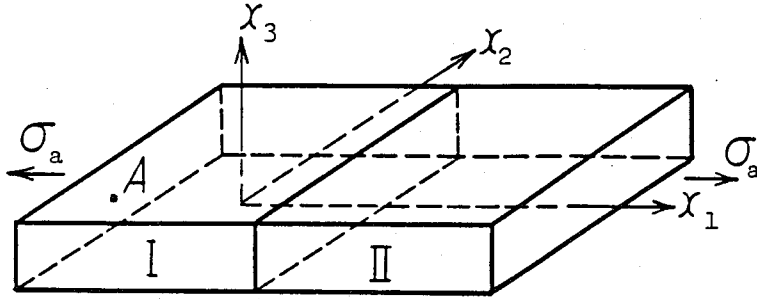
図2-9 粒界面が引張り軸に垂直な板状双結晶試料
