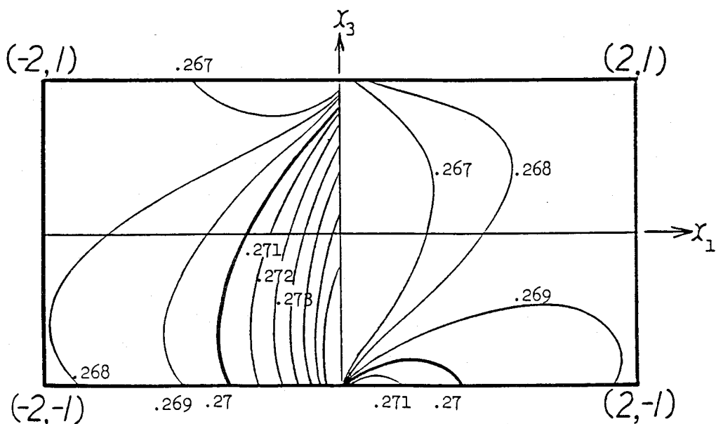
図6-6 (c) 分解せん断応力 (Case 1 \theta = \pi/4 すべり系 a_3 , 単位はPa)
