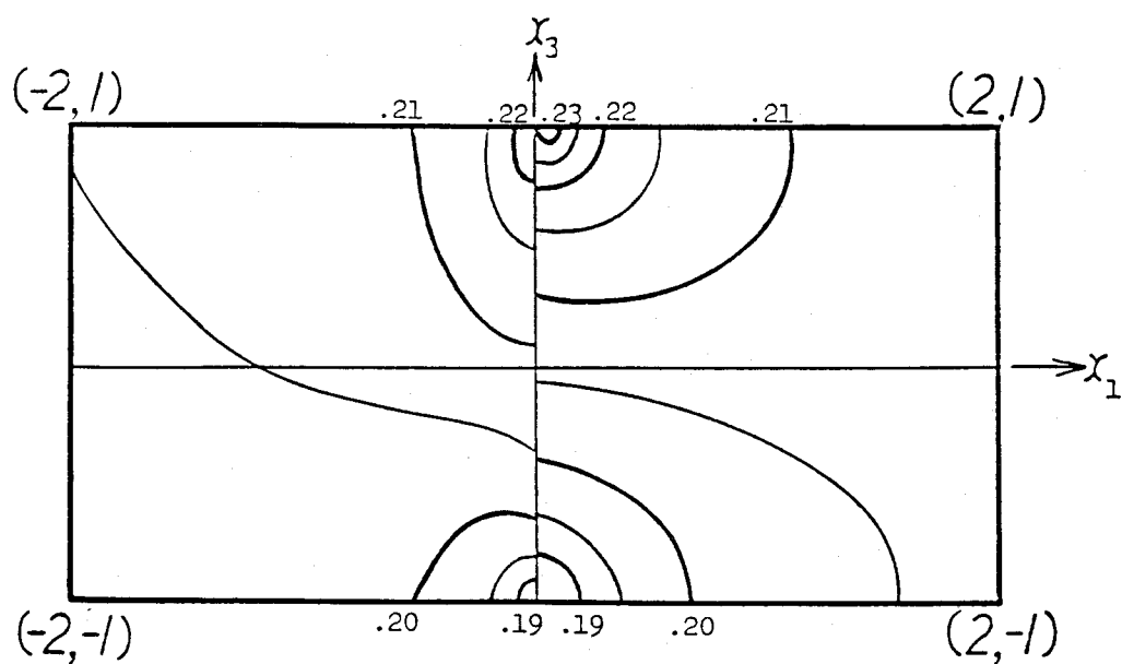
図6-7 (b) 分解せん断応力 (Case 2 \theta = \pi/3 すべり系 a_2 , 単位はPa)
