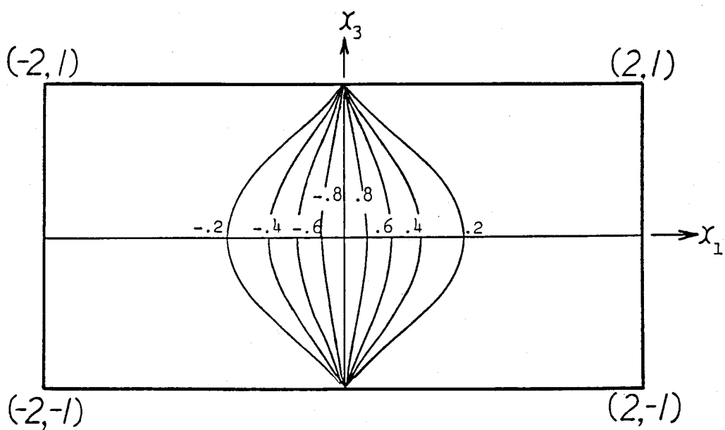
図5-13 不適合応力場 (等応力線 \sigma_{33} , 単位は \rho v )
