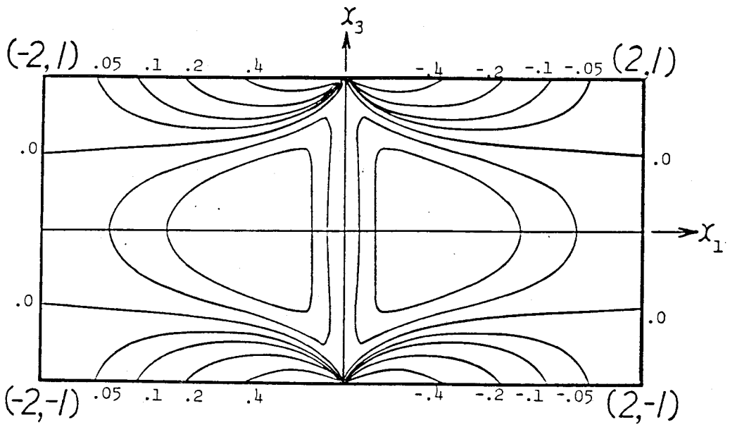
図5-5 単位仮想表面力による応力場 (等応力線 \sigma_{11} , 単位は \rho_0 )
