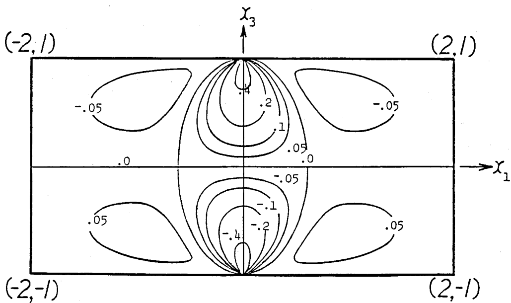
図5-10 単位仮想表面力による応力場 (等応力線 \sigma_{12} , 単位は \rho_0 )
