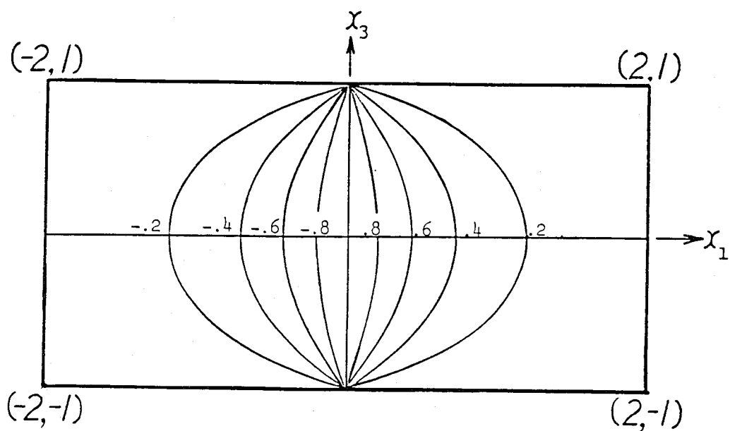
図5-14 不適合応力場 (等応力線 \sigma_{23} , 単位は \rho_0 )
