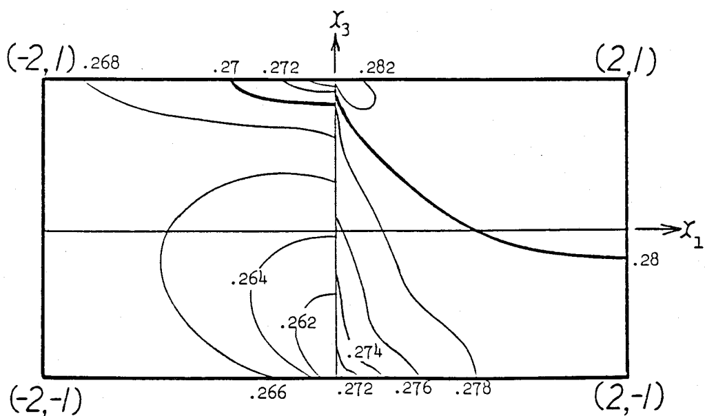
図6-6 (f) 分解せん断応力 (Case 1 \theta = \pi/4 すべり系 b_3 , 単位はPa)
