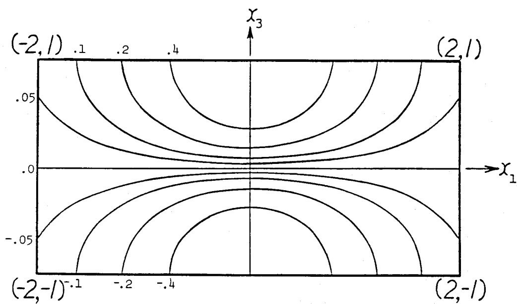
図5-15 不適合応力場 (等応力線 \sigma_{31} , 単位は \rho_0 )
