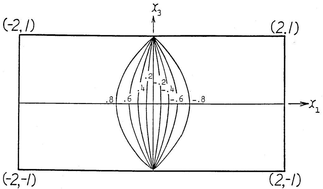
図5-6 単位仮想表面力による応力場 (等応力線 \sigma_{22} , 単位は \rho_0 )
