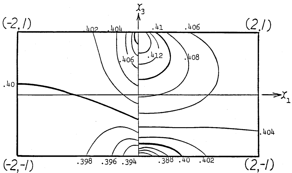
図6-7 (h) 分解せん断応力 (Case 2 \theta = \pi/3 すべり系 c_2 , 単位はPa)
