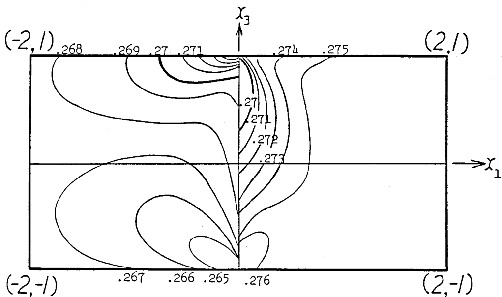
図6-6 (g) 分解せん断応力 (Case 1 \theta = \pi/4 すべり系 c_1 , 単位はPa)
