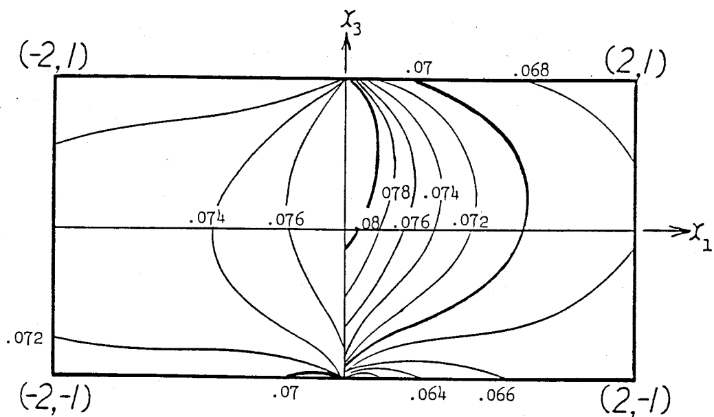
図6-7 (k) 分解せん断応力 (Case 2 \theta = \pi/3 すべり系 d_2 , 単位はPa)
