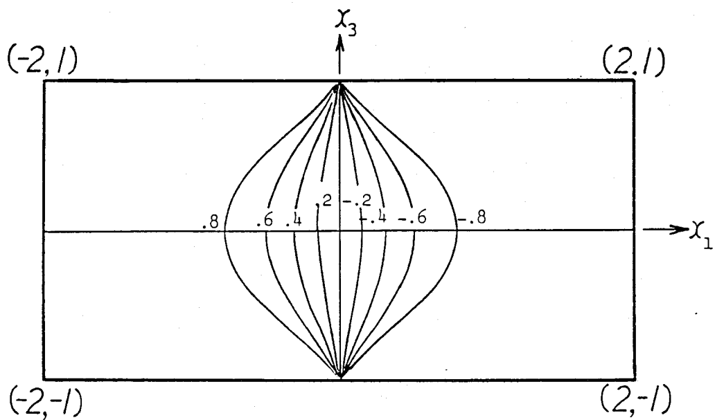
図5-7 単位仮想表面力による応力場 (等応力線 \sigma_{33} , 単位は \rho_0 )
