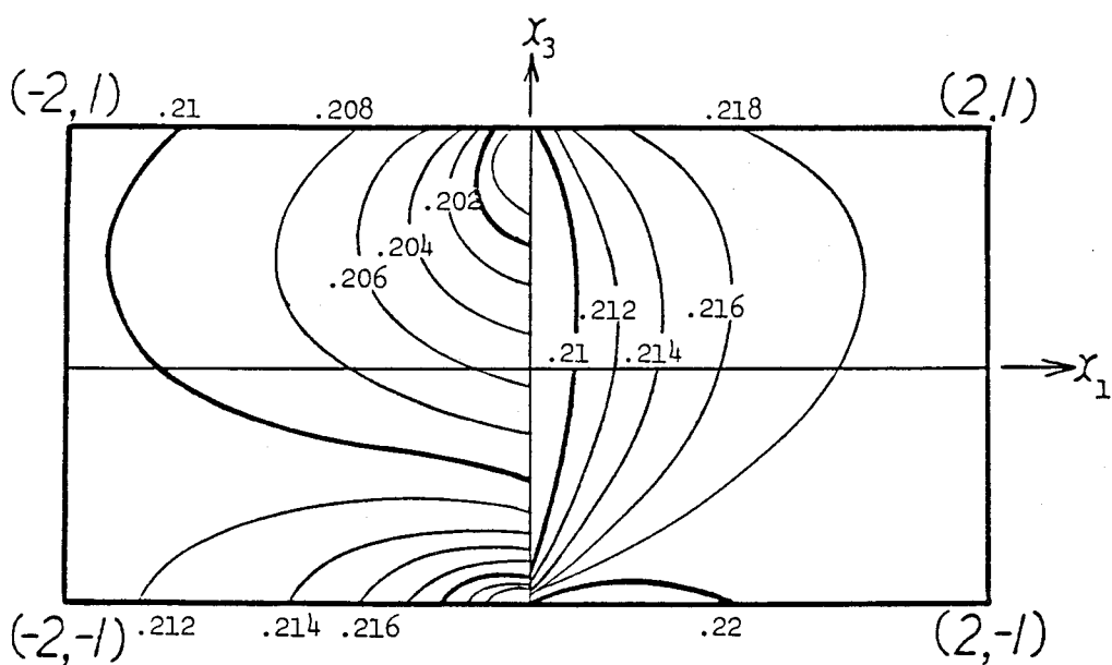
図6-7 (l) 分解せん断応力 (Case 2 \theta = \pi/3 すべり系 d_3 , 単位はPa)
