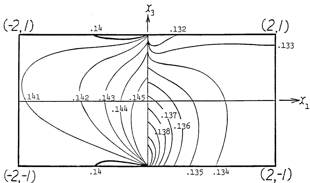
図6-6 (e) 分解せん断応力 (Case 1 \theta = \pi/4 すべり系 b_2 , 単位はPa)
