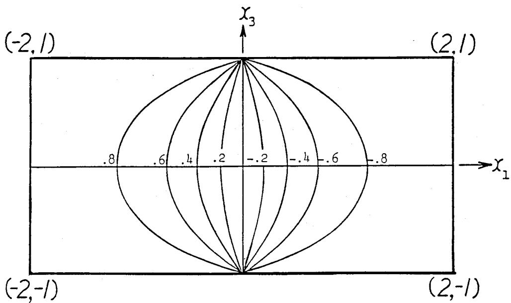
図5-8 単位仮想表面力による応力場 (等応力線 \sigma_{23} , 単位は \rho_0 )
