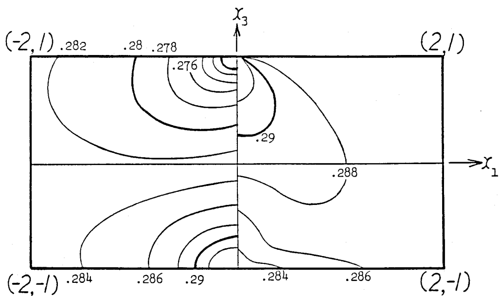
図6-7 (j) 分解せん断応力 (Case 2 \theta = \pi/3 すべり系 d_1 , 単位はPa)
