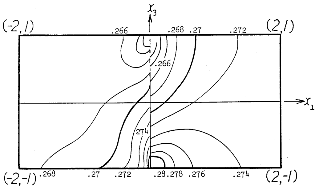
図6-6 (h) 分解せん断応力 (Case 1 \theta = \pi/4 すべり系 c_2 , 単位はPa)
