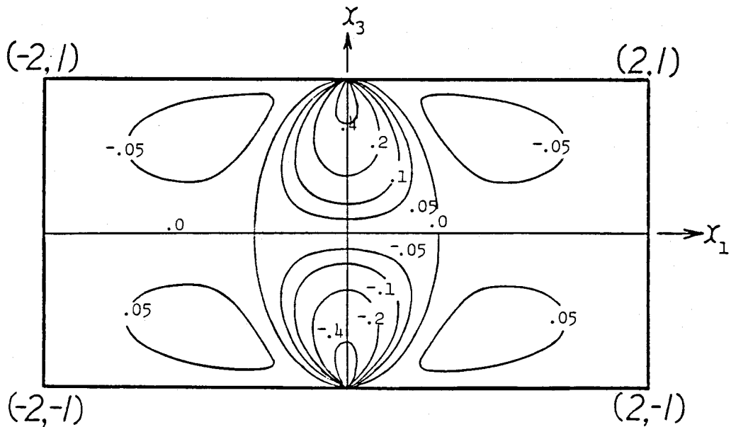
図5-16 不適合応力場 (等応力線 \sigma_{12} , 単位は \rho a )
