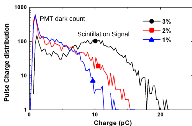
図 10 PrF 3 ドーピング量を変えた時の発光量分布測定。ドーピング量増加に伴い発光量増加がみられる。
