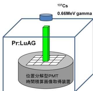
図 54 シンチレータースタックからの発光発散角測定セットアップ
