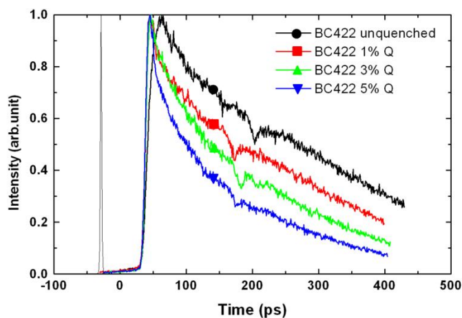
図 12 BC-422 BC-422Q の発光応答ラインプロファイル
