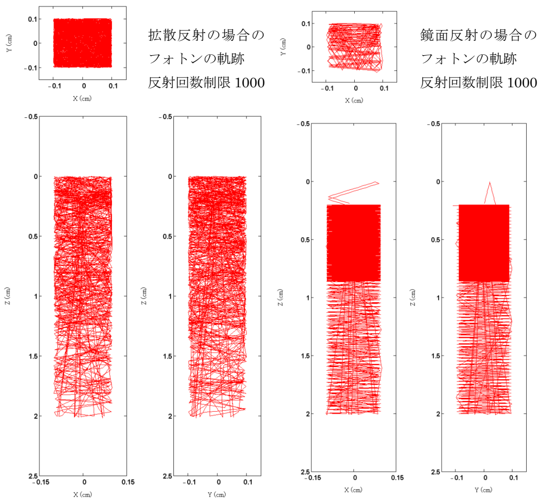
図 52 シミュレーション計算によるフォトン軌跡
