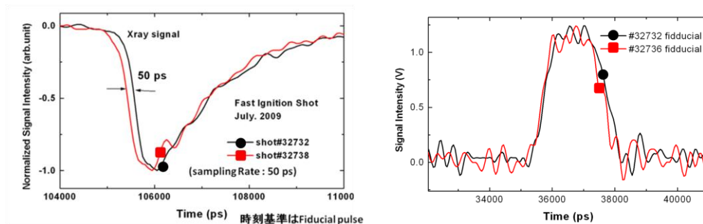
図 32 高速点火ショットにおけるバースタイム測定時間分解能評価。左はシンチレータからの信号、右はタイムフィデューシャルである激光 XII レーザーの散乱光をピックアップしてフォトダイオードで観測したもの。
