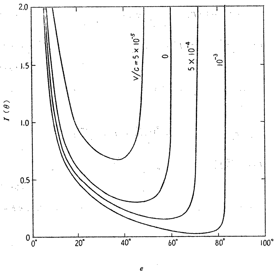
図5・3 角スペクトラム
