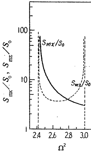
図 2・2 正規化 Poynting ベクトル ( v/u=0 , U=-1 , R^2=2 )
