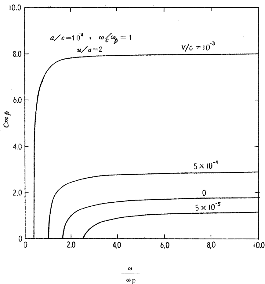
図 5・1 Cerenkov 放射に対する分散式
