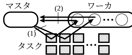
図 2.5: マスタ・ワーカー方式の概念図
