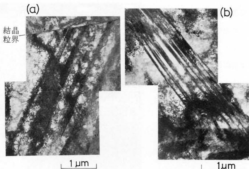
図 4.3.8 -196 °C で 8hr 深冷処理した 40% 加工材の内部組織。 (a) 100 °C 加工, (b) 100 °C 加工 → 深冷.
