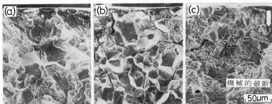
図 2.3.14 負荷応力に対する SCC 破面形態の変化（通気状態の沸騰42% \text{MgCl}_2 溶液）. (a) 10 \text{ kg/mm}^2 , (b) 30 \text{ kg/mm}^2 , (c) 45 \text{ kg/mm}^2 負荷.
