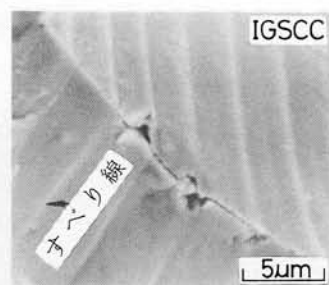
図 2.3.15 粒界型 SCC (IGSCC) 破面上のすべり線模様（脱気状態の沸騰42% \text{MgCl}_2 溶液， 40 \text{ kg/mm}^2 負荷）.
