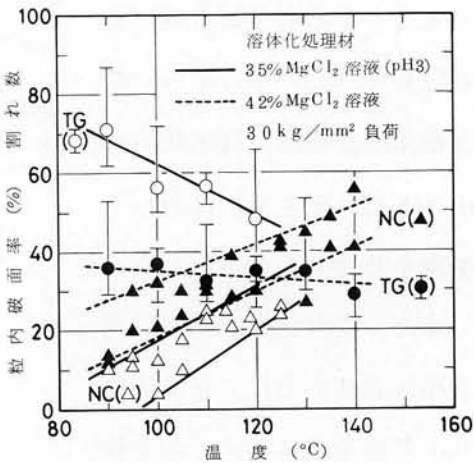
図 2.3.10 粒内破面率 (TG)、割れ数 (NC) と溶液温度との関係。
