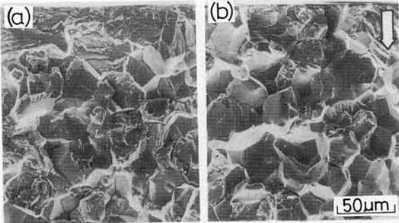
図 2.3.11 100℃, \text{MgCl}_2 溶液中における SCC 破面形態, (a) 35% (pH3), (b) 42% \text{MgCl}_2 .
