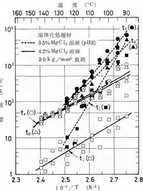
図 2.3.9 \text{MgCl}_2 溶液中における破断時間 ( t_f )、割れ発生期間 ( t_i )、割れ伝播期間 ( t_p ) と溶液温度との関係 (アレニウス・プロット)。
