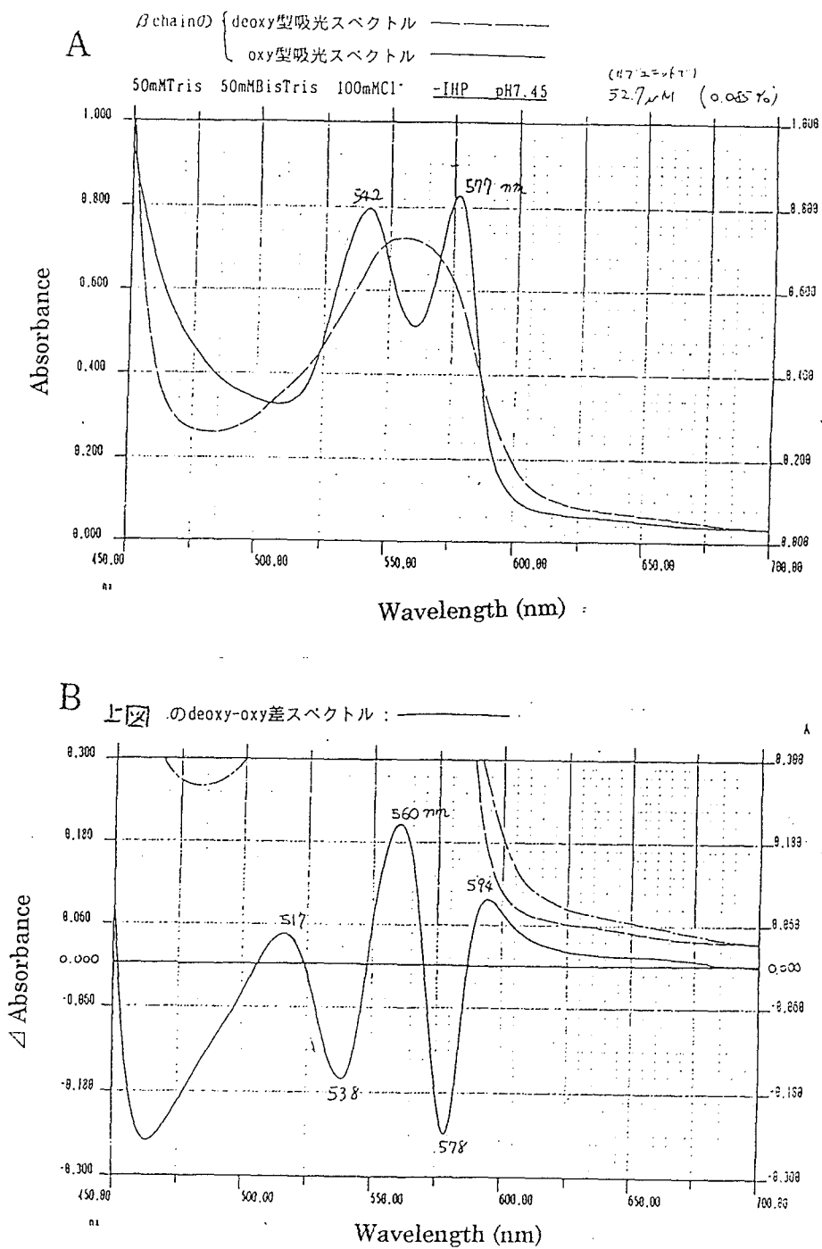
図 2-4 \beta (Fe)サブユニット、 \alpha_2(\text{Cr})\beta_2(\text{Fe}) の吸光スペクトルの吸光スペクトル
