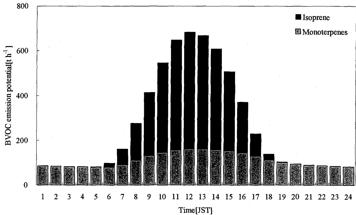
図 5-8 8月における BVOC 発生量の日変動
