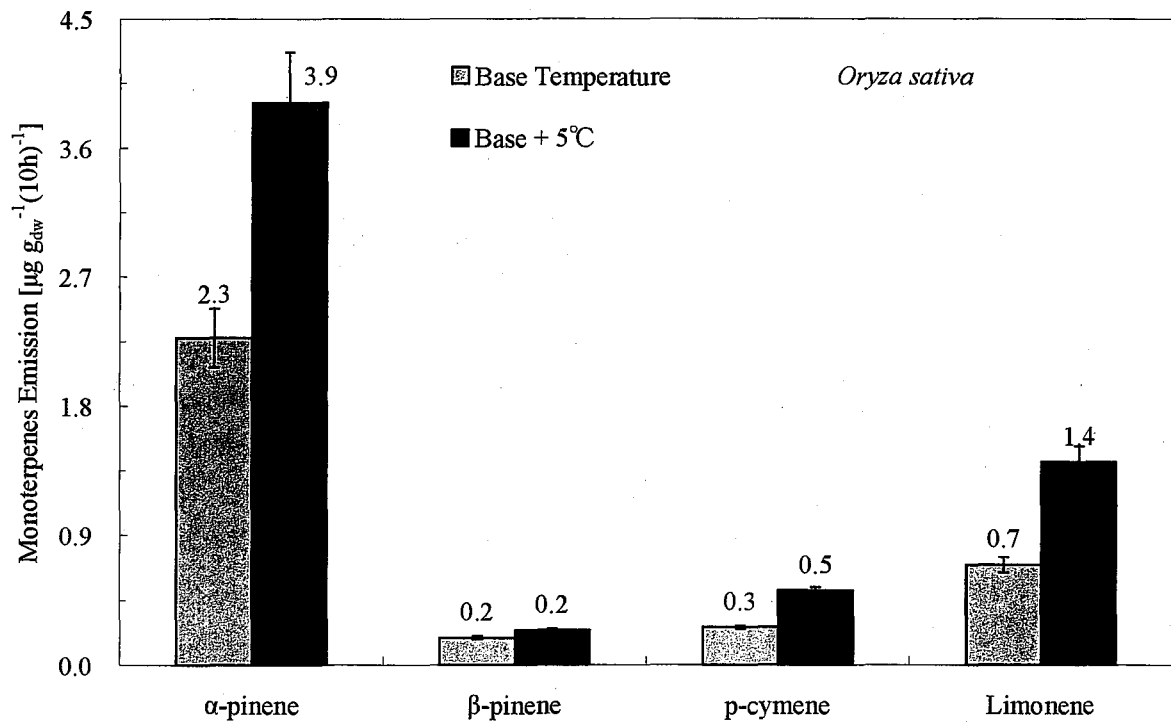
図 3-26 イネから発生するモノテルペン類の日積算発生量の葉温依存性の比較
