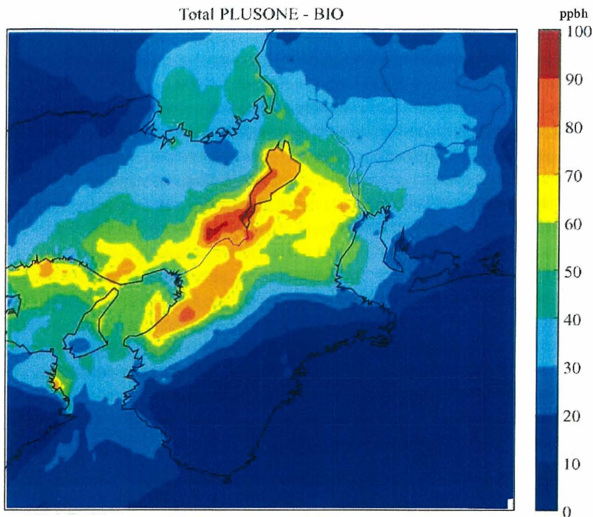
図 6-17 葉温 1℃上昇に伴う BVOC 発生量の影響による月積算 オゾン AOT40 の増加(ppbh)分布
