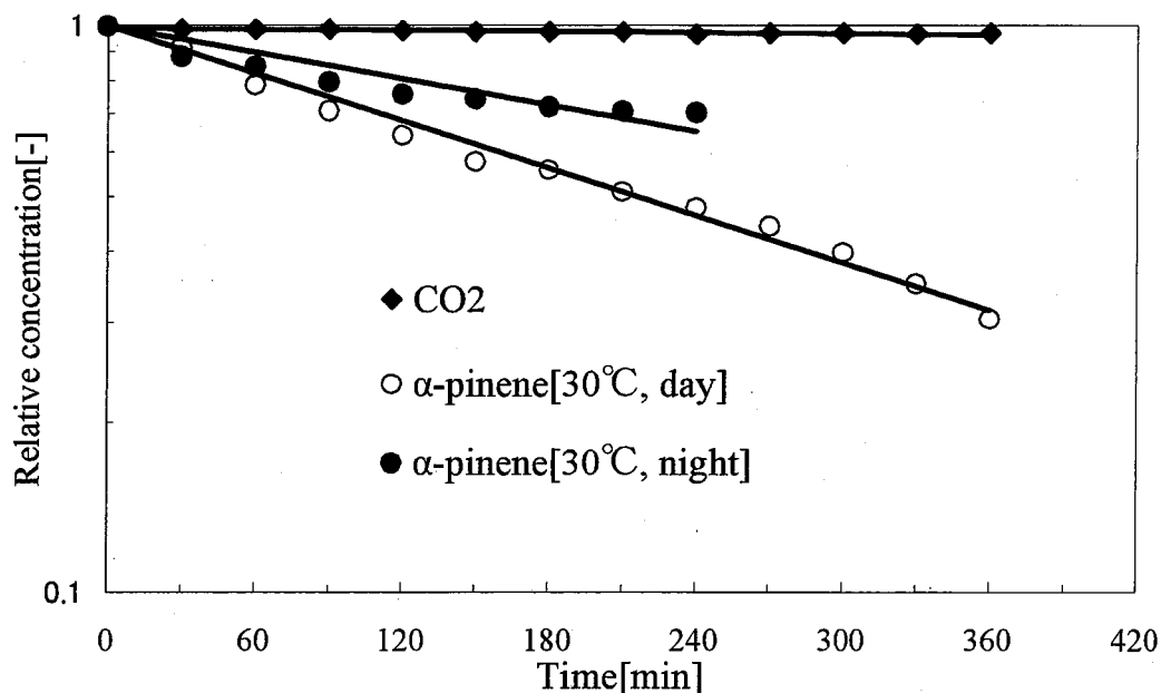
図3-8 チャンバー内気温 30 \pm 1^\circ\text{C} , PAR 0, 335 \mu\text{mol m}^{-2} \text{s}^{-1} α-ピネン初期濃度1.14ppb, 及び \text{CO}_2 初期濃度6000ppmでの相対濃度の時間変化
