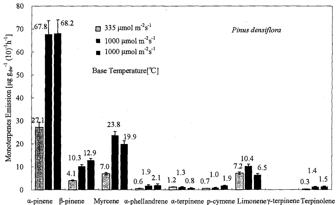
図 3-35 ベース気温におけるアカマツから発生するモノテルペン類の日積算量の比較
