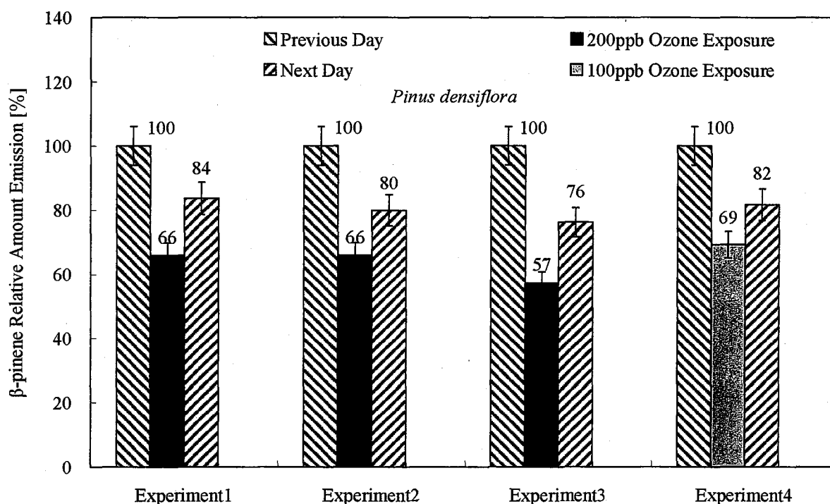
図 4-9 オゾン暴露前日の \beta -ピネン発生量を基準とした アカマツからの \beta -ピネン発生量の相対値
