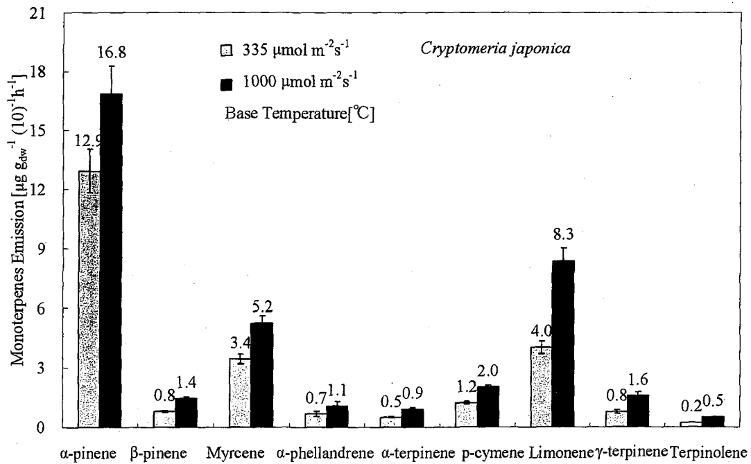
図 3-31 ベース気温におけるスギから発生するモノテルペン類の日積算量の比較
