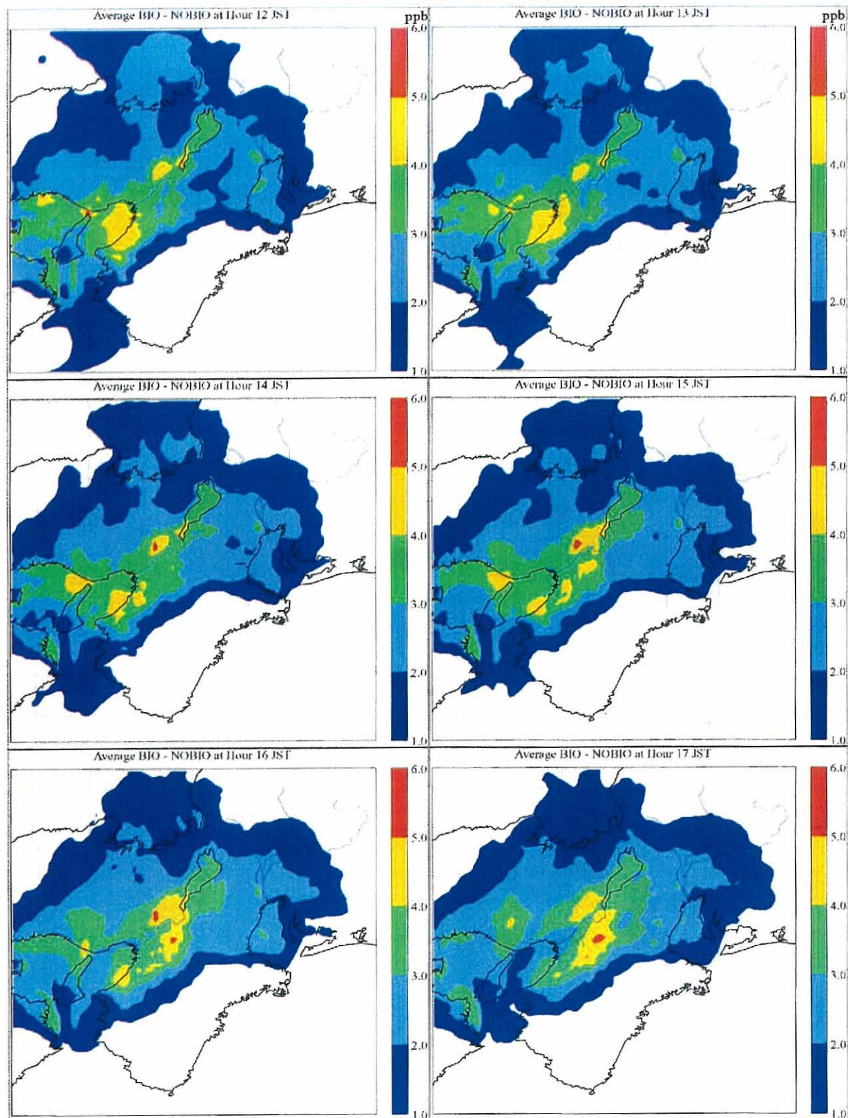
図 6-14 BIO と NOBIO-シミュレーション結果における月平均時間ごとのオゾン濃度の増加分布(2002 年 7 月) (3)
