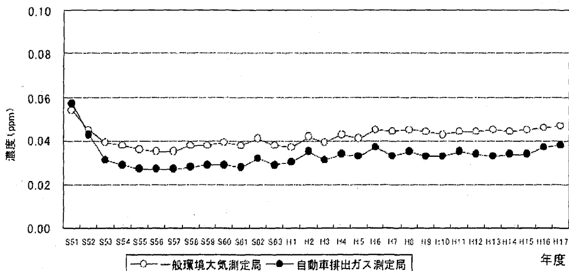
図 1-1 昼間の日最高 1 時間値の年平均値の経年変化
