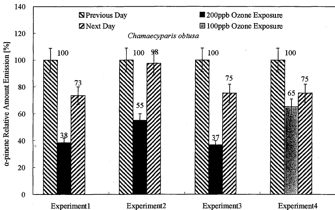
図4-6 オゾン暴露前日の \alpha -ピネン発生量を基準としたヒノキからの \alpha -ピネン発生量の相対値
