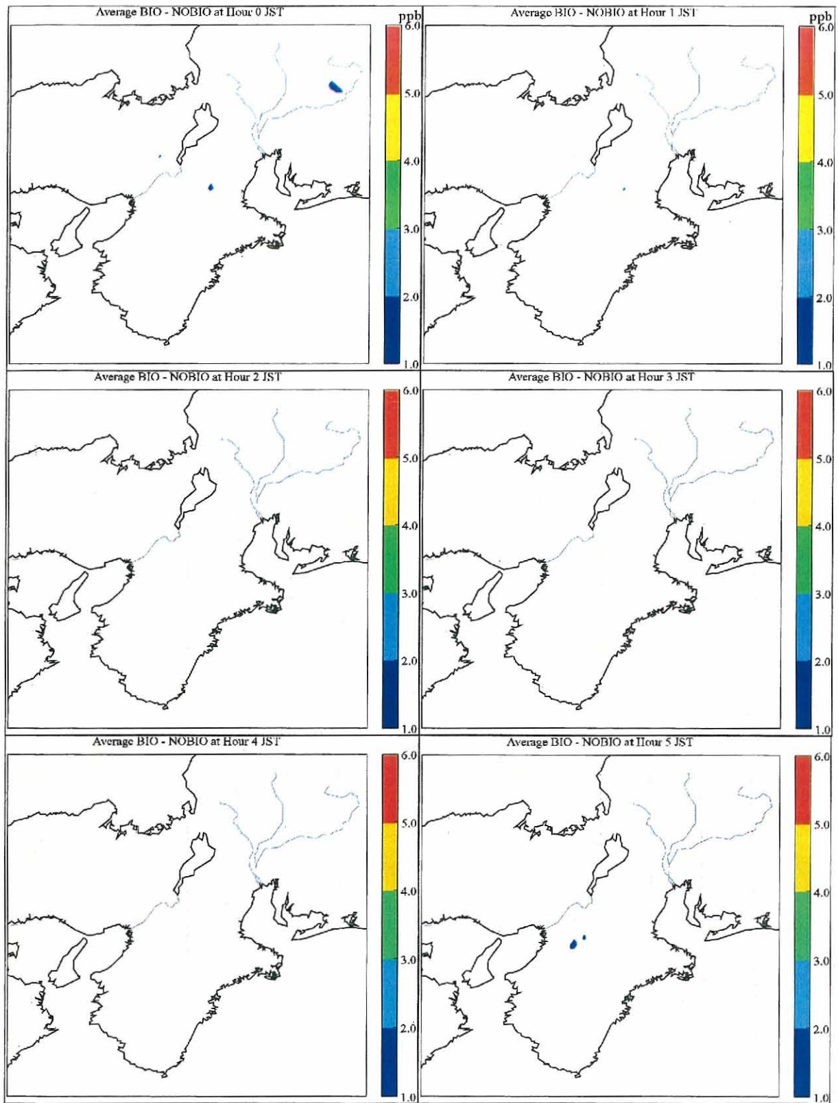
図 6-14 BIO と NOBIO-シミュレーション結果における月平均時間ごとのオゾン濃度の増加分布(2002 年 7 月)(1)
