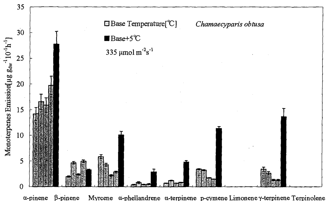
図 3-22 ヒノキから発生するモノテルペン類の日積算発生量の葉温依存性の比較
