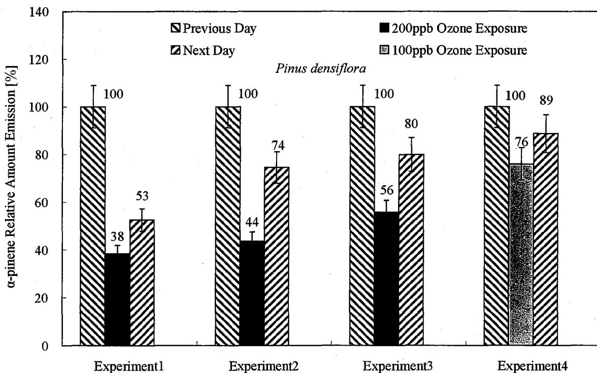
図4-8 オゾン暴露前日の \alpha -ピネン発生量を基準としたアカマツからの \alpha -ピネン発生量の相対値
