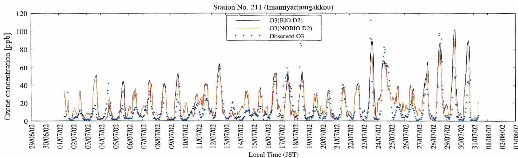
図 6-11 観測地点今宮中学校における NOBIO-シミュレーション結果と BIO-シミュレーション結果の観測値との比較 (2002 年 7 月)
