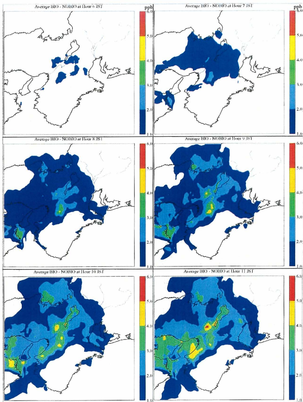
図 6-14 BIO と NOBIO-シミュレーション結果における月平均時間ごとのオゾン濃度の増加分布(2002 年 7 月) (2)
