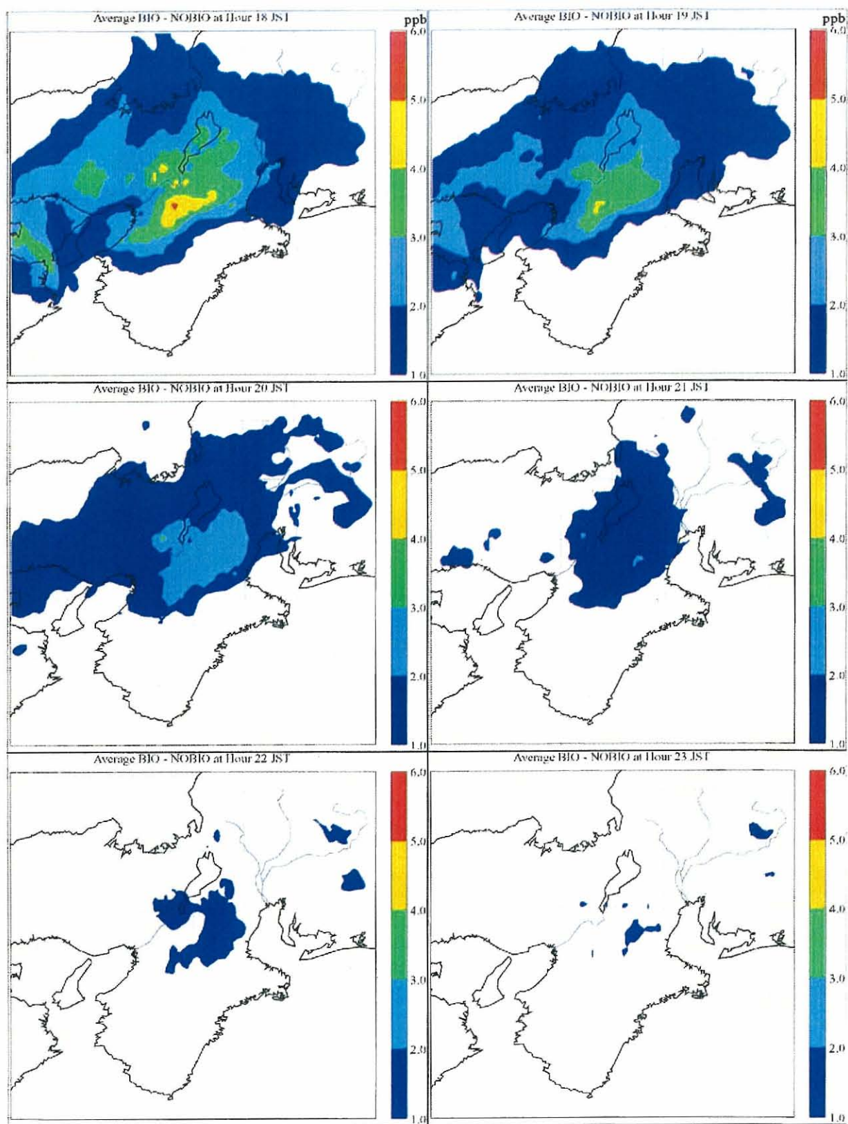
図 6-14 BIO と NOBIO-シミュレーション結果における月平均時間ごとのオゾン濃度の増加分布(2002 年 7 月) (4)
