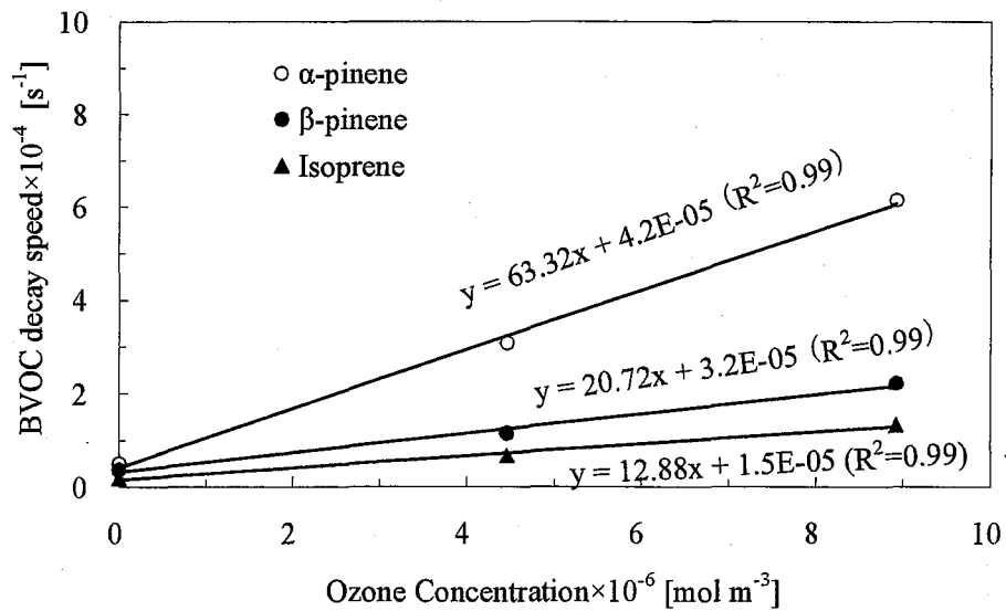
図 4-3 チャンバー内気温 30\pm1^{\circ}\text{C} , オゾン濃度 0, 100, 200ppb における BVOC の減衰速度
