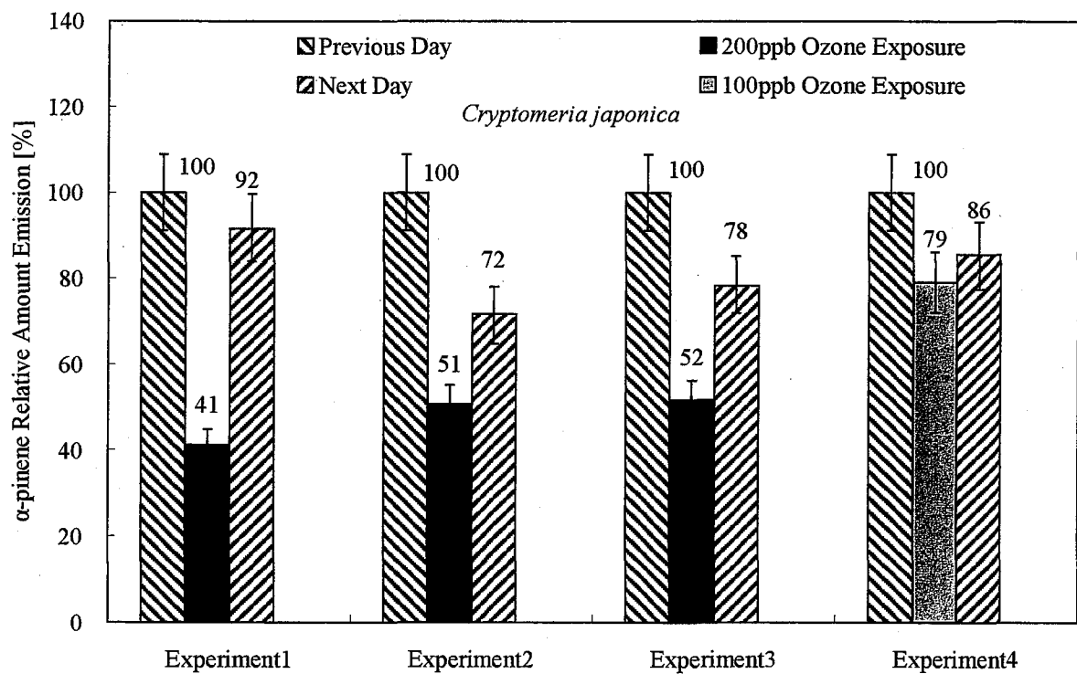
図4-4 オゾン暴露前日の \alpha -ピネン発生量を基準としたスギからの \alpha -ピネン発生量の相対値
