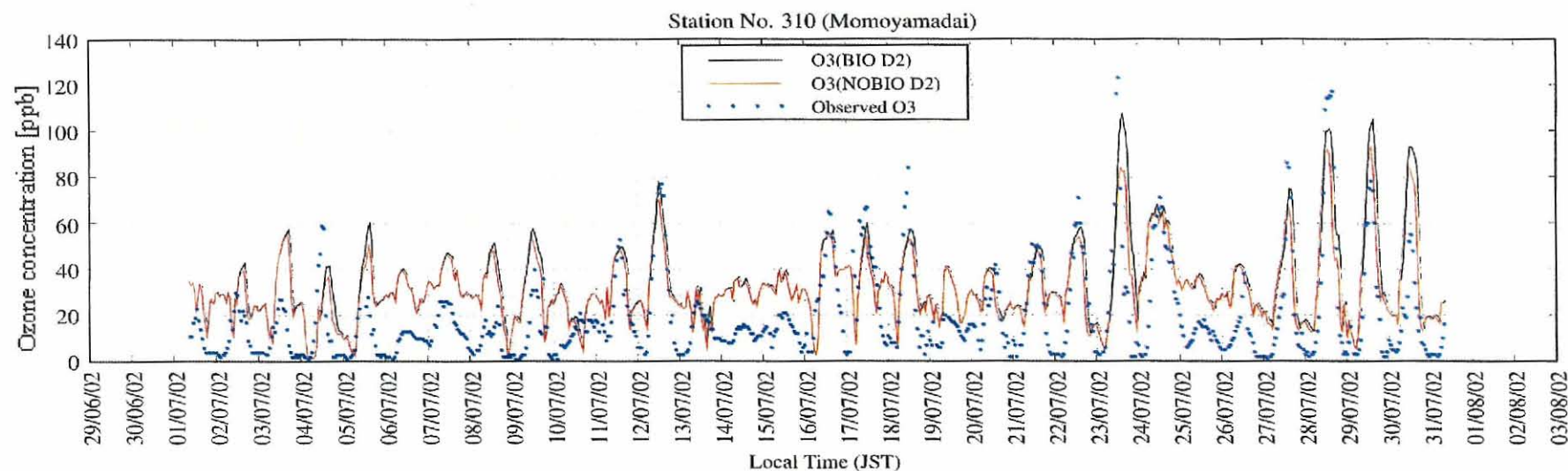
図 6-10 観測地点桃山台における NOBIO-シミュレーション結果と BIO-シミュレーション結果の観測値との比較(2002 年 7 月)
