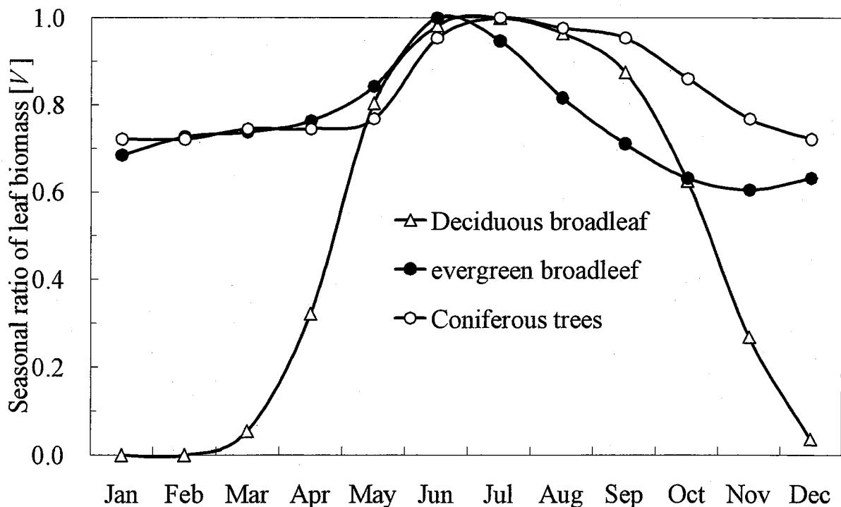
図5-10 樹木の葉の量の季節変化
