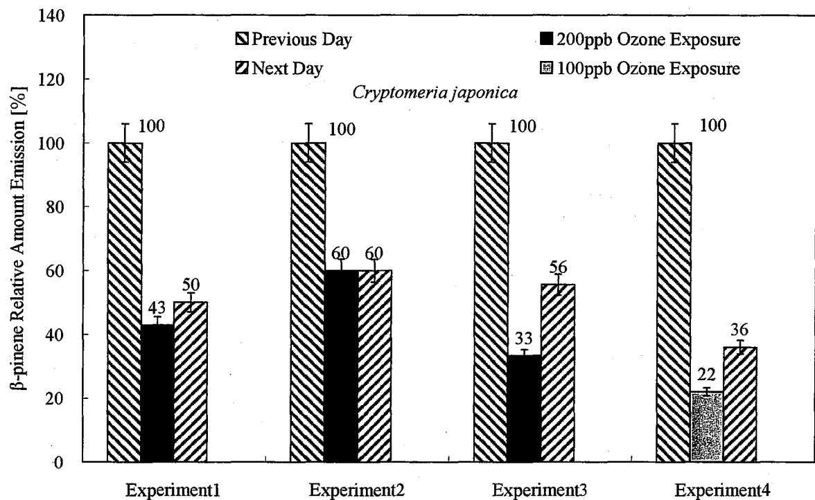
図4-5 オゾン暴露前日の \beta -ピネン発生量を基準としたスギからの \beta -ピネン発生量の相対値
