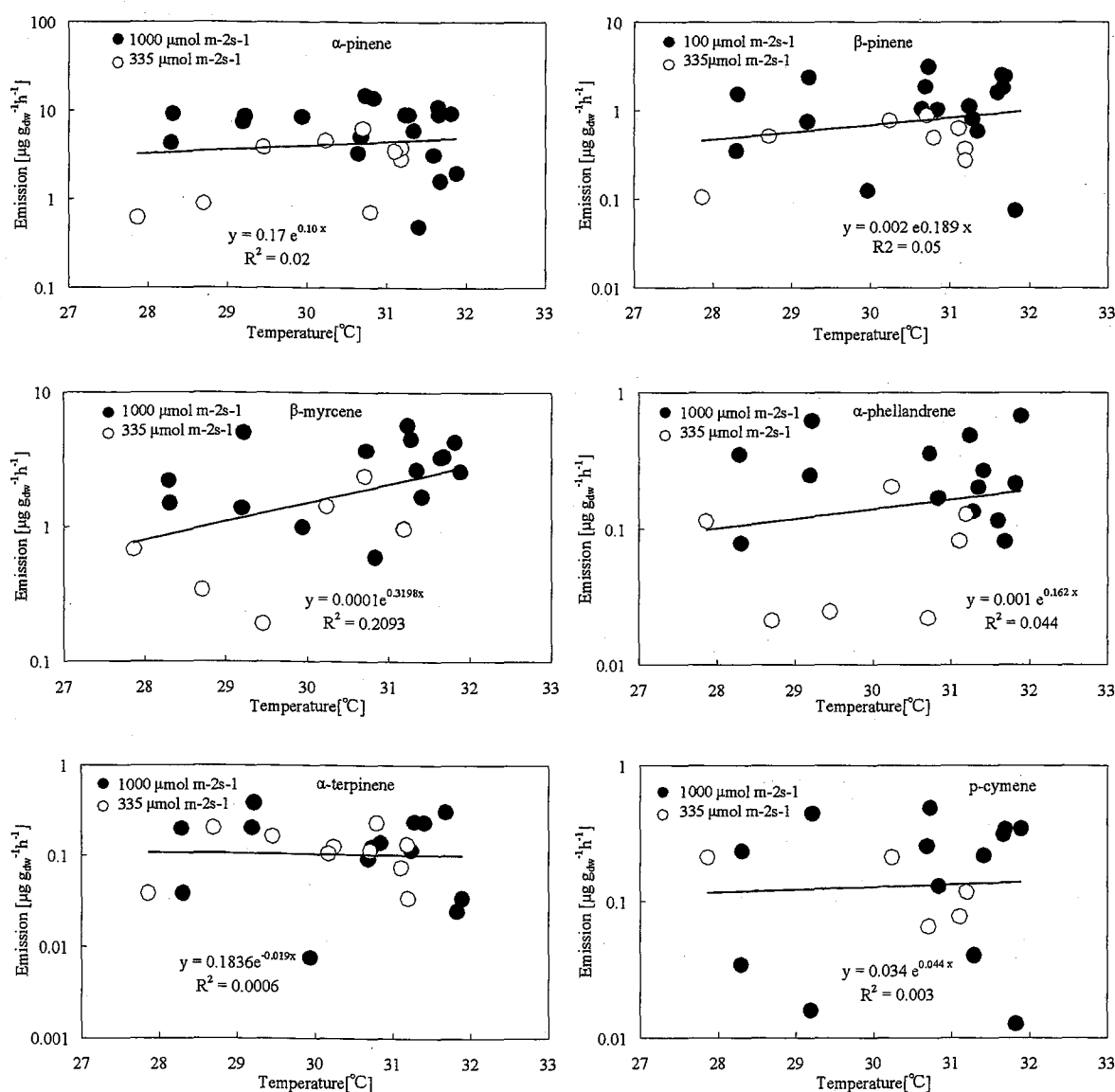
図 3-34 ベース気温におけるアカマツから発生するモノテルペン類の 光量及び葉温依存性
