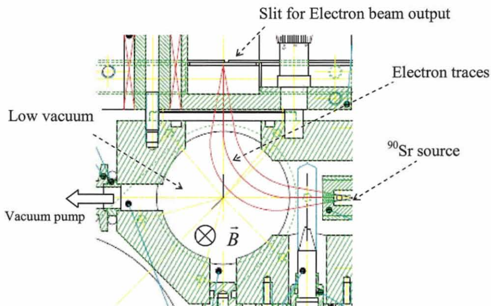
Fig. 2.2.1 Schematic view of the electron spectrometer at CENBG (Le Centre d'Études Nucléaires de Bordeaux Gradignan), France [18]
