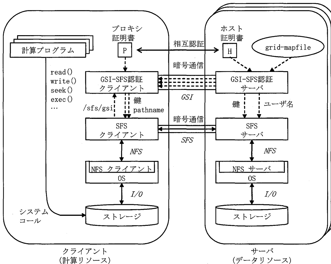
図 3.1 GSI-SFS のアーキテクチャ。
