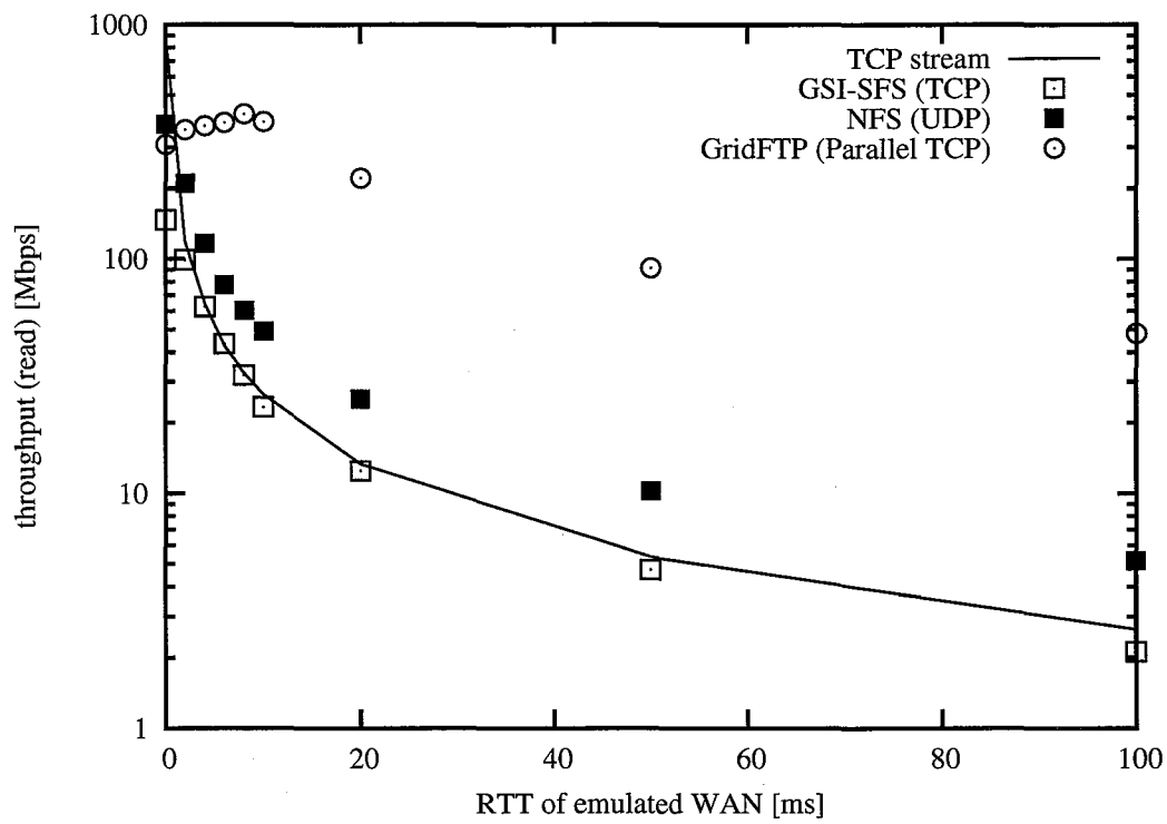
図 3.6 遅延の大きい環境での RTT と読み込みスループット.
