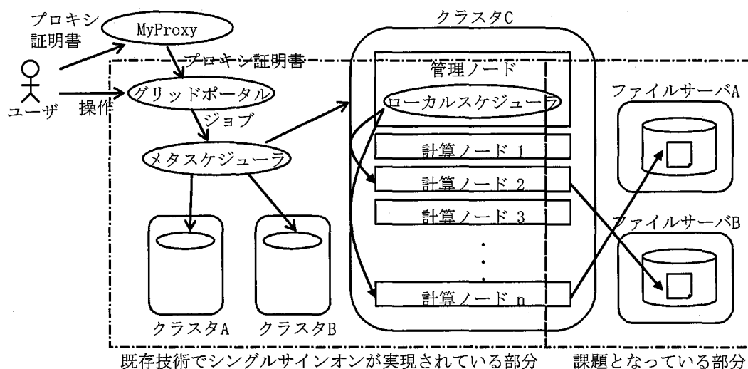
図 2.12 シングルサインオンの科学技術計算に向けての課題。
