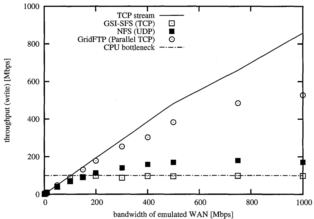
図 3.5 遅延の小さい環境での帯域と書き込みスループット.
