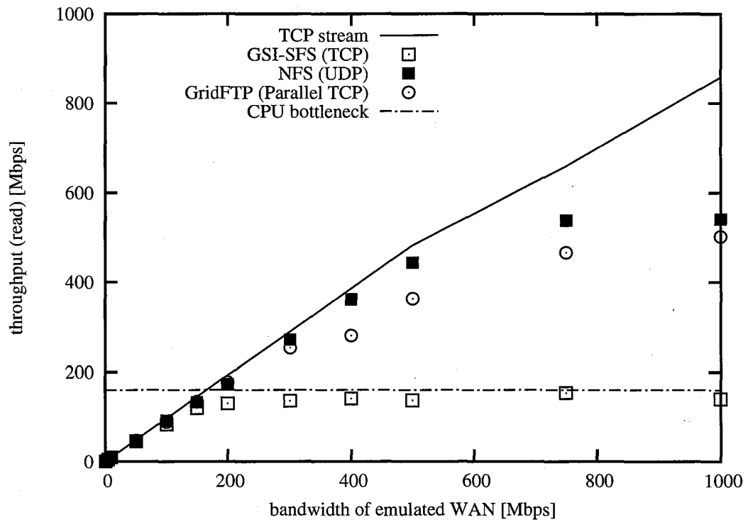
図 3.4 遅延の小さい環境での帯域と読み込みスループット.
