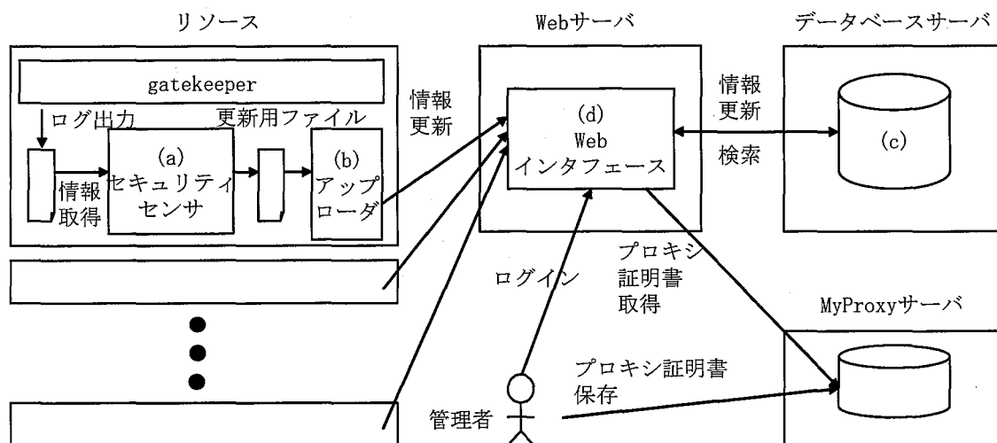
図 4.3 提案するセキュリティモニタリングシステムの構成。
