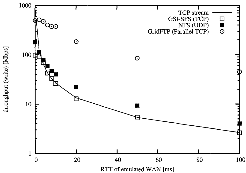
図 3.7 遅延の大きい環境での RTT と書き込みスループット.
