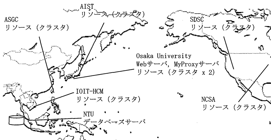
図 4.13 評価実験を行ったテストベッド構成.
