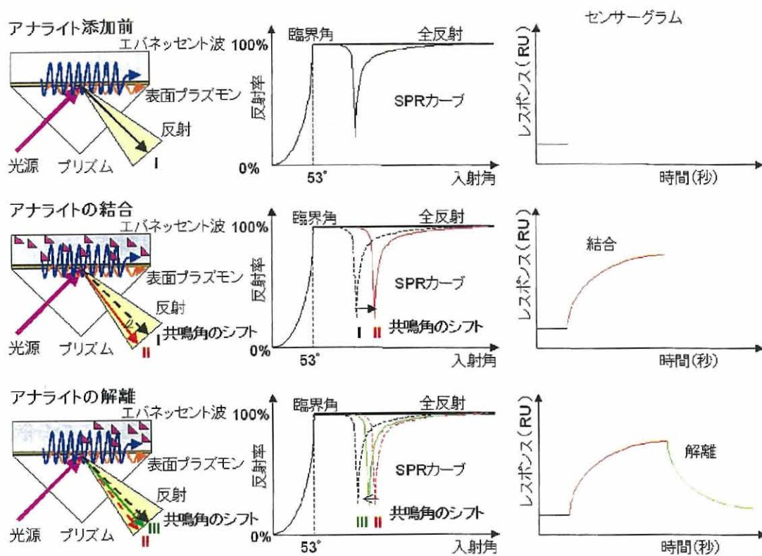
図 1-13 アナライต์の結合および解離に伴う共鳴角のシフトとそのセンサグラム
