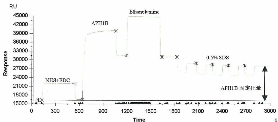
図 6-3 APH1B 固定化センサーグラム
