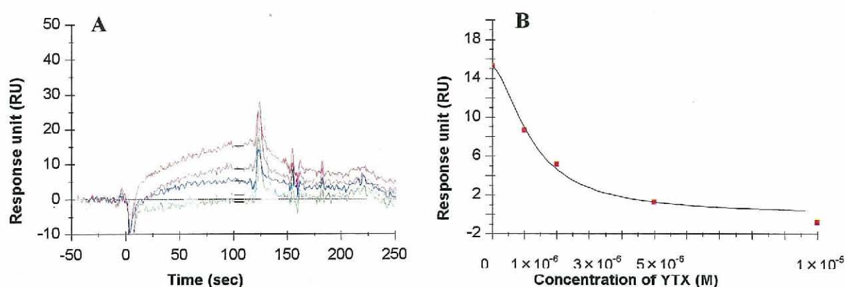
図 4-22 (A) 阻害測定法による YTX (0～10 \mu M) と 1 nM PDE4D を含んだ試料のセンサーグラム（グレー，ベースライン；赤，0；マゼンタ；1，青；2，水色；5 および緑，10 \mu M YTX）と (B) YTX の濃度（横軸）と平衡時（添加 100～110 秒後）の RU 値（縦軸）のプロットと阻害曲線
