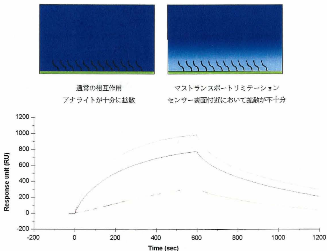
図 2-14 マスポートリミテーション (上: 濃淡はアナライトの濃度を示す) とマスポートリミテーションが生じたセンサーグラム (下: 黄, 1 \mu M; 茶, 5 \mu M およびマゼンタ, 20 \mu M AmB と 20%エルゴステロール含有 POPC 脂質二重膜とのセンサーグラム)
