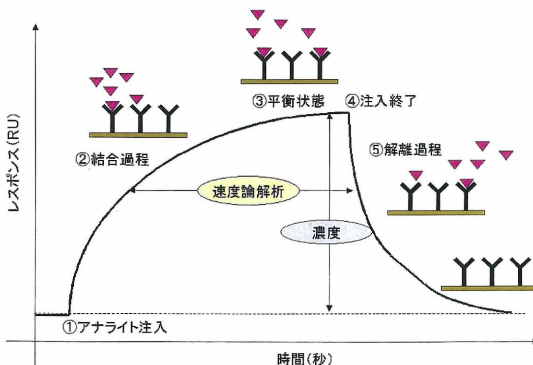
図 1-6 一般的な SPR センサーグラム
