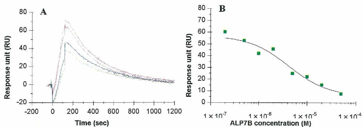
図 4-34 (A)阻害測定法による ALP7B と 5 \mu g/mL PDEII を含んだ試料のセンサーグラム (赤, 0 ; マゼンタ, 0.5 ; 青, 2 および 緑, 20 \mu M ALP7B) と (B) ALP7B の濃度 (横軸) と平衡時 (添加 100~110 秒後) の RU 値 (縦軸) のプロットと阻害曲線
