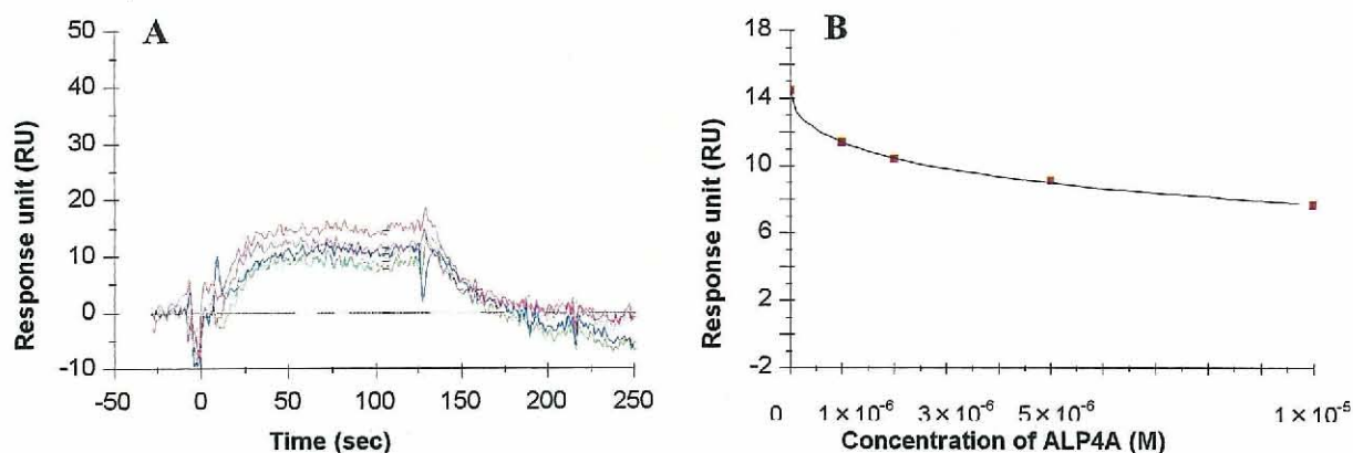
図 4-27 (A) 阻害測定法による ALP4A (0~10 \mu\text{M} ) と 1 nM PDE4D を含んだ試料のセンサーグラム (グレー, ベースライン; 赤, 0; マゼンタ; 1, 青; 2, 水色; 5 および緑, 10 \mu\text{M} ALP4A) と (B) ALP4A の濃度 (横軸) と平衡時 (添加 100~110 秒後) の RU 値 (縦軸) のプロットと阻害曲線
