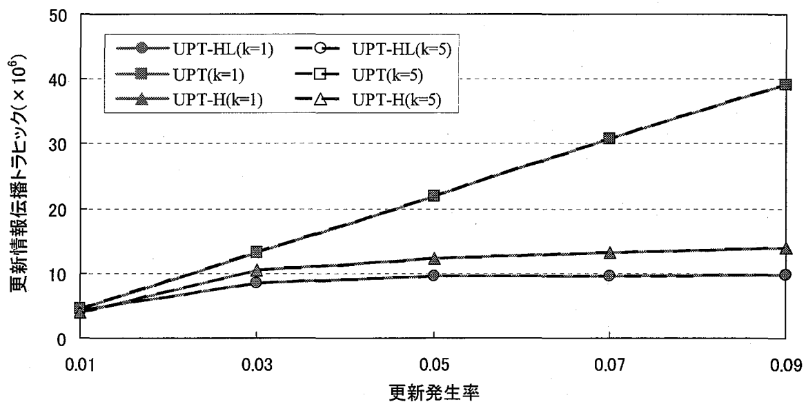
図 3.6: 更新情報伝播トラヒック
