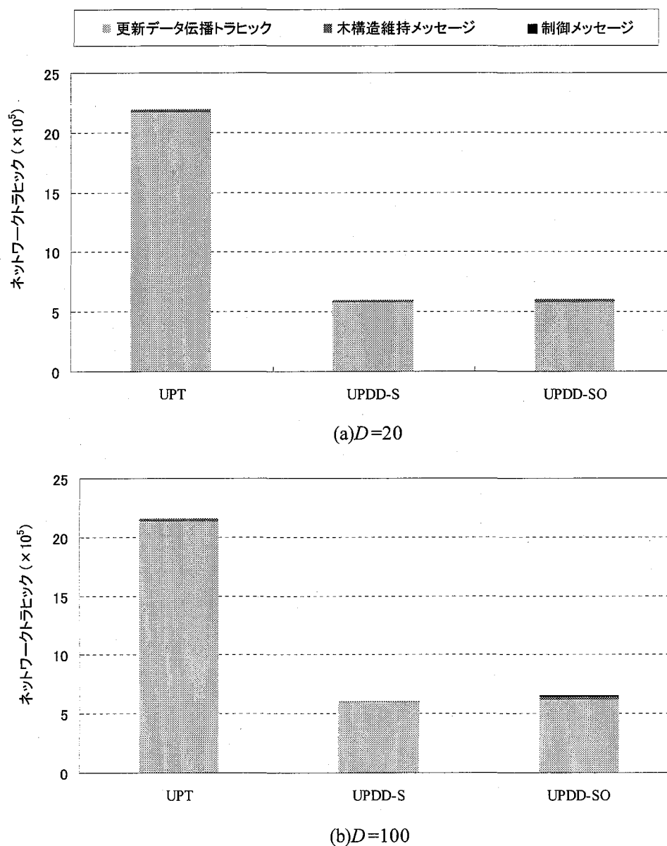
図 4.10: ネットワークトラフィック
