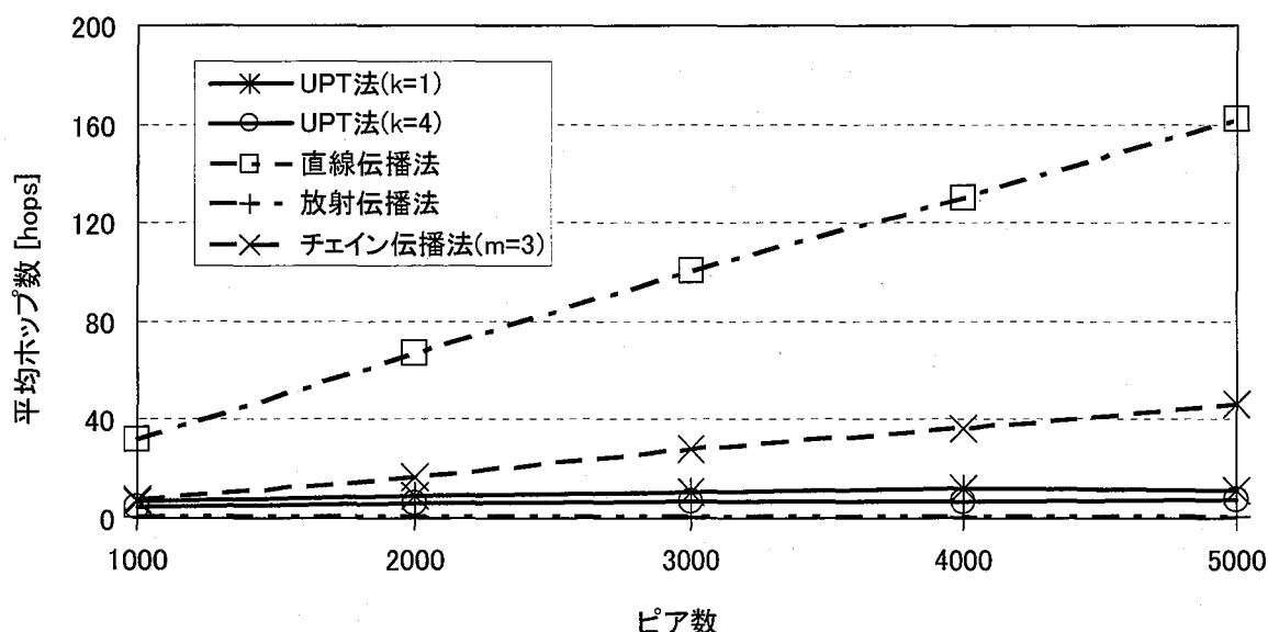
図 2.10: 平均ホップ数
