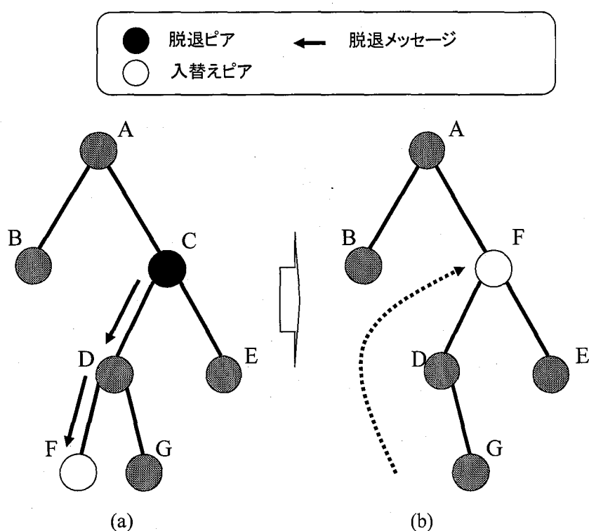
図 2.6: ピアの脱退例
