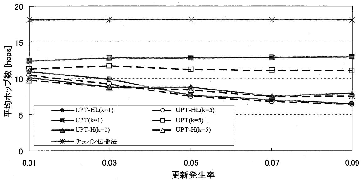
図 3.8: 平均ホップ数
