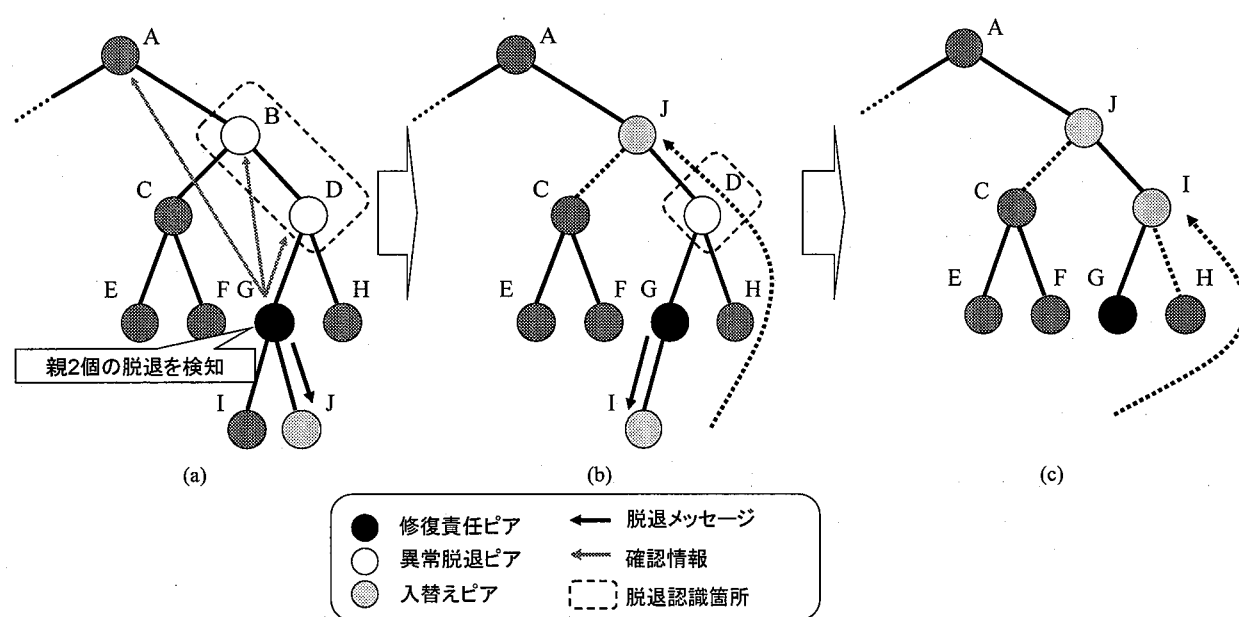
図 2.7: 異常脱退発生時の木の修復法
