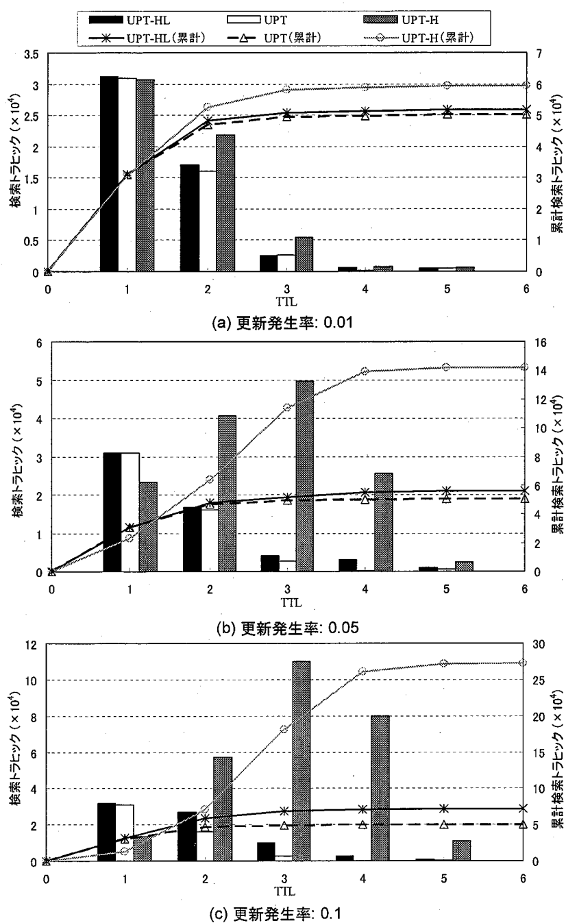
図 3.10: 検索トラフィック
