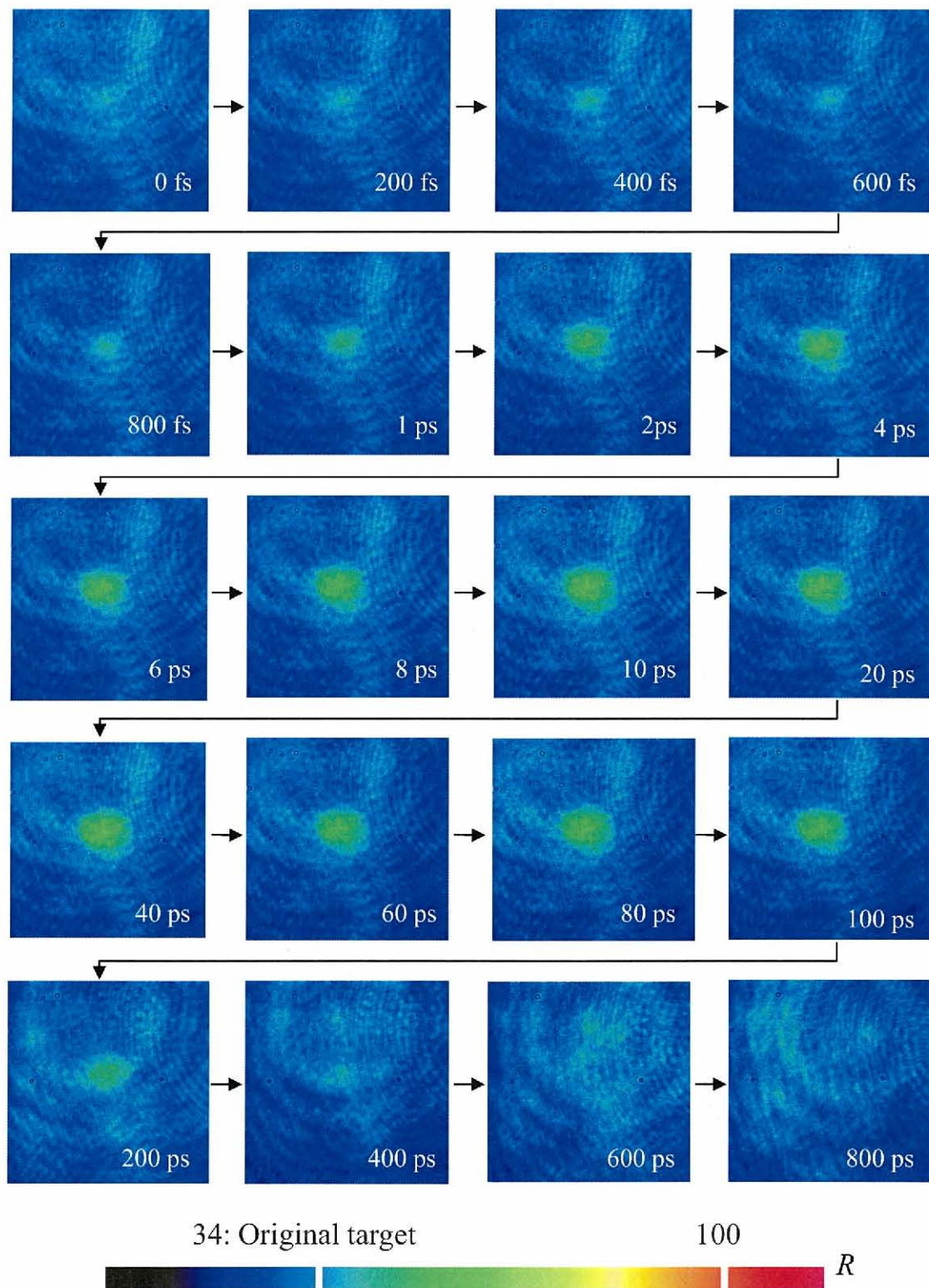
図 4-8 波長 800 nm のフェムト秒レーザー照射によって発生する a-Si 結晶化に対する Imaging Pump Probe 測定結果 (照射パルス数 : 1 pulse)
