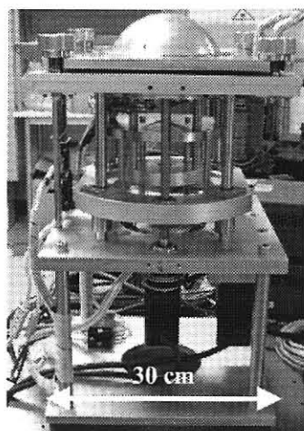
図 7-6 球面エキスパンド自動チップ化装置の概要
