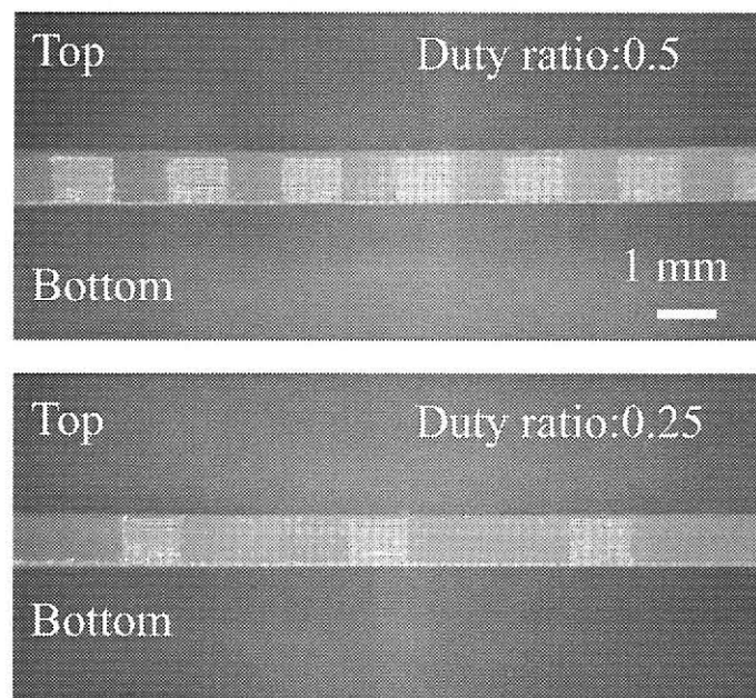
図 5-24 ミシン目内部加工を施したガラスウエハの割断面. 上図 Duty ratio 0.5, 下図 Duty ratio 0.25.
