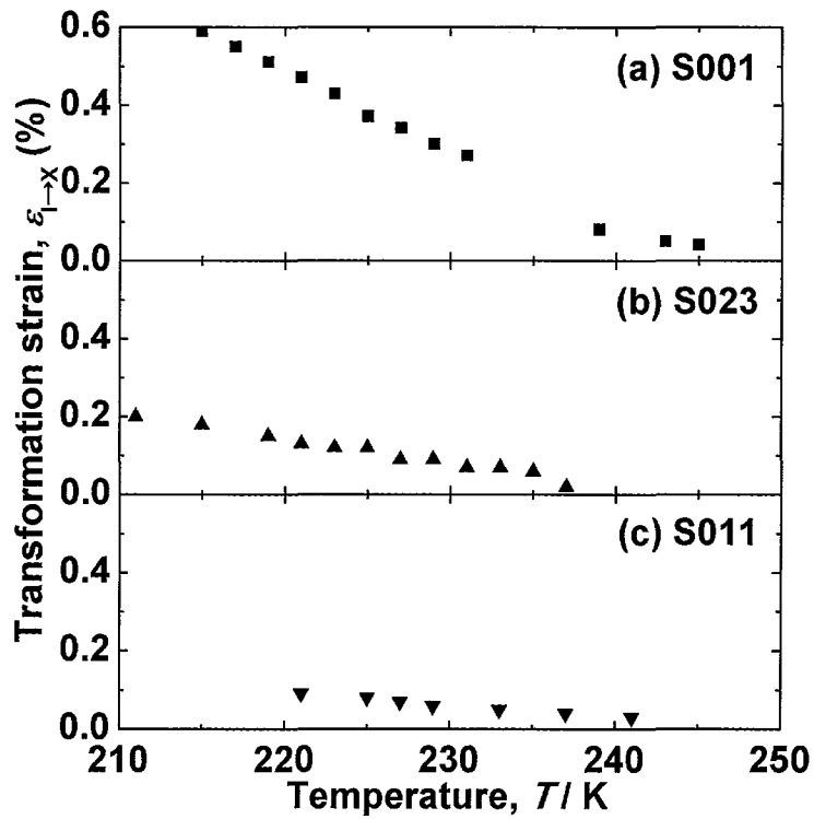
図 3-4 各温度における(a) S001、(b) S023 および(c) S011 の変態歪 \varepsilon_{I \leftrightarrow X}
