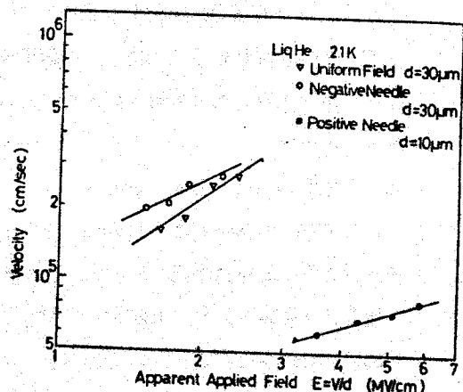
第3・54図 2.1Kでの v_f の見かけ上の電界依存性
