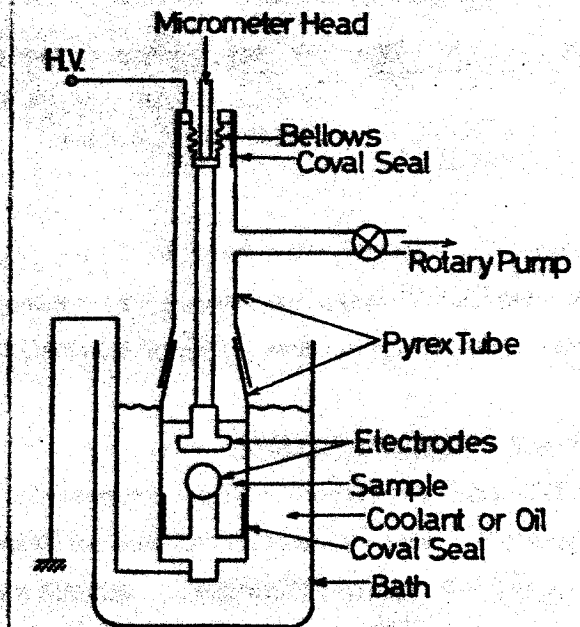
第 5.1 図 テストセルの概略図
