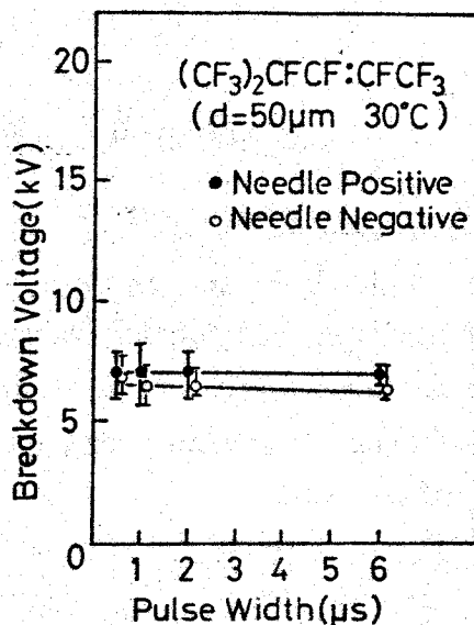
第5・8図 不平等電界下での perfluoro -trans-4-methyl-2-pentene の 破壊電圧の電圧パルス幅依存性
