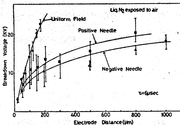
第4・5図 空気に曝した液体窒素の破壊電圧の電極間隔依存性
