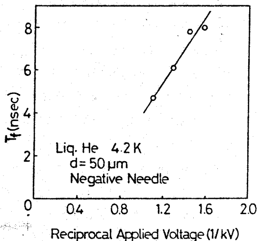
第3・45図 T_f の V^{-1} 依存性
