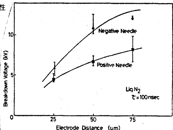
第4・2図 \tau = 100 \text{ n sec} での破壊電圧の電極間隔依存性
