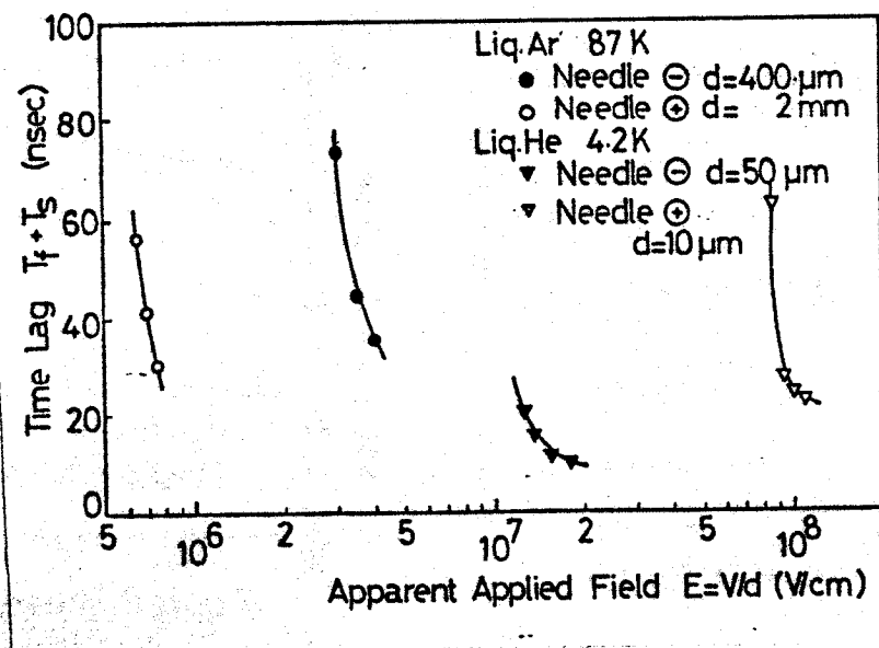
第3・51図 液体Ar及びHeに於ける (T_f + T_s) の見かけの電界依存性
