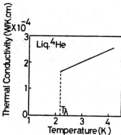
第3・5図 液体 ^4\text{He I} の熱伝導率
