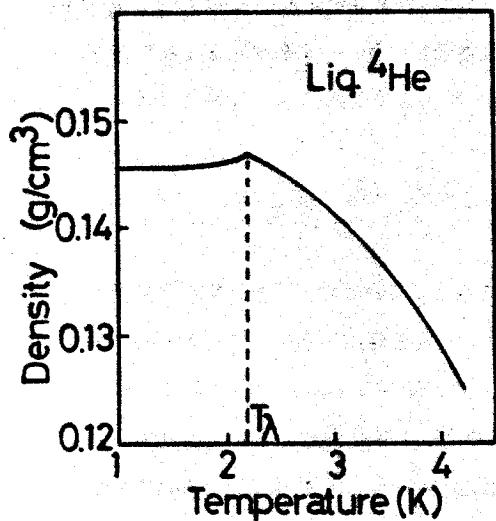
第3・2図 液体 ^4\text{He} の密度
