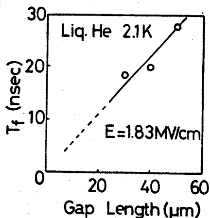
第3・39図 T_f の d 依存性
