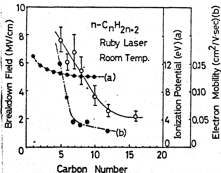
第6・4図 直鎖状炭化水素液体のルビーレーザー光による 破壊電界の n 依存性
