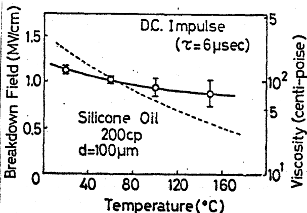
第 6・25 図 6 μ sec 電圧パルスによるシリコン油 (200 cp) の破壊電界の温度依存性 (d=100 μm) .....: 粘度の温度依存性 28)
