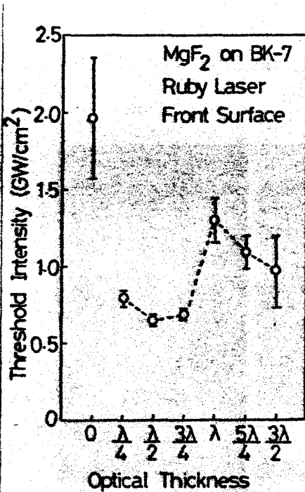
第7・4図 \text{MgF}_2 ガラスのルビーレーザー光による表面破壊光強度の膜厚依存性 ( \lambda=6948 \text{ \AA} )
