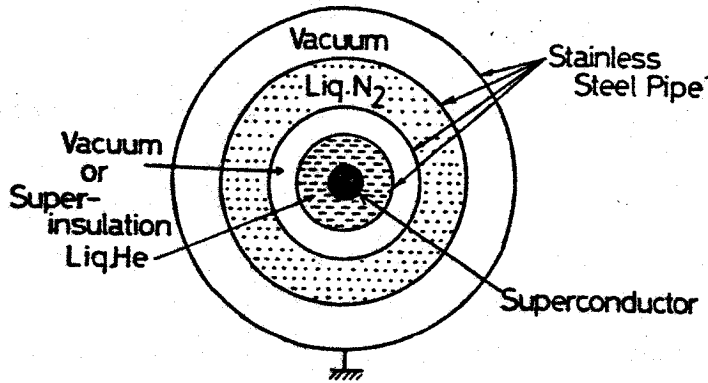
第1・1図，超電導直流ケーブルの概念図 11)
