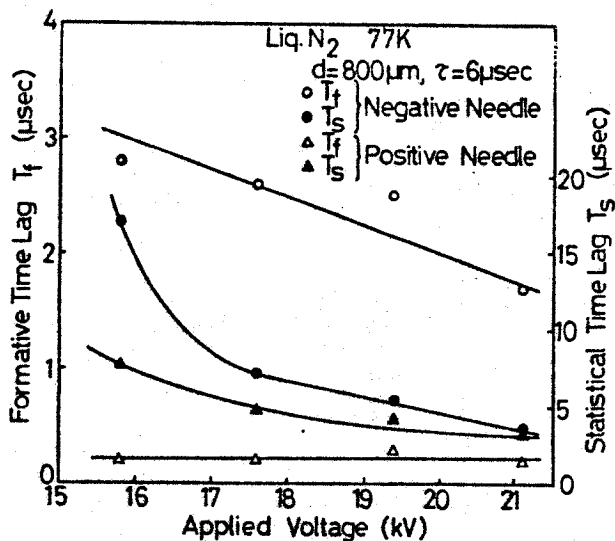
第4・9図 T_f , T_s の印加電圧依存性
