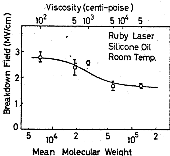
第6・21図 ルビーレーザー光によるシリコン油の破壊電界の平均分子量依存性
