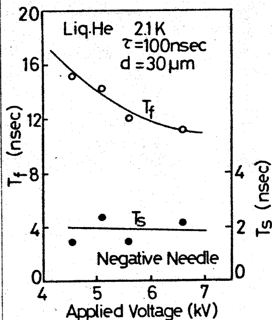
第3・52図 2.1K、負針、 d=30\mu\text{m} 、 \tau=100\text{nsec} 条件での T_f 、 T_s の電圧依存性
