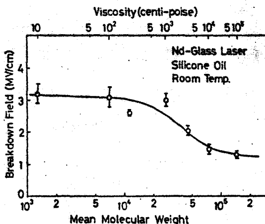
第6・20図 ガラスレーザー光によるシリコン油の 破壊電界の平均分子量依存性
