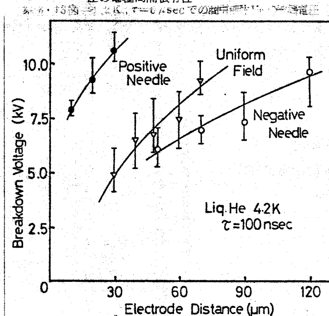
第3・14図 4.2 K, \tau=100\text{nsec} での商用液体Heの破壊電圧の電極間隔依存性
