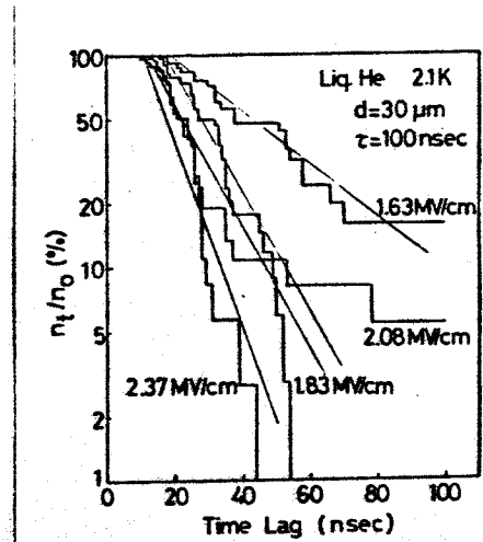
第3.36図 d = 30 \mu\text{m} , \tau = 100 \text{ nsec} での Laue プロット (2.1K)
