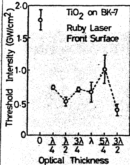
第7・5図 \text{TiO}_2 膜コートBK-7ガラスのルビーレーザー光による表面破壊光強度の膜厚依存性
