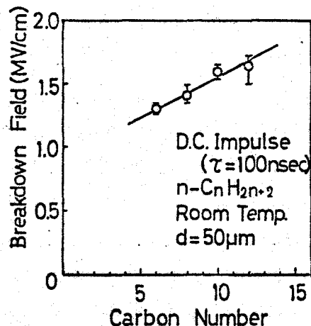
第6・5図 直鎖状炭化水素液体の 100 n sec 電圧パルスによる 破壊電界の n 依存性 (平等電 界, d = 50 \mu\text{m} )
