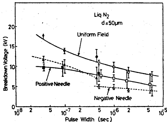
第4・4図 破壊電圧のパルス幅依存性 ( d = 50 \mu\text{m} )
