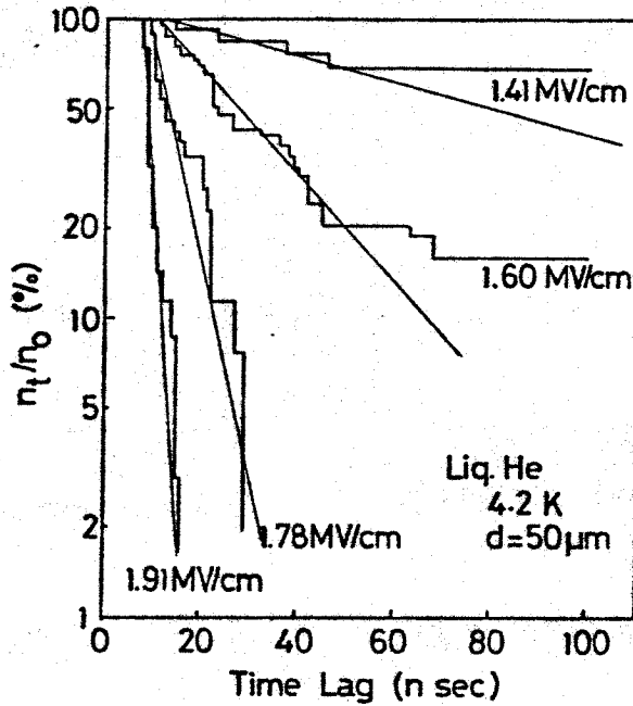
第3・29図 4.2 K, d=50\text{ }\mu\text{m} , \tau=100\text{ nsec} での破壊遅れのLaueプロット
