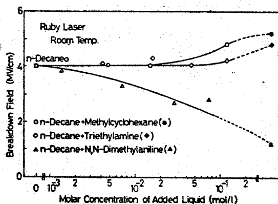
第6・15図 n-decaneに種々の液体を加えて行った時のルビーレーザー光による破壊電界の添加液体のモル濃度依存性
