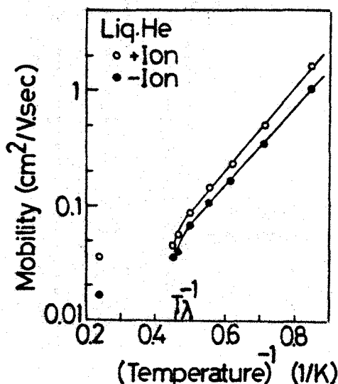
第3・8図 液体He中のキャリアの移動度
