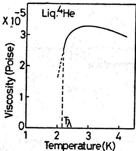
第3・4図 液体 ^4\text{He} の粘性率
