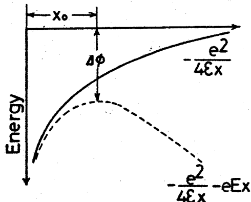
第2・7図 解離エネルギーの高電界での低下
