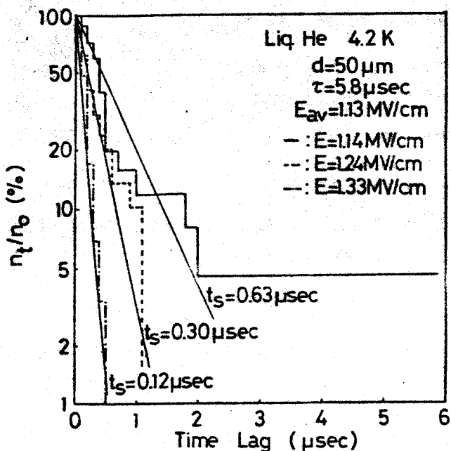
第3・28図 \tau=5.8 \mu sec パルスによる破壊遅れのLaueプロット(4.2K, d=50 \mu m )
