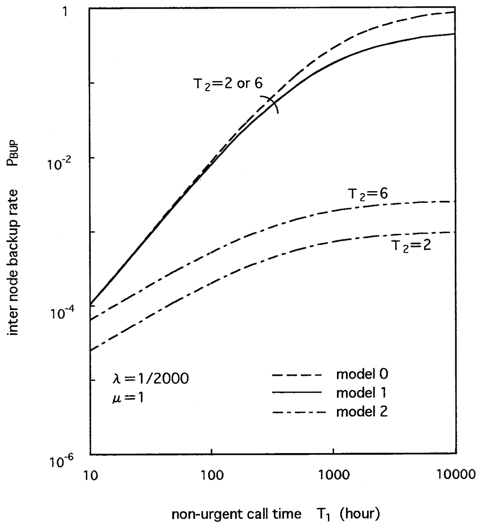
図 7.1 1 非緊急駆付け時間とノード間バックアップ率
