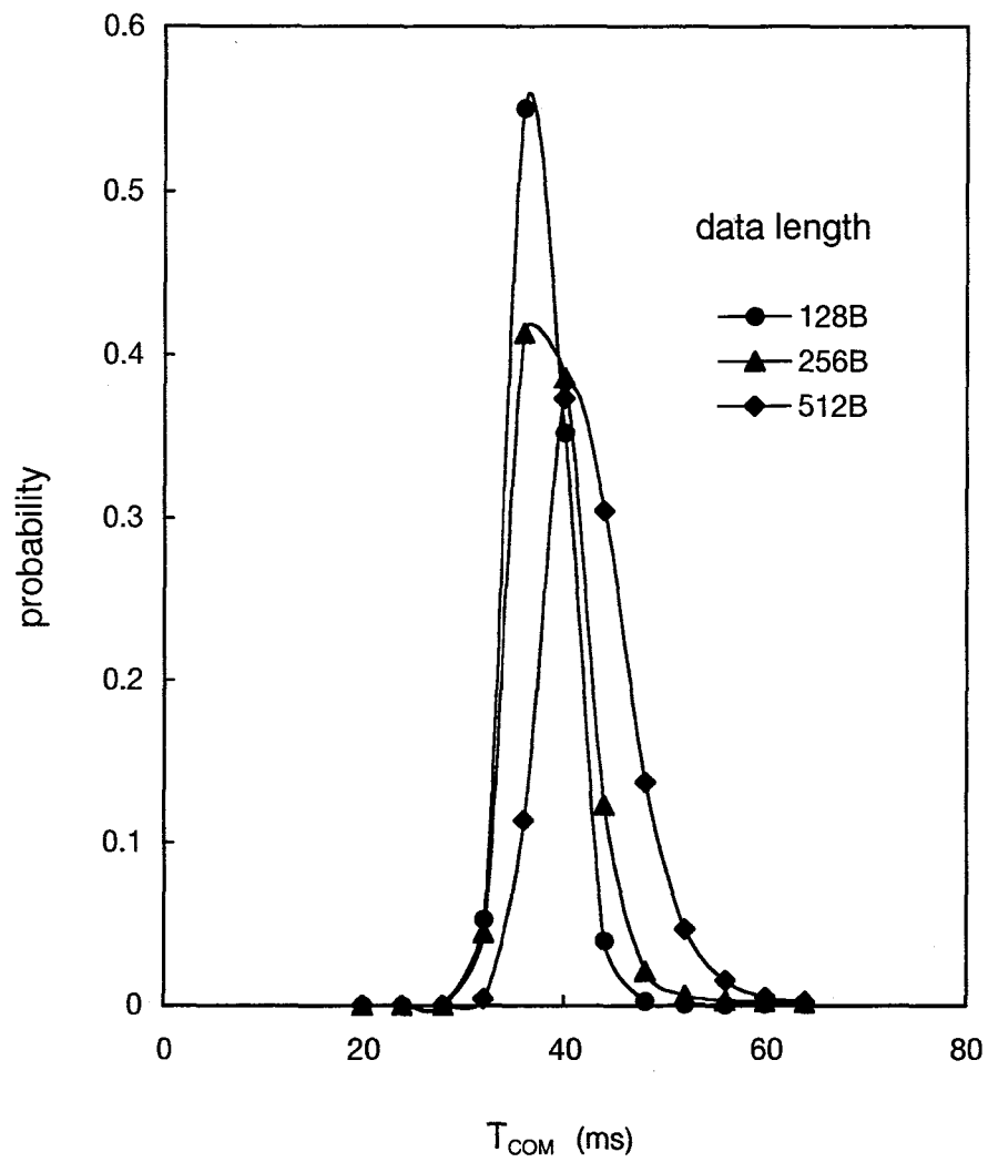
図 5.1 4 モジュール間の通信時間の分布
