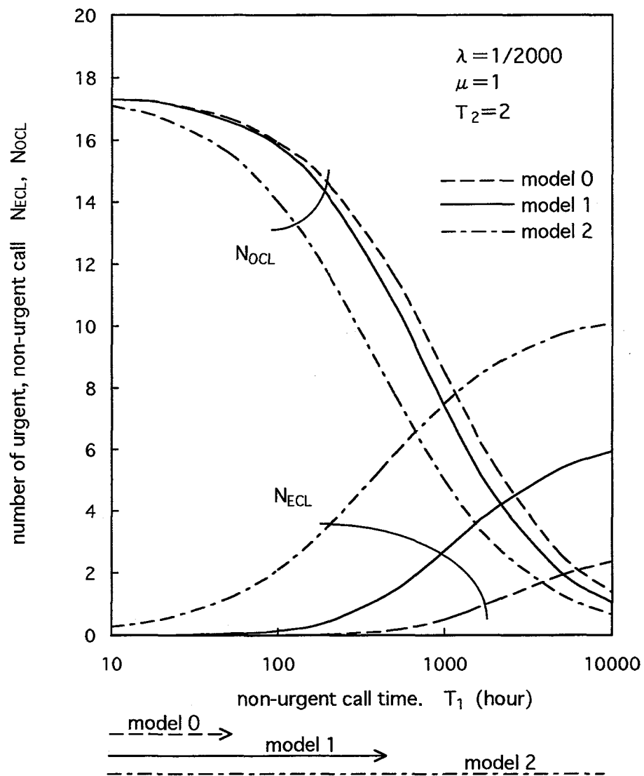
図 7.1 3 非緊急駆付け時間と緊急，非緊急駆付け回数
