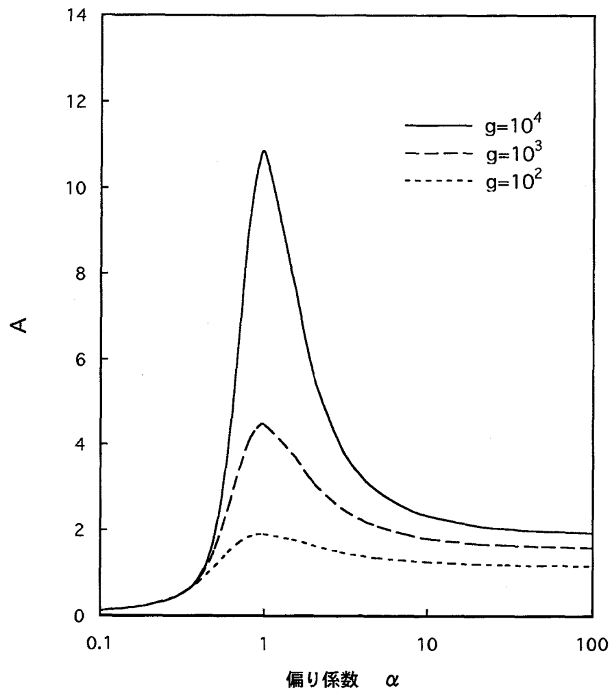
図4.9 \alpha と A の関係
