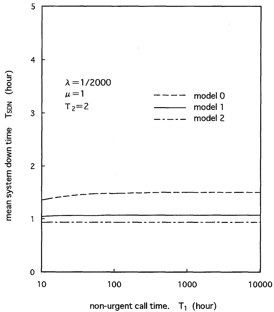
図 7.6 非緊急駆付け時間と平均システムダウン時間
