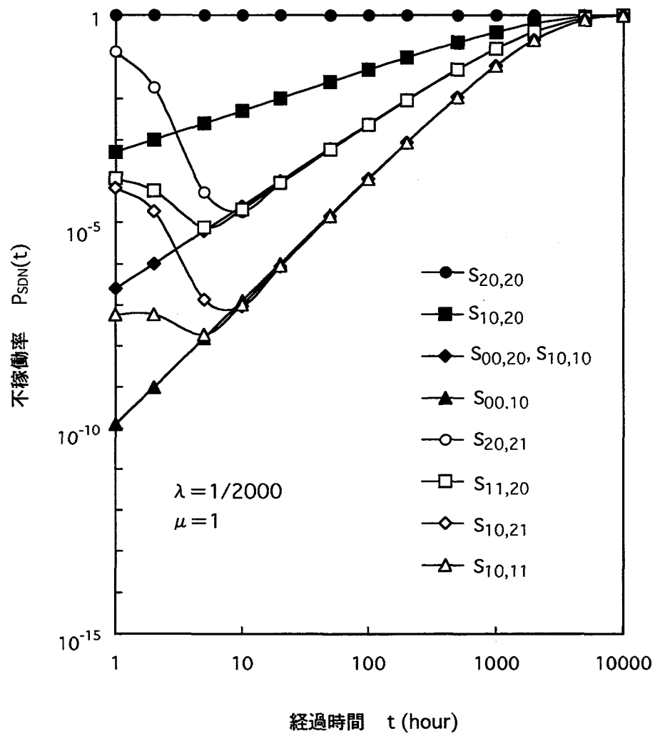
図 7.4 経過時間と不稼働率
