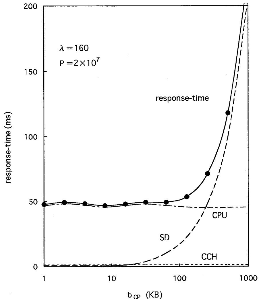
図A・6.2.2 b_{CP} とレスポンスタイムの関係
