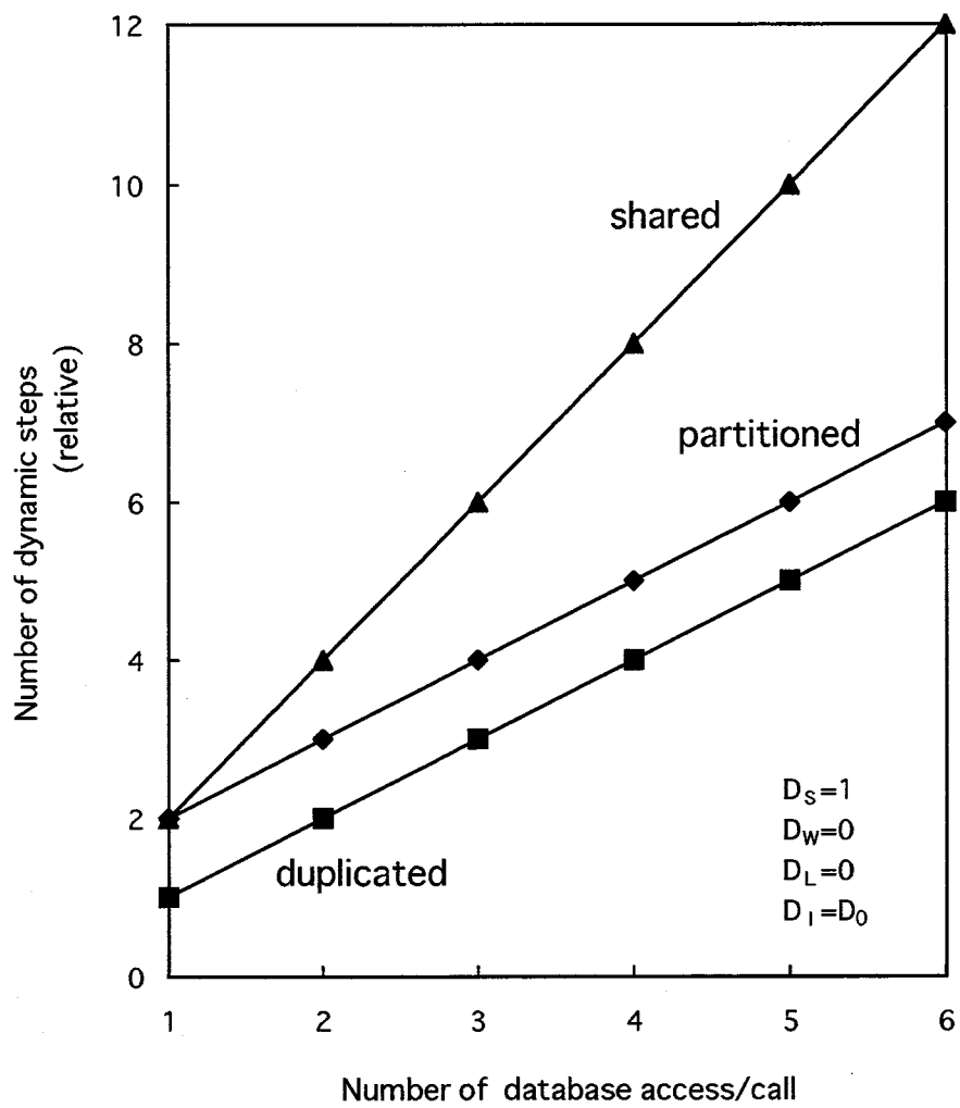
図 3.3 D S の比較 (参照系データベース)
