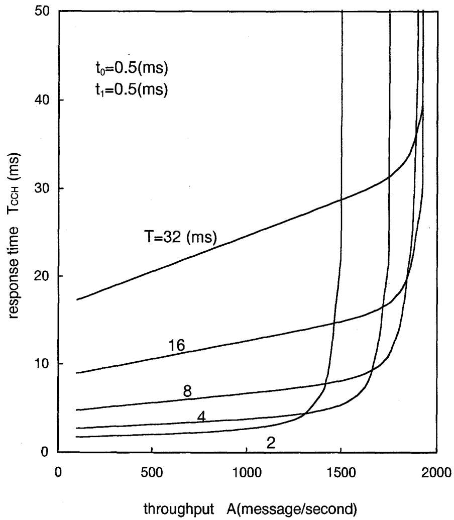
図 5.1.1 スループットと応答時間
