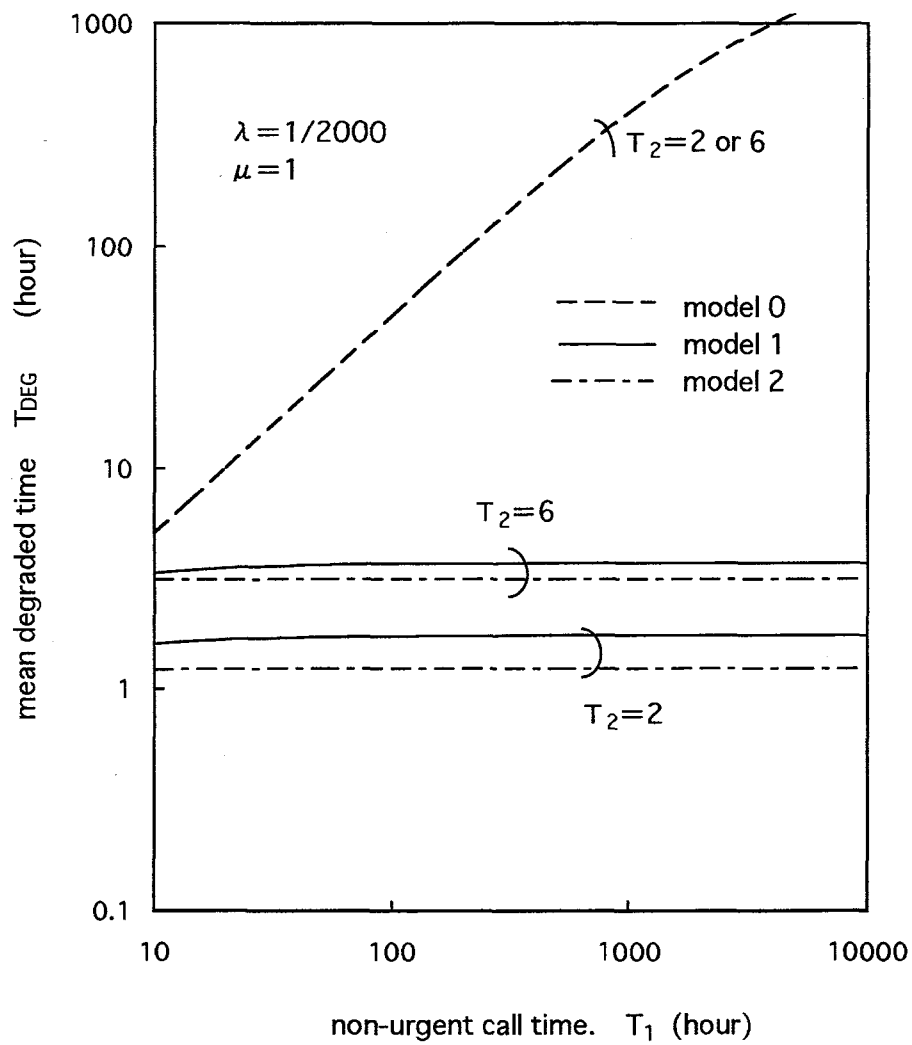
図 7.1 0 非緊急駆付け時間と平均デグレート時間
