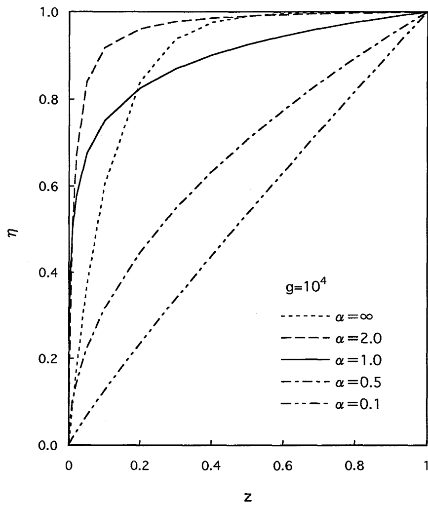
図4.5 z と \eta の関係
