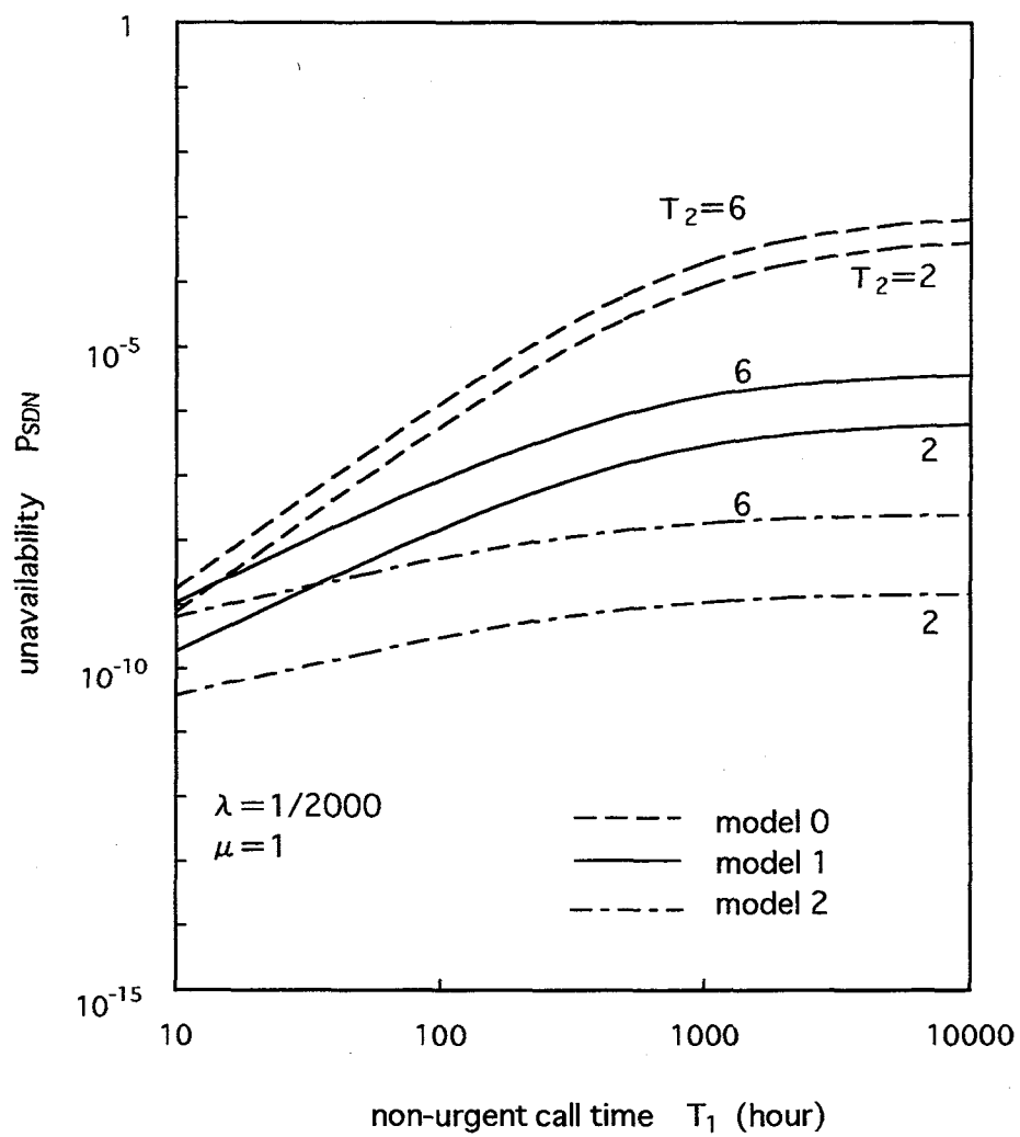
図 7.8 非緊急駆付け時間と不稼働率
