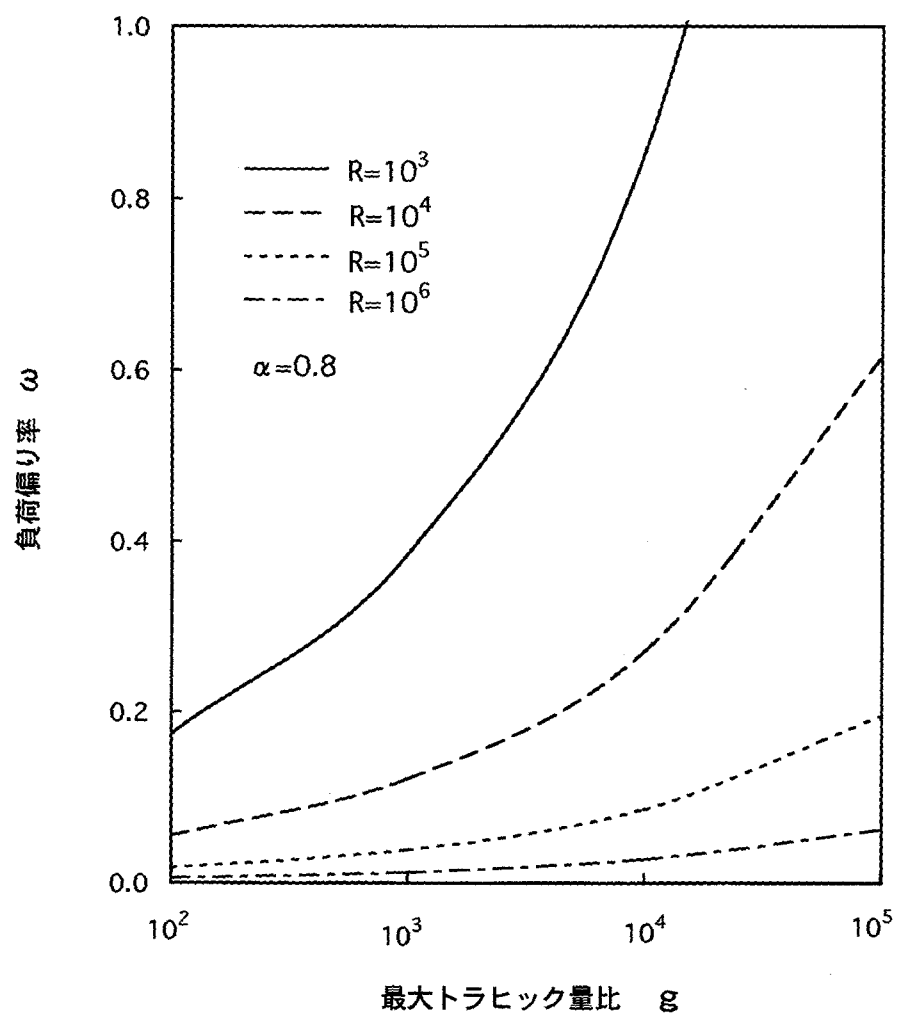
図4.8 g と \omega の関係
