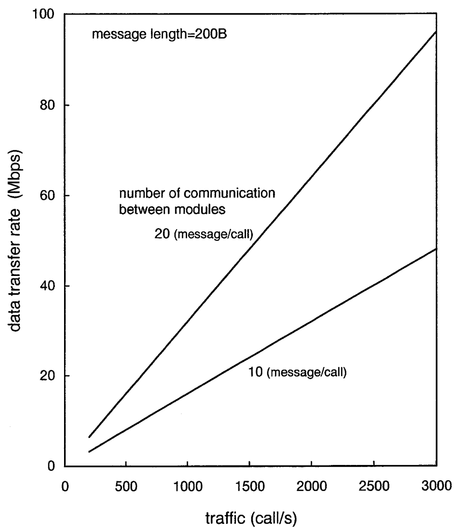
図 5.2 トラヒックとモジュール間のデータ転送量
