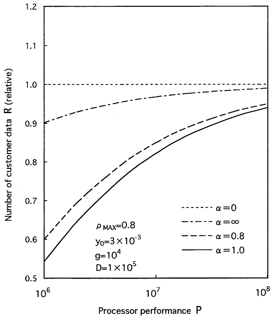
図 4.10 P と R の関係
