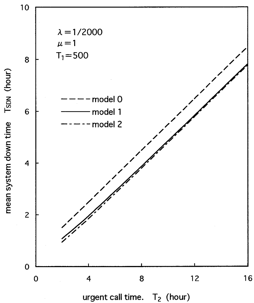
図 7.7 緊急駆付け時間と平均システムダウン時間
