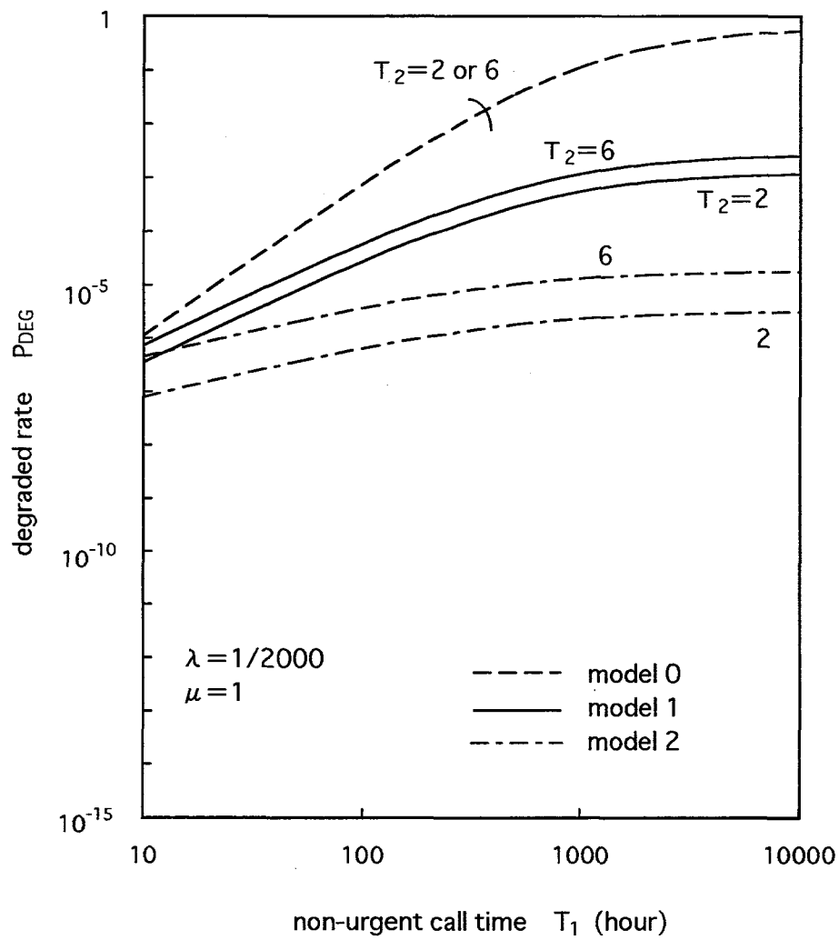
図 7.9 非緊急駆付け時間とデグレート率
