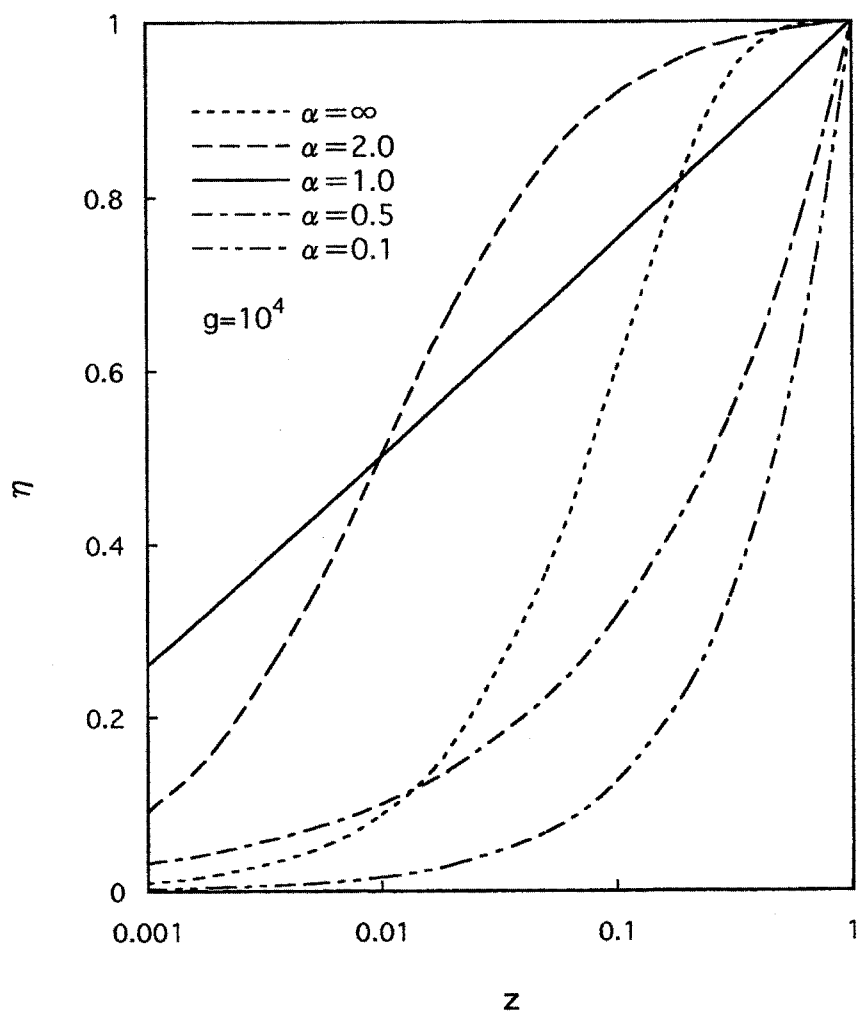
図 4.6 z と \eta の関係
