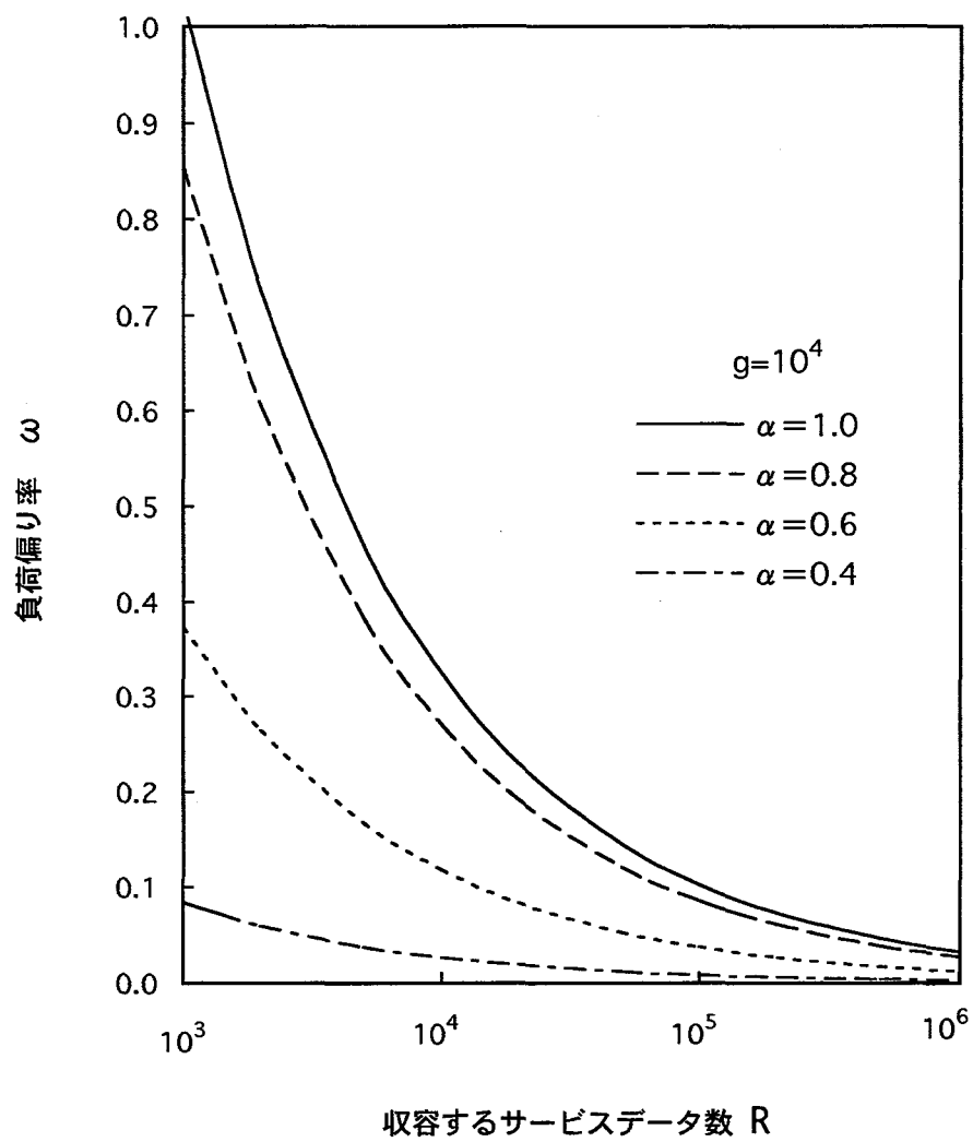
図4.7 R と \omega の関係
