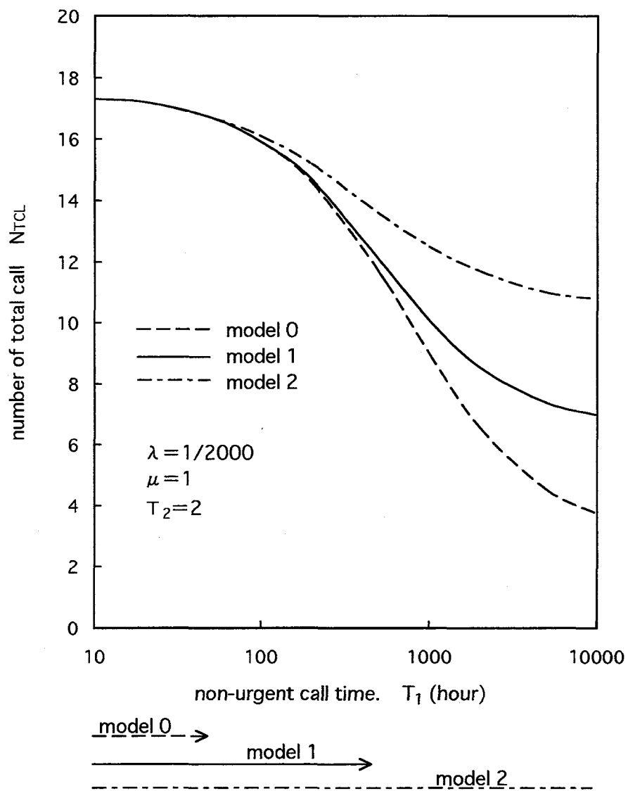
図 7.1 2 非緊急駆付け時間と総駆付け回数
