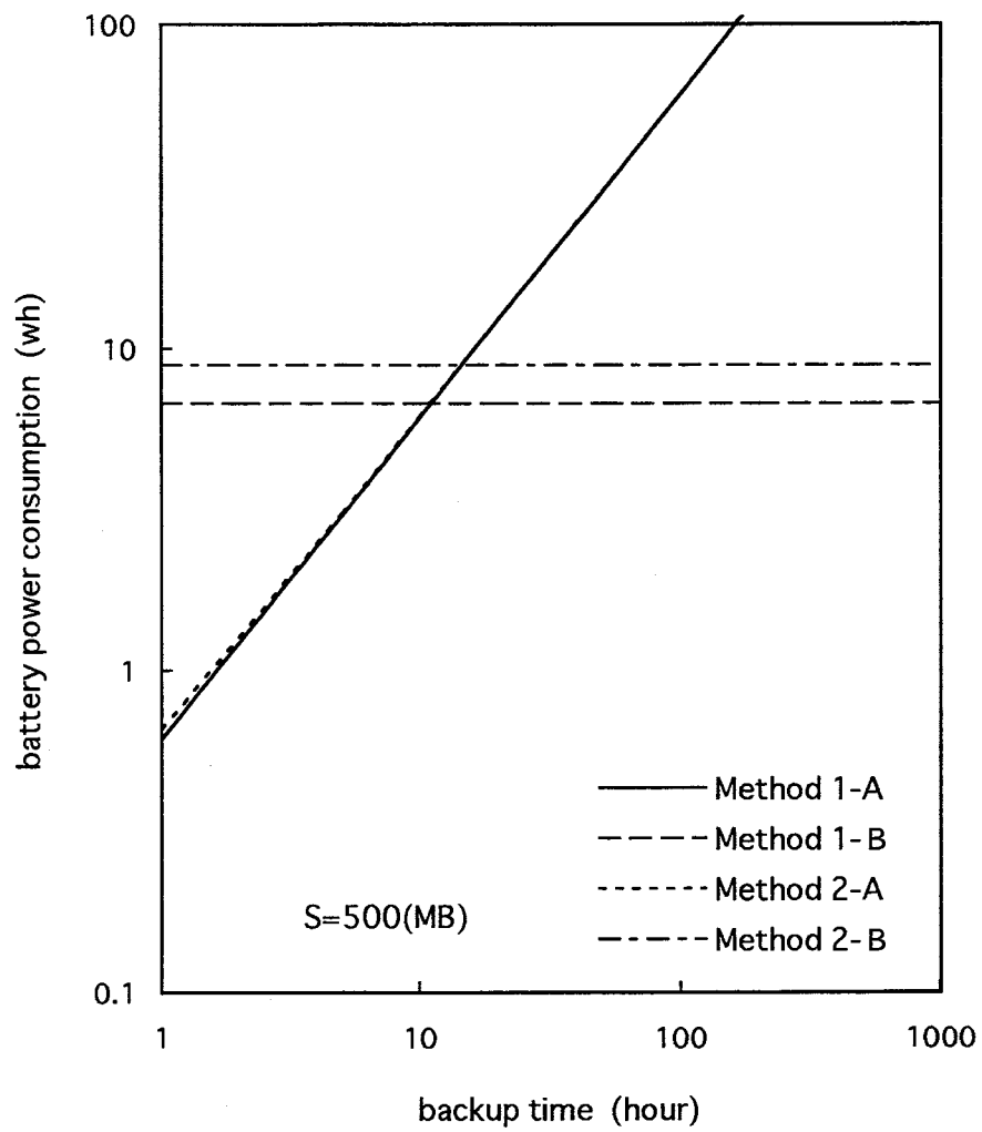
図 6.9 バックアップ時間とバッテリーの消費電力
