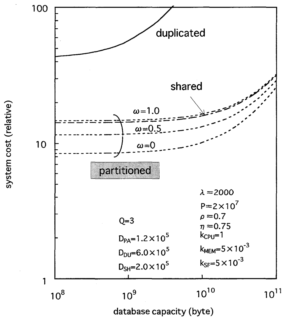
図 3.6 コスト比較（更新系データベース）
