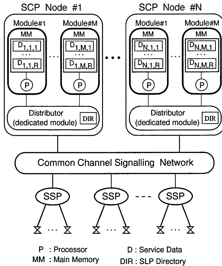
図 4.1 分散システム構成
