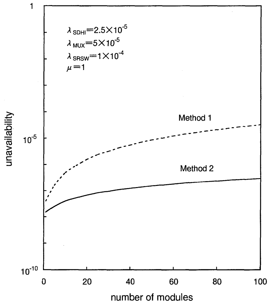
図 5.5 ATM結合機構の不稼働率
