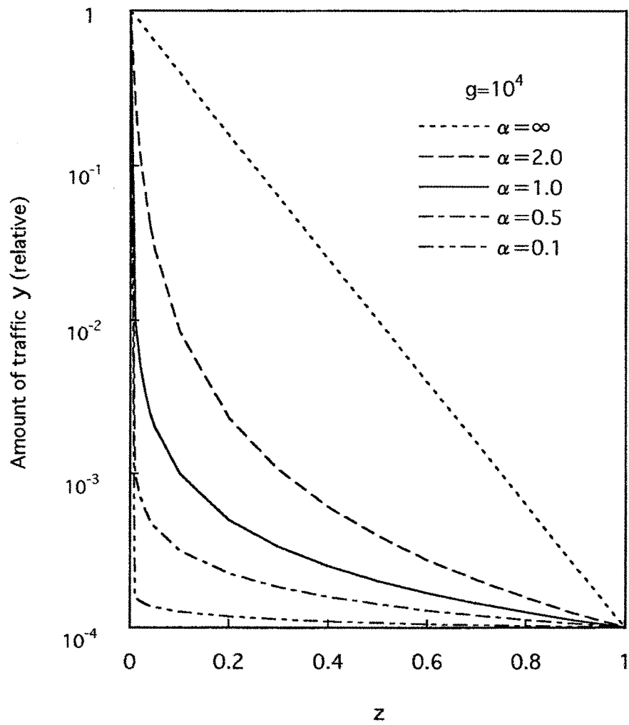
図4.4 トラヒック量
