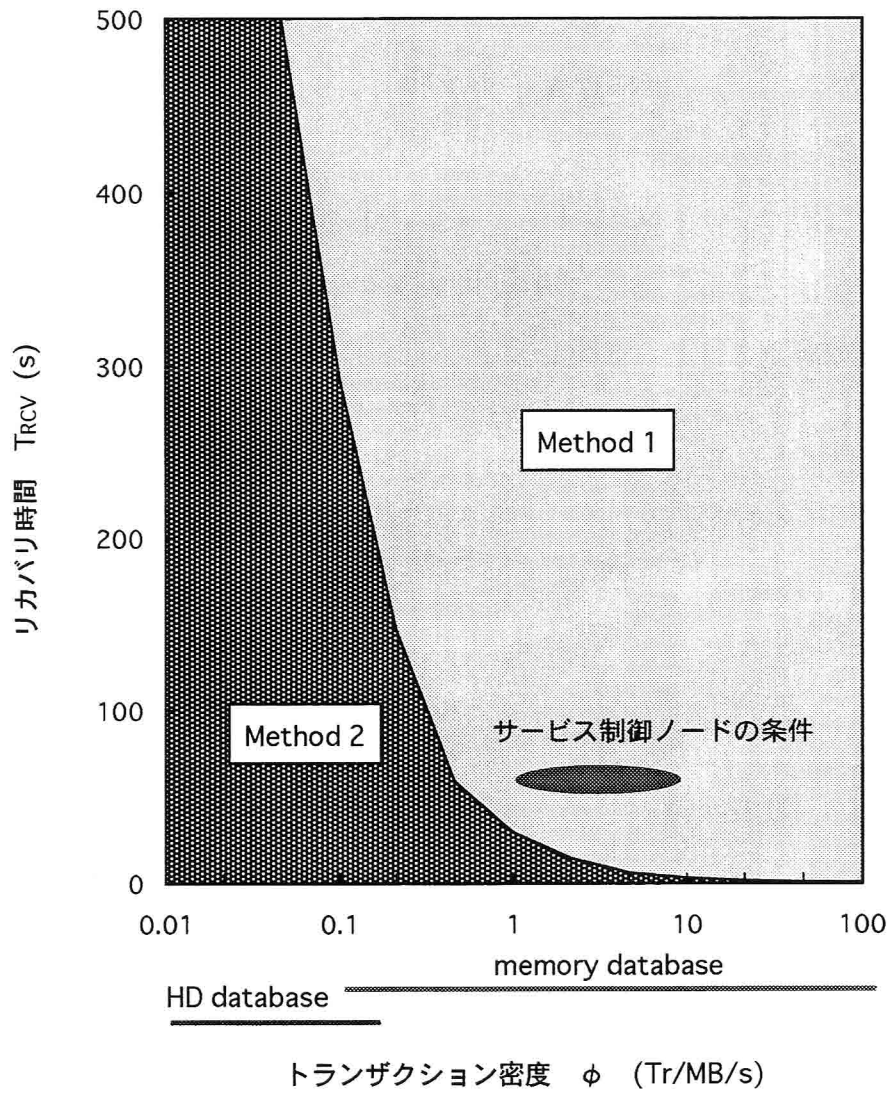
図 6.7 リカバリ方式の適用領域
