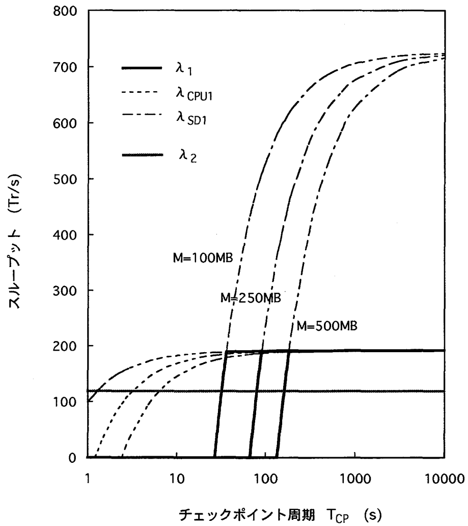
図 6.3 チェックポイント時間とスループット
