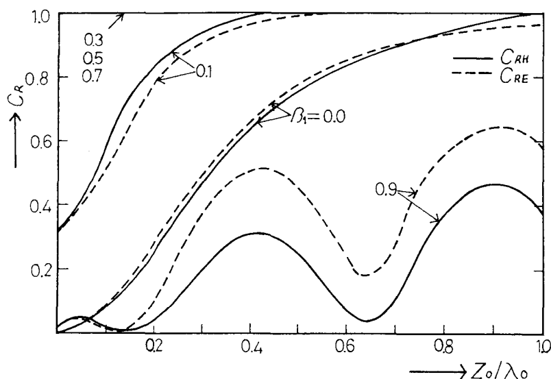
図 2.6 電力反射係数 C_R ( \epsilon_1^* = \epsilon_2^* = 4.0 \epsilon_3^* = 2.0, \beta_1 = \beta_2, \theta_i = 60^\circ )
