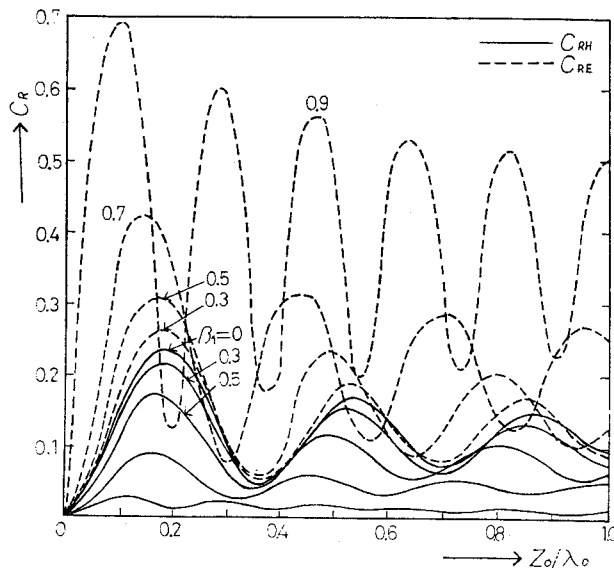
図2.5 電力反射係数 C_R ( \varepsilon_1^* = 1.0, \varepsilon_2^* = 4.0 \varepsilon_3^* = \varepsilon_4^* = 1.0, \theta_i = 0^\circ )
