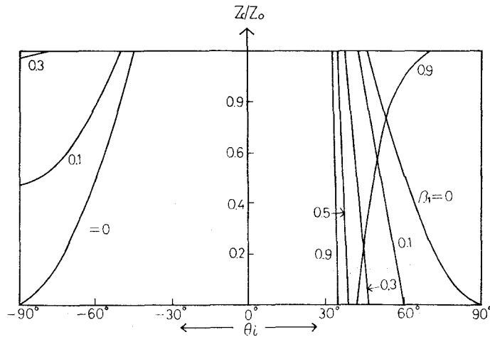
図2.4 幾何光学的反射点 Z_c/Z_o ( \epsilon_1^* = \epsilon_2^* = 4.0, \epsilon_3^* = 2.0 )
