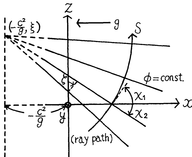
図5.1 加速系 \mathcal{L} 系における等位相面 \phi = \text{const.} ，ポインティングベクトル S および光線の軌跡
