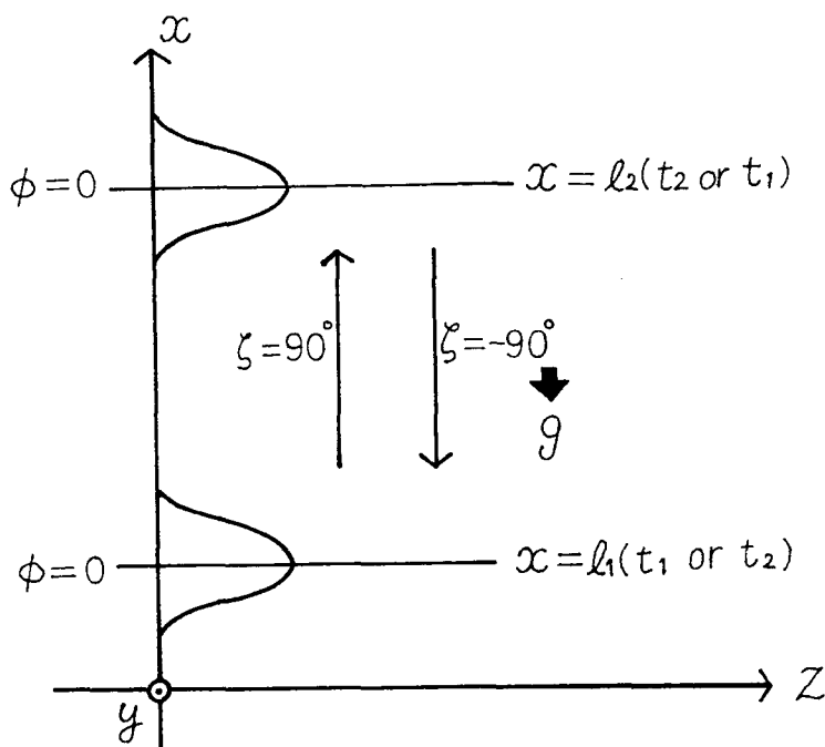
図 5.2 Pound-Rebka の実験
