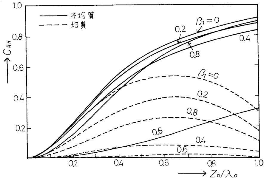
図 2.8 電力反射係数 C_{RH} ( \frac{\omega_B}{\omega} = 0, \frac{\omega_B}{\omega} = 1.3, \theta_i = 0^\circ, Z_{cp}/Z_0 = 0.59 )
