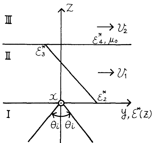
図2.1 座標系および媒質Ⅰ,ⅡおよびⅢの比誘電率
