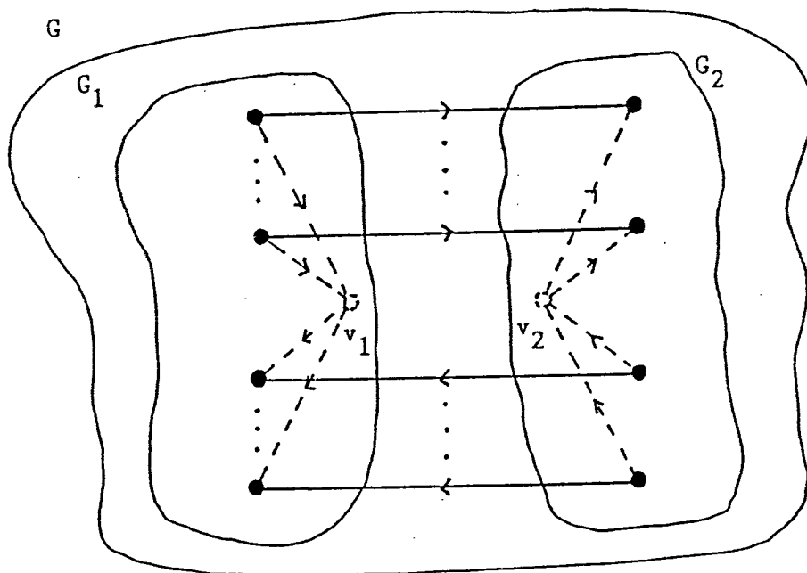
図 6. 11 グラフの合成法 dmerge1(G_1, IE_1, OE_1, G_2, OE_2, IE_2) .
