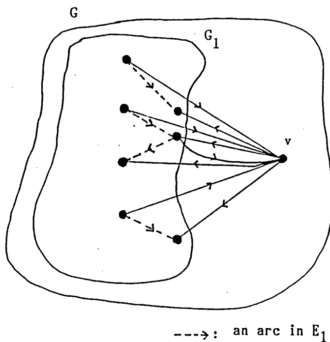
図 6. 12 グラフの合成法 dmerge2(G_1, E_1', v) .
