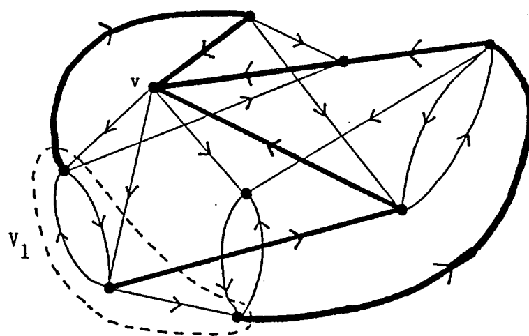
(c) A (V_1, v) -fanin.
