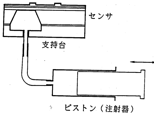
図3-12 圧力印加法
