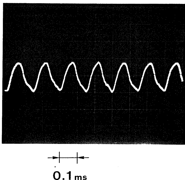
図 4 - 1 9 カンチレバ共振時の光出力
