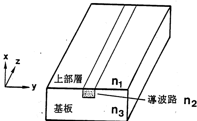
(b) チャネル導波路
