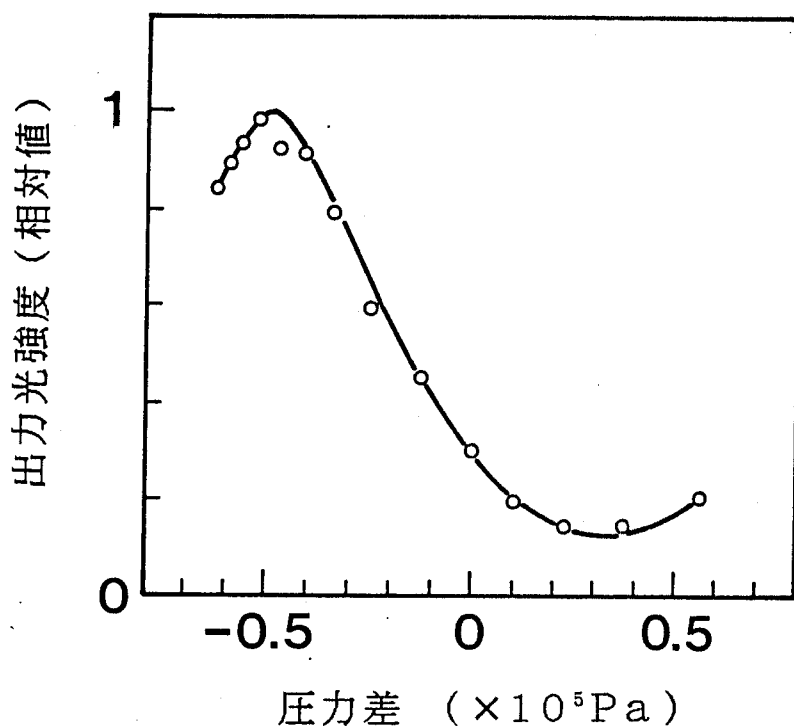
図3-13 測定結果
