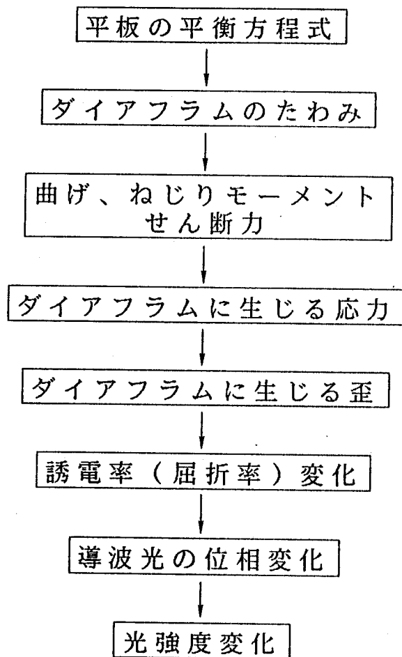
図 3 - 3 解析手順
