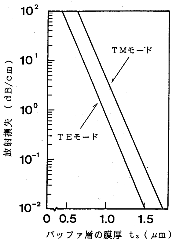
図 2-6 バッファ層の膜厚とシリコンへの放射損失の関係
