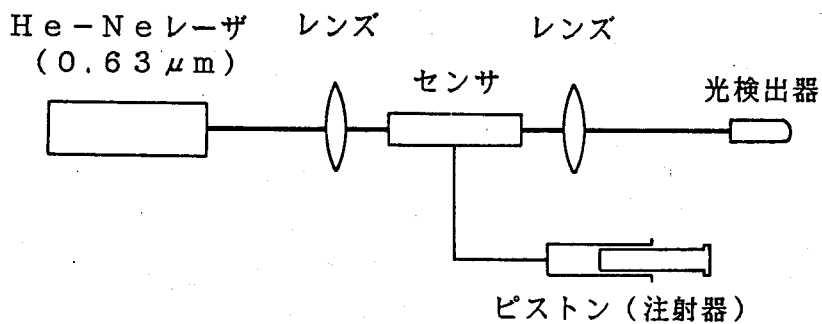
図3-11 測定系
