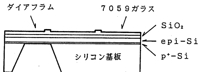
(b) 断面図
