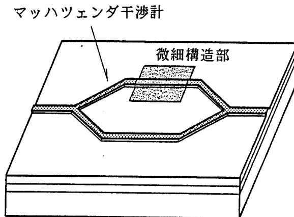
図 2 - 1 6 マッハツェンダ干渉計を用いた 光集積回路センサの構成
