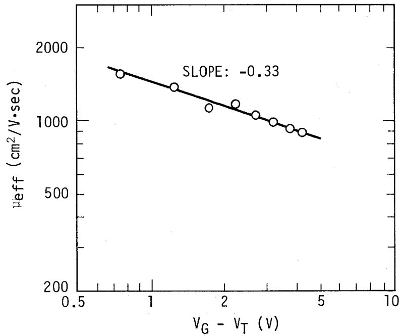
図 5-13 電子の実効移動度 ( \mu_{\text{eff}} ) のゲート電圧 ( V_G ) 依存性 ( V_T : 閾値電圧)
