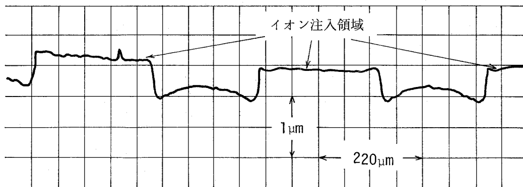
図3-5 窒素イオン注入と光照射電解エッチングを併用した半絶縁性 GaAs 表面のマスクレス選択エッチング
