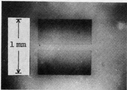
図 4.15 円筒型ゾーンプレート・レンズの顕微鏡写真 ( f = 5\text{ mm} ; \lambda = 0.6328\text{ }\mu\text{m} )
