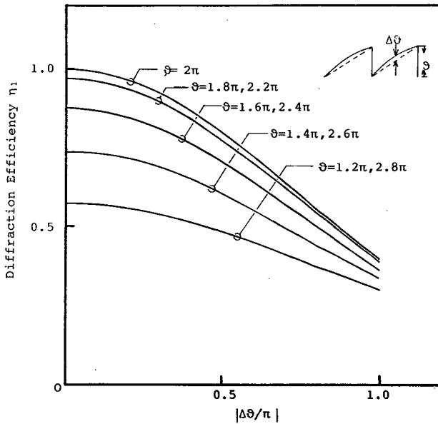
図 2.8 1次回折効率 \eta_1 の位相形状依存性, \eta_1 と (\theta, \Delta\theta) の関係
