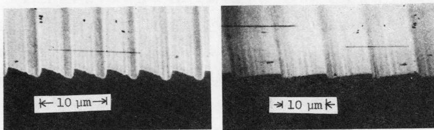
図 5.7 ブレーズドグレーティングの断面 S E M 写真,
