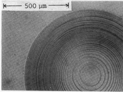
図 5.8 作製したマイクロ・フレネルレンズ ( f=5\text{mm} , \lambda=0.6328\text{ }\mu\text{m} )
