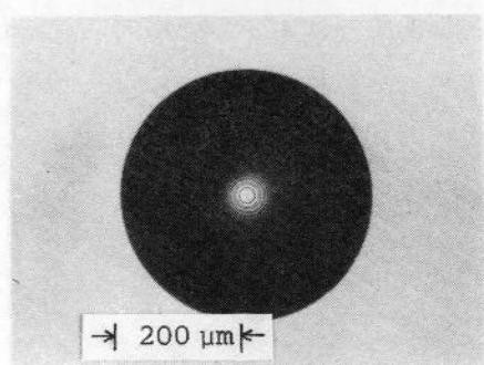
図 4.9 作製したマイクロ・ゾーンプレート・レンズ ( f=0.26\text{ mm} ， 2d=0.4\text{ mm} ； \lambda=0.6328\text{ }\mu\text{m} )
