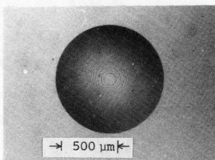
図 4.8 作製したマイクロ・ゾーンプレート・レンズ ( f=5\text{ mm} ， 2d=1\text{ mm} ； \lambda=0.6328\text{ }\mu\text{m} )
