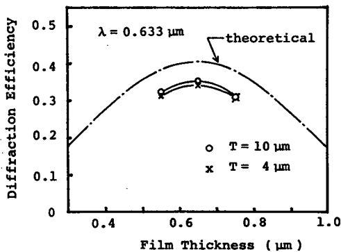
図 4.4 1 次回折効率の PMMA 膜厚依存性
