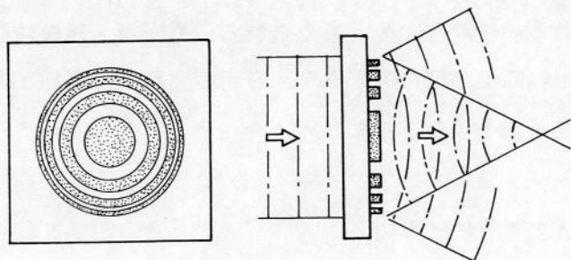
図 4.7 ゾーンプレート・レンズの構造
