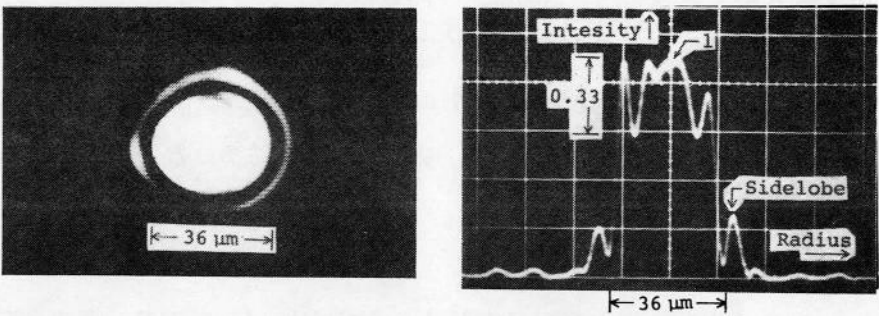
図 6.13 焦点面上の光強度分布，(a) TV モニタ像， (b) TV カメラからの映像信号のトレース
