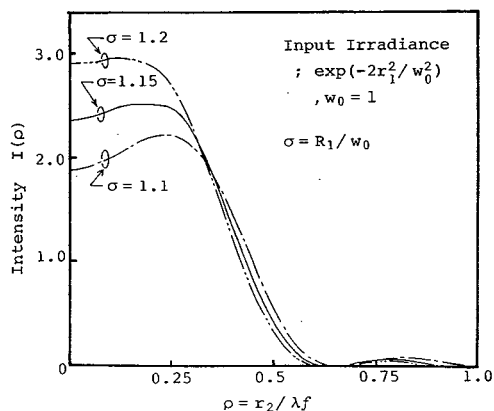
図 6.16 光強度分布変換特性
