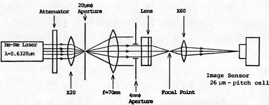
図 4.10 スポット径測定系
