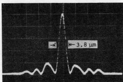
図 5.15 円筒型フレネルレンズ ( f = 5\text{mm} ; 2d = 1\text{mm} )
