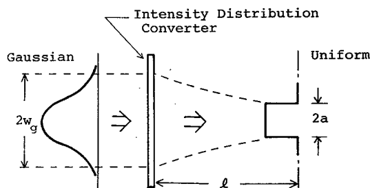
図 6.1 強度分布変換用レンズの機能
