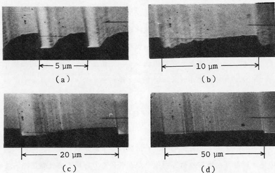
図 5.3 PMMA 化学エッチング特性測定用グレーティングの断面 SEM 写真, (a) 周期 5\ \mu\text{m} , (b) 10\ \mu\text{m} , (c) 20\ \mu\text{m} , (d) 50\ \mu\text{m}
