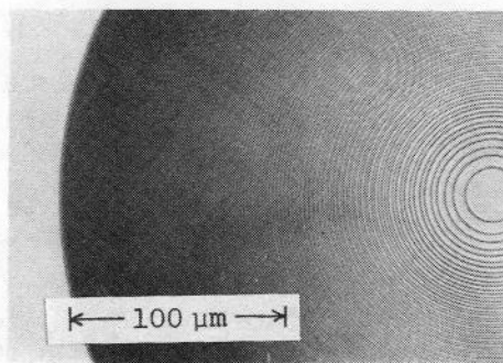
図 4.9 作製したマイクロ・ゾーンプレート・レンズ ( f=0.26\text{ mm} ， 2d=0.4\text{ mm} ； \lambda=0.6328\text{ }\mu\text{m} )
