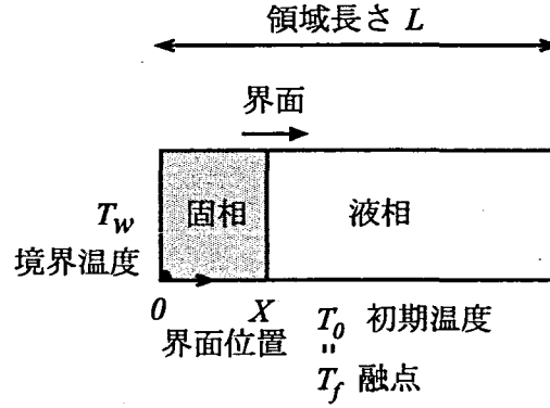
図. 5.5: 1次元凝固問題の計算対象図
