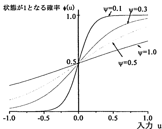
図. 5.11: ニューロンの入出力関数 (ボルツマンマシン) [11]
