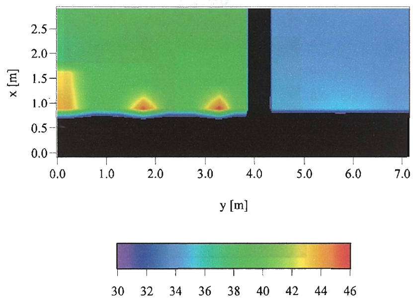
図. 3.11: A-A' 断面における 15 時の平均放射温度分布 [°C] (Case1, z=7.1\text{m} )
