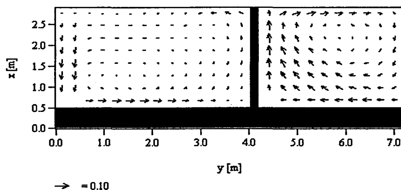
図. 3.10: A-A' 断面における 15 時の速度ベクトル [m/s] (Case1, z=7.1\text{m} )
