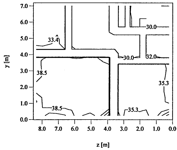
図. 3.8: y-z 断面における 15 時の温度分布 [°C] (Case1, x=1.6\text{m} )
