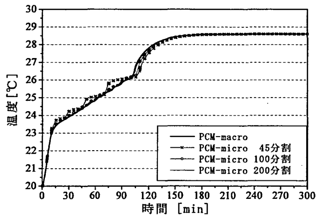
図. 6.5: 冷却側表面温度の比較
