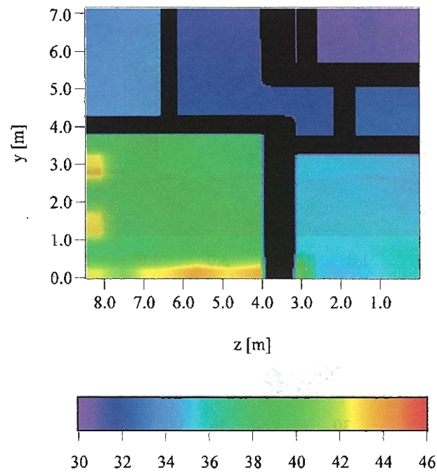
図. 3.14: y-z 断面における 15 時の平均放射温度分布 [°C] (Case3, x=1.6\text{m} )
