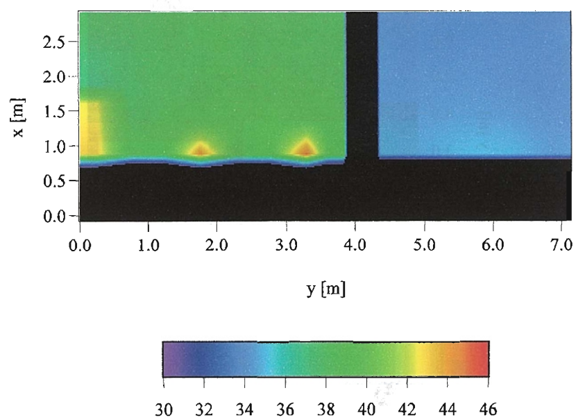
図. 3.12: A-A' 断面における 15 時の平均放射温度分布 [°C] (Case3, z=7.1\text{m} )
