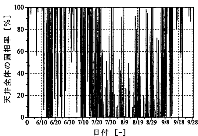
図. 6.25: 天井面における PCM 壁ボード全体の固相率の予測結果 (長野, CaseF, 6/1~9/30)
