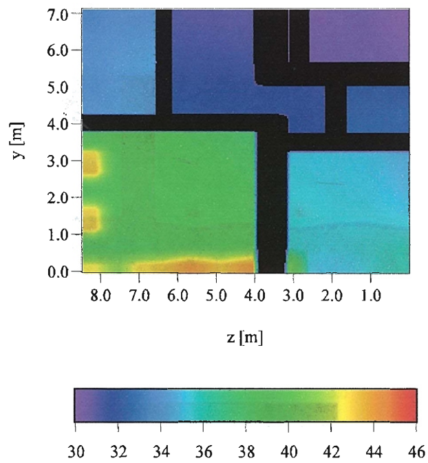
図. 3.13: y-z 断面における 15 時の平均放射温度分布 [°C] (Case1, x=1.6\text{m} )
