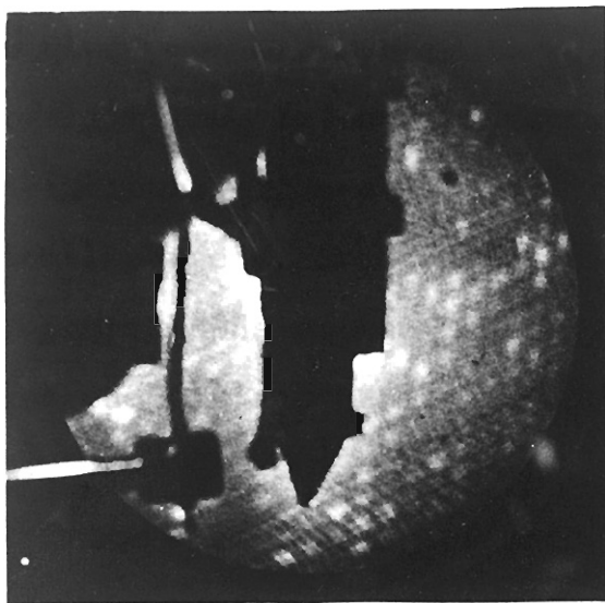
Si(111) 7x7 E = 76 eV
