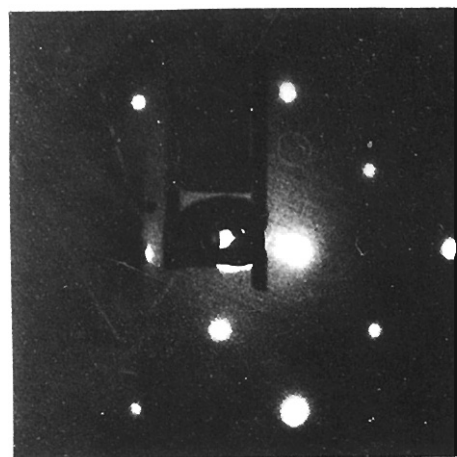
clean MgO (001) 138V
