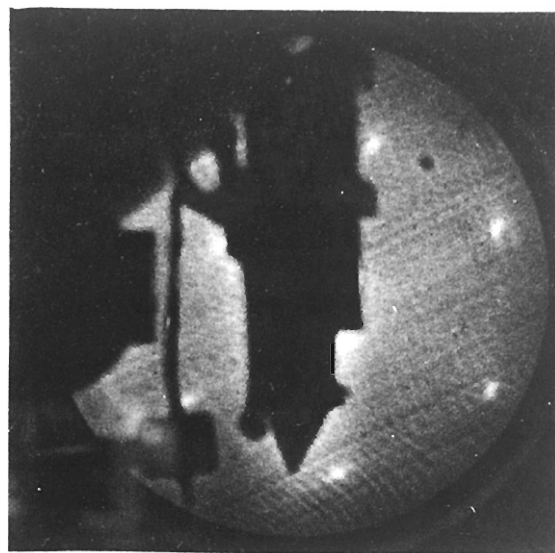
Fe/Si(111) 1x1 E = 81 eV
