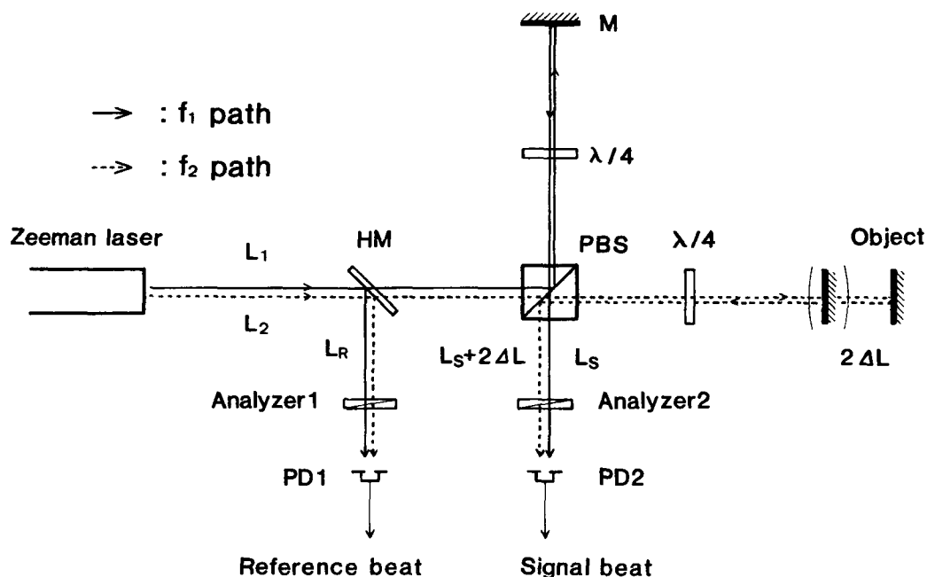
図7.1 二周波直交偏光干渉光学系の構成例
