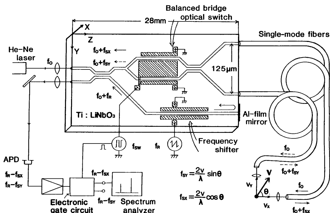
図6.1 提案した時分割2次元速度計測用光集積回路デバイス
