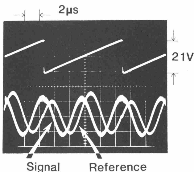
図7.8 観測したビート信号波形
