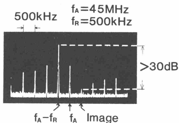
図5.6 セロダイン形周波数シフタの出力光の周波数スペクトル
