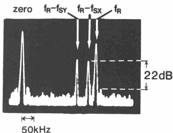
図6.10 スイッチングゲートを駆動しないときに観測した周波数スペクトル
