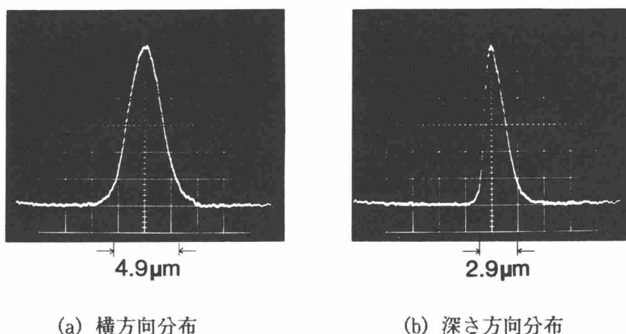
図2.5 作製したZ軸伝搬 \text{LiNbO}_3 導波路の出射光強度分布(波長 0.633\mu\text{m} )
