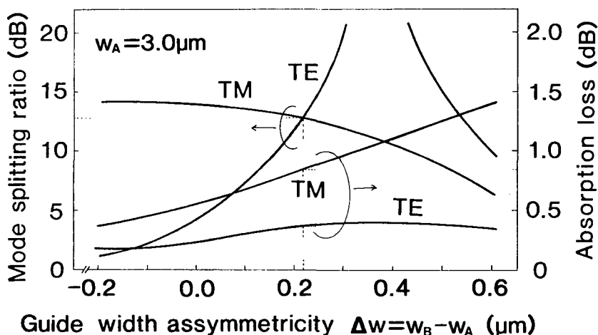
図3.9 導波路幅の非対称性に対するモードスプリッティング比と吸収損失の関係
