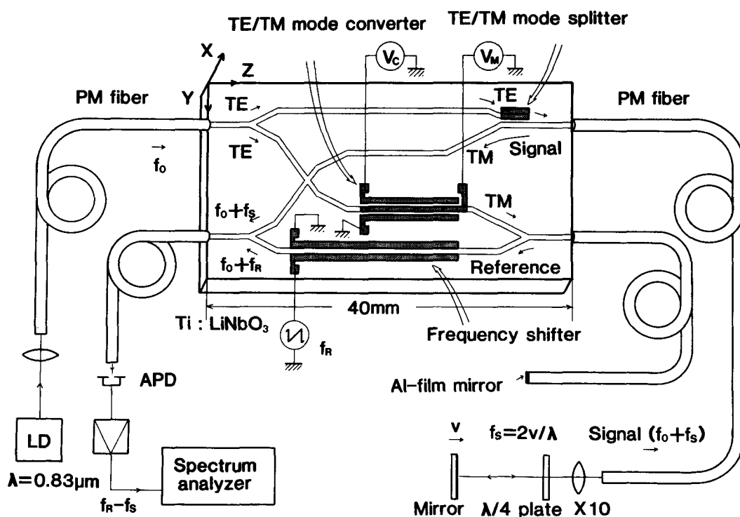
図5.5 0.8\text{ }\mu\text{m} 帯FP形半導体レーザを用いたLDV用光集積回路デバイスの構成
