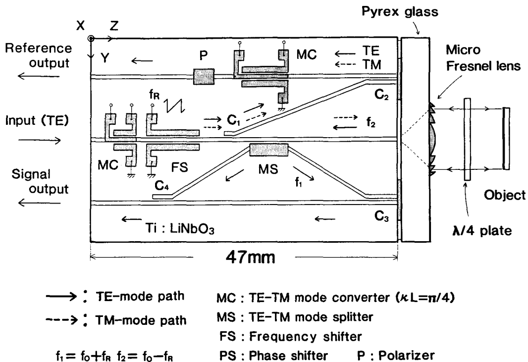
図7.2 提案した変位計測用光集積回路デバイスの構成
