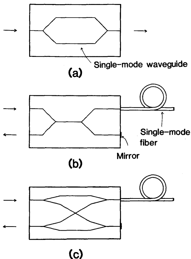
図2.7 単一モードチャネル導波路における導波形干渉計の構成例
