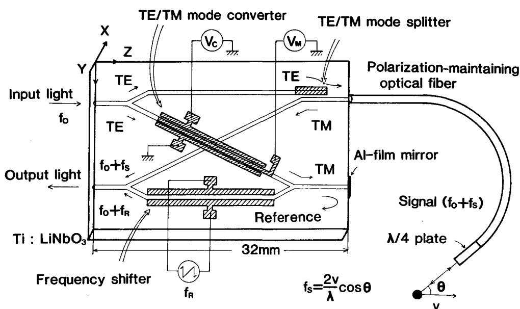
図2.8 提案したLDV用光集積回路デバイスの構成
