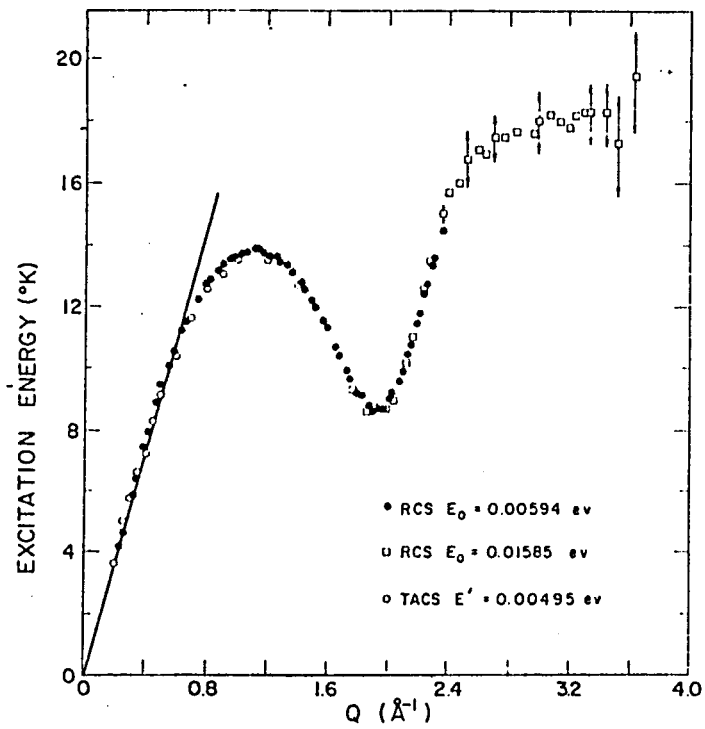
Fig.6 1.1°Kでの液体He 4 の単一フォンのエネルギースペクトル 35)
