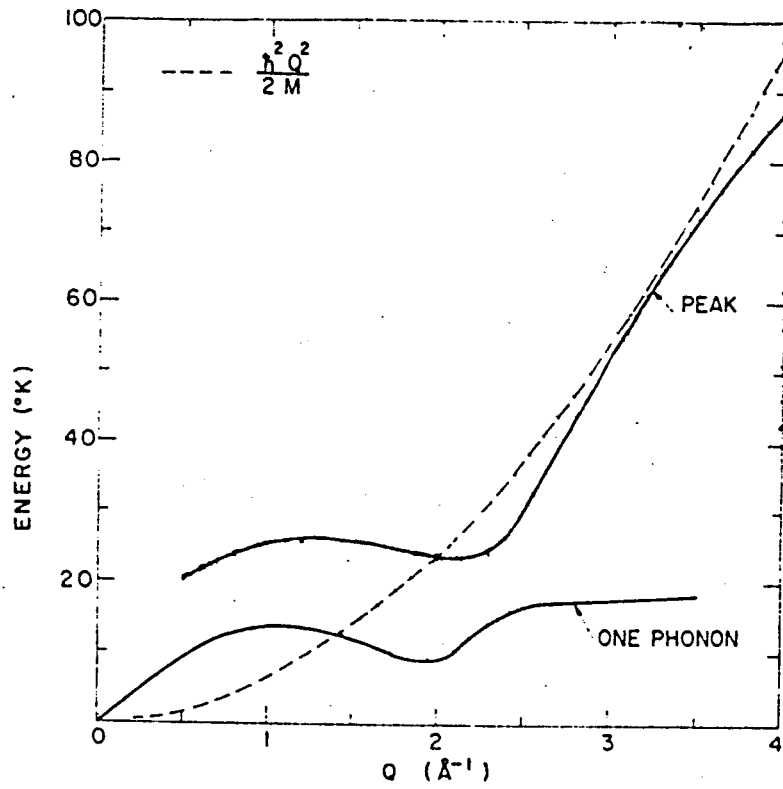
Fig.5 1.1°Kでの液体He 4 の素励起のエネルギースペクトル 35)
