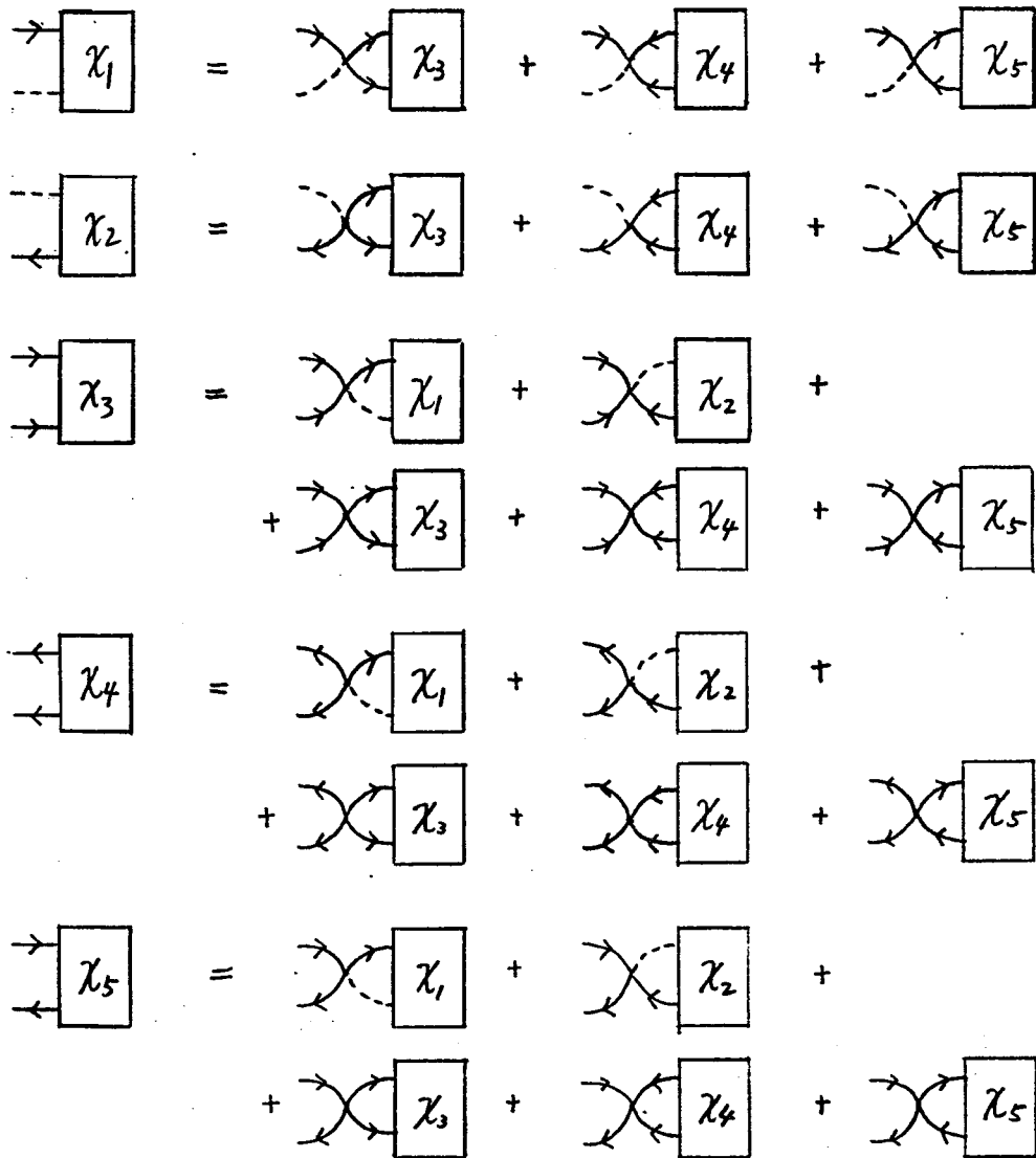
Fig.1 \chi_1(\vec{p}), \chi_2(\vec{p}), \dots, \chi_5(\vec{p}, \omega) の方程式のダイアグラム表現 実線は演算子 a, a^\dagger で表現される個別励起の自由な因果 Green 関数である。
