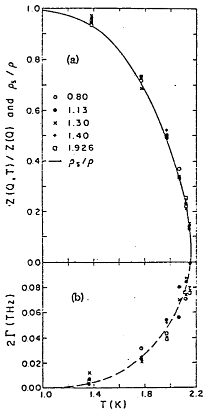
Fig. 11 (a) 超流体成分の \frac{Z(Q, T)}{Z(Q)} と \frac{\rho_s}{\rho} (b) 超流体成分のフォノンピーク のエネルギー P(T)
