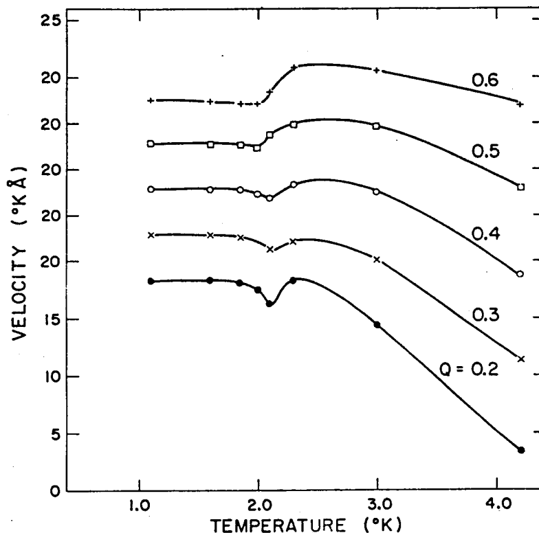
Fig. 7 小さな運動量でのフォノン速度 \omega(\vec{q})/Q の温度依存性 35)
