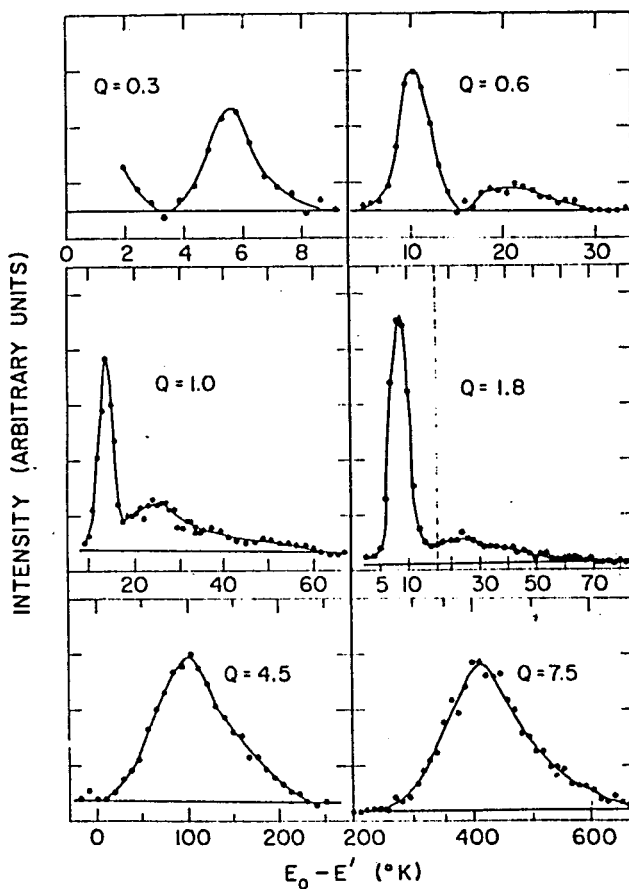
Fig. 4 1.1°K での液体Heの散乱スペクトル 35) E_0, E' は入射および散乱中性子のエネルギー \omega = E_0 - E'
