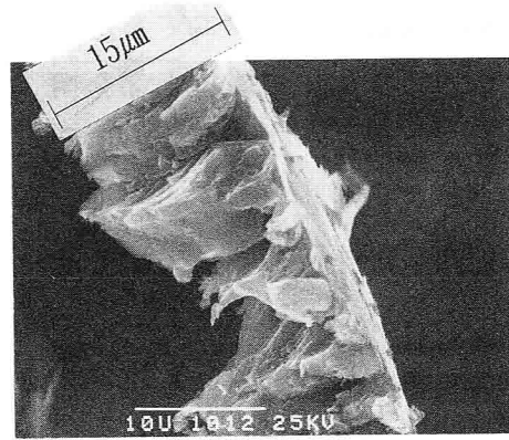
図4-13 切り厚さ 10\mu\text{m} の場合の切りくずのSEM写真
