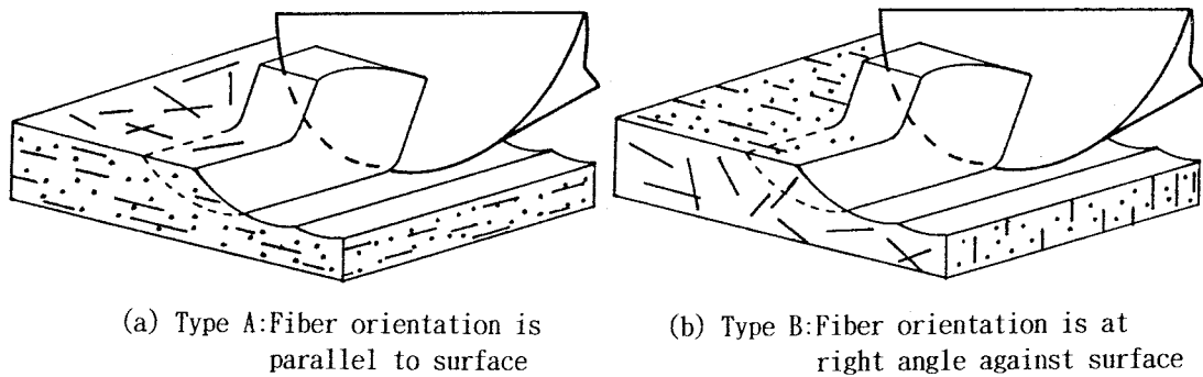
図 3 - 3 0 繊維配向と仕上げ面の関係
