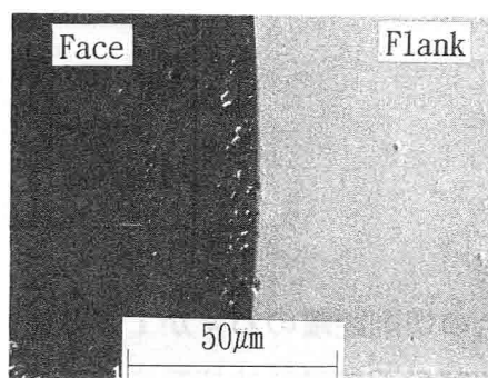
図2-8 A4032ダイヤモンド切削の工具摩耗 超精密旋盤，切削距離：490mm 切削速度：145～393m/min 送り速度：0.01mm/rev 切込み：10μm
