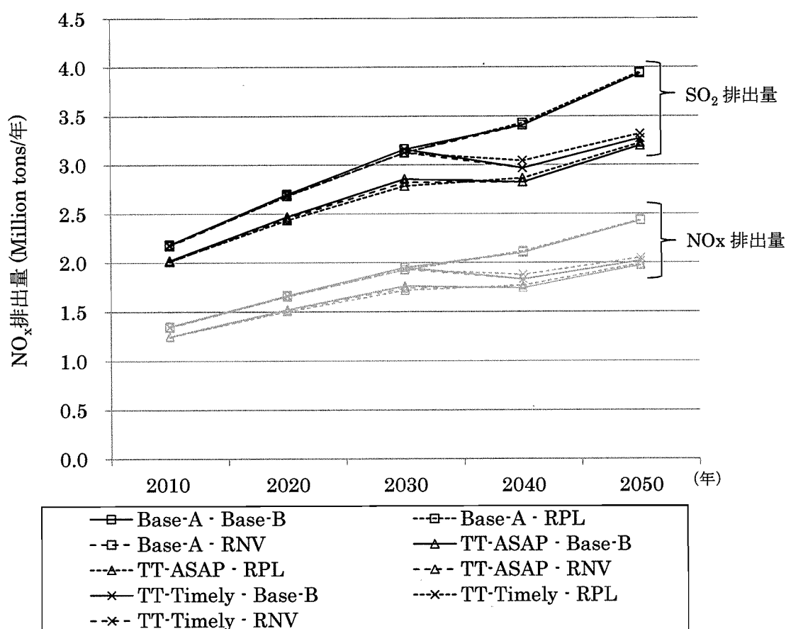
図 3-17 SO 2 , NO x のケース別排出量の推移
