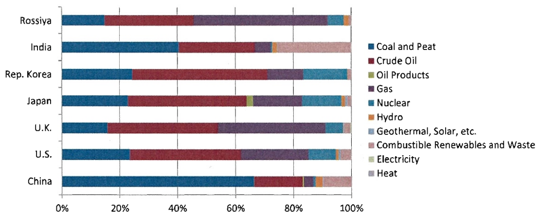
図 2-3 2008 年の主要国のエネルギー消費構造 2 （出典：IEA, 2011）
