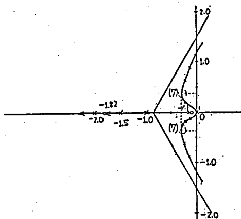
图 4.6 根軌跡 ( \gamma = 0\% , a/b = 0.10 )
