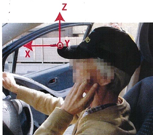
Figure 1 運転者に取り付けたジャイロセンサの計測軸
