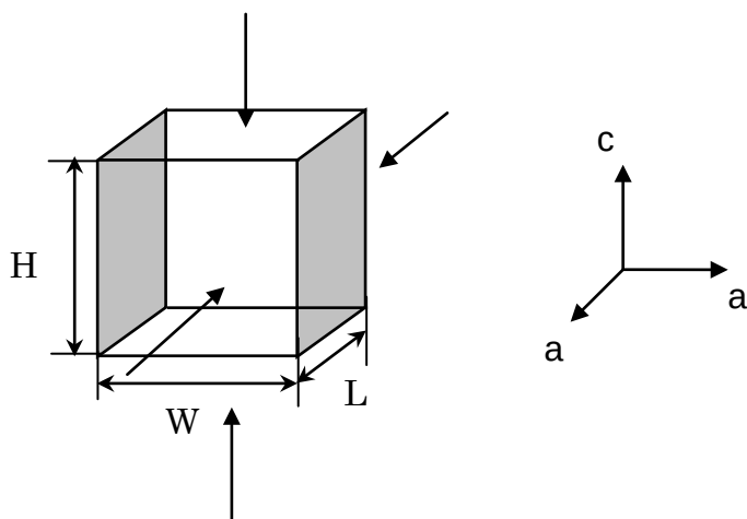
図 2-1 LB4 結晶のカット
