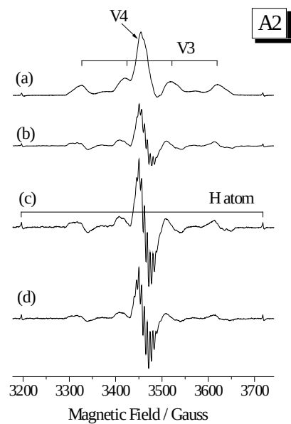
図 2-24 異なる温度で 1 \mu Wのマイクロ波出力で測定した、77 Kで ^{60}\text{Co} からの 1.2 \times 10^4 Gyの線量を照射した試料A2 のEPRスペクトル (a) 4 K, (b) 20 K, (c) 30 K, (d) 50 K.
