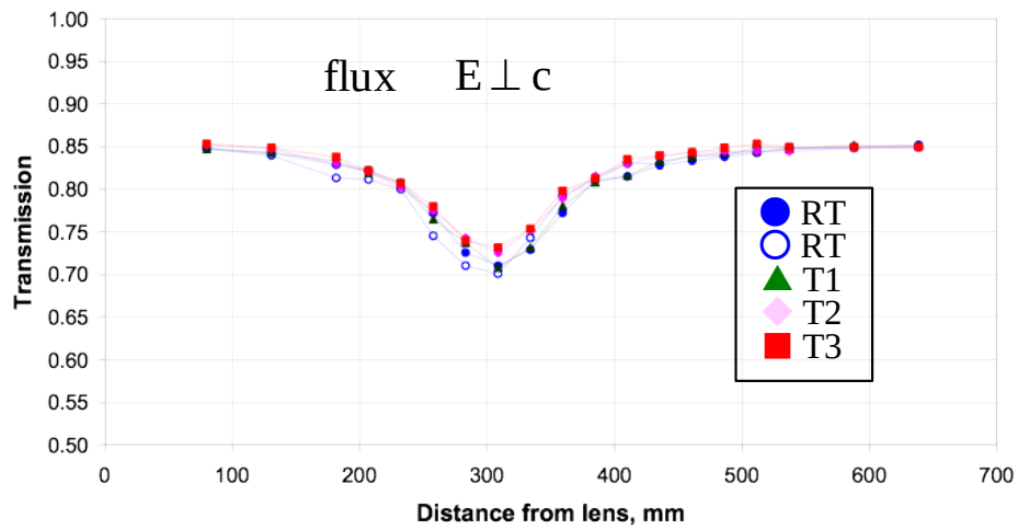
図 3-3 10kHz、4 つの異なる温度における flux-grown BB0 結晶の E \perp c 偏光 (o) 262nmUV の透過率
