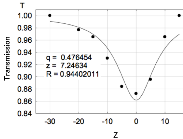
図 2-5 1W のポンプパワーにおける Z-scan データのフィッティング結果
