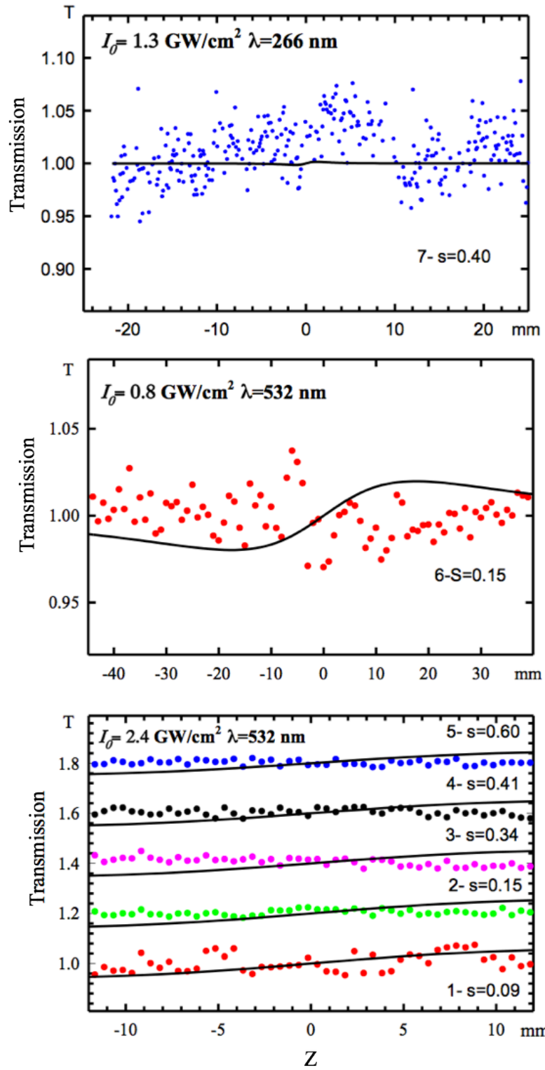
図 2-8 LB4 結晶の 266nm と 532nm 励起での Z-scan 測定
