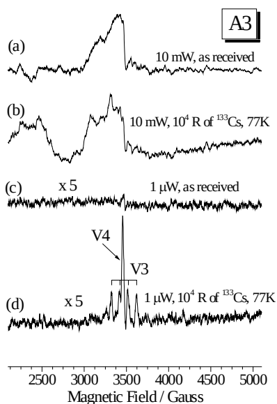
図 2-22 4 K で異なるマイクロ波出力で測定した、77 K で ^{137}\text{Cs} からの 10^2 Gy の線量を照射した試料 A3 の EPR スペクトル (a) 10 mW のマイクロ波出力でのバックグラウンド、(b) \gamma 線照射、10 mW、(c) 1 \mu W のマイクロ波出力でのバックグラウンド、(d) \gamma 線照射、10 mW
