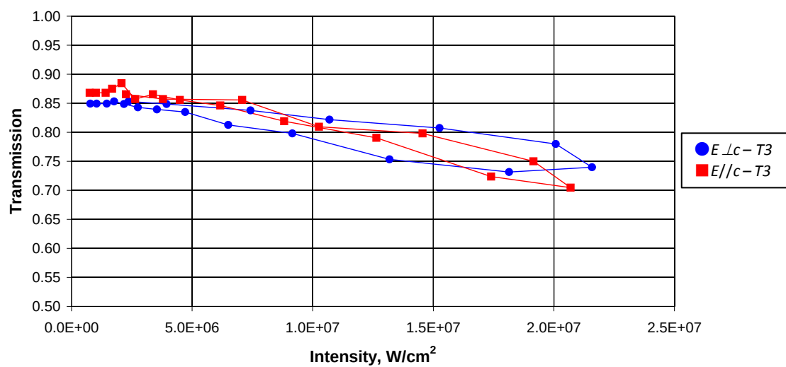
図 3-12 10kHz、151℃における E \perp c 偏光及び E // c 偏光の flux-grown BBO 結晶の 262nm 透過率とピークパワー密度との関係
