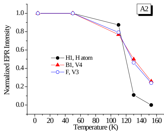
図 2-26 77K で ^{60}\text{Co} 線源からの 1.2 \times 10^4 Gy の \gamma 線照射後の EPR センター信号の温度依存性
