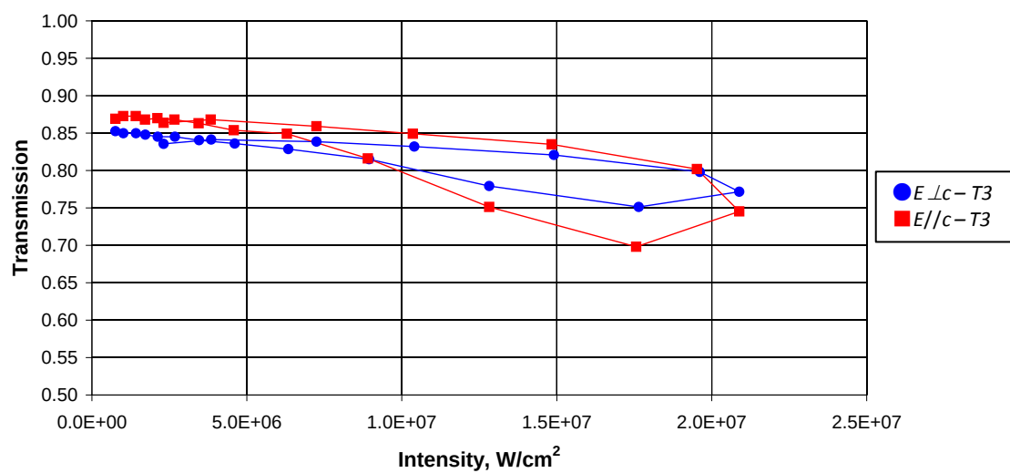
図 3-14 10kHz、51 °Cにおける E \perp c 偏光及び E // c 偏光の flux-grown BBO 結晶の 262nm
