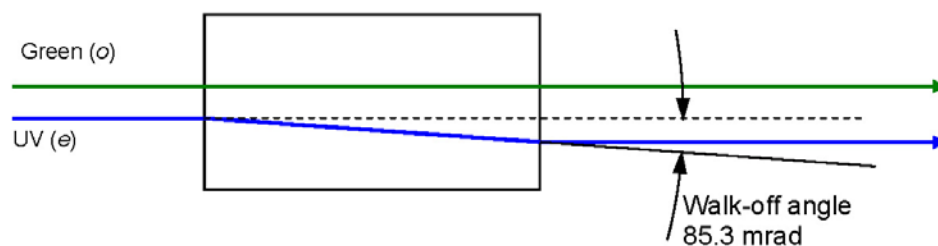
図3-35 BB0結晶中での通常光線(green)と異常光(262nm)のビーム伝播の関係
