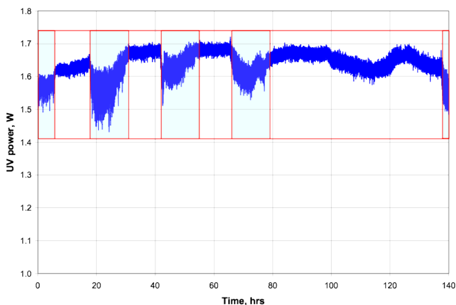
図3-30 結晶長8mmのflux-grown BB0結晶での262nm出力(~1.6 W)の経時安定性(安定性評価
