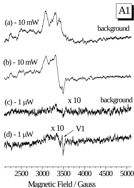
図 2-18 4K で異なるマイクロ波出力(10mW(a, b), 1\mu\text{W} (c, d))で測定した EPR のバックグラウンドスペクトル(a, c)と \gamma 線照射を行っていない試料 A1 の信号(b, d)
