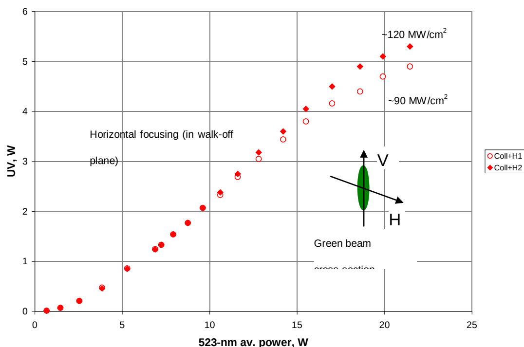
図3-26 CZ-grown BB0結晶における入力Greenと262nmの出力との関係(実験3)
