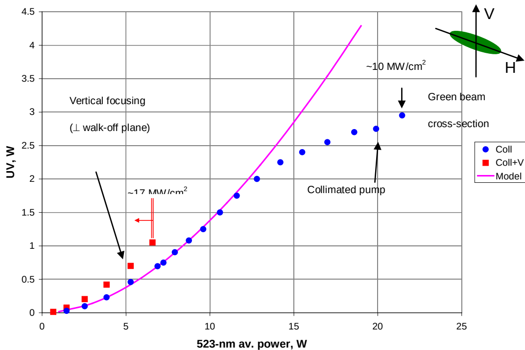
図3-23 CZ-grown BBO結晶における入力Greenと 262\text{nm} の出力との関係(実験1及び実験2)
