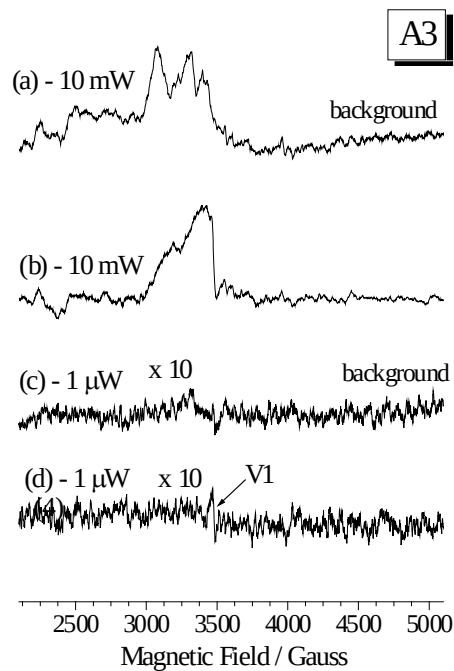
図 2-19 4K で異なるマイクロ波出力(10mW(a, b), 1\ \mu\text{W} (c, d))で測定した EPR のバックグラウンドスペクトル(a, c)と \gamma 線照射を行っていない試料 A3 の信号(b, d)
