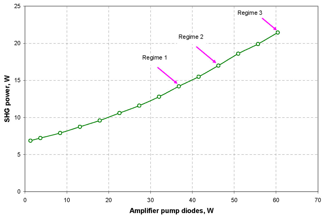
図3-18 SHG (Green) 平均出力とアンプリファイアーの励起ダイオードレーザの出力の関係
