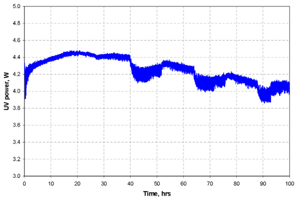
図3-29 結晶長8mmのCZ-grown BB0結晶での262nm出力(～4.4W)の経時安定性(安定性評価3)
