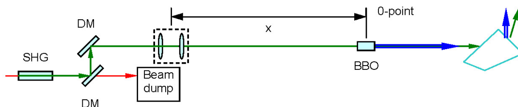
図3-21 第四高調波発生の実験レイアウト
