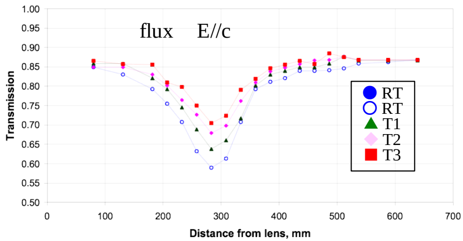
図 3-4 10kHz、4 つの異なる温度における flux-grown BB0 結晶の E // c 偏光 (e) 262nmUV の透過率
