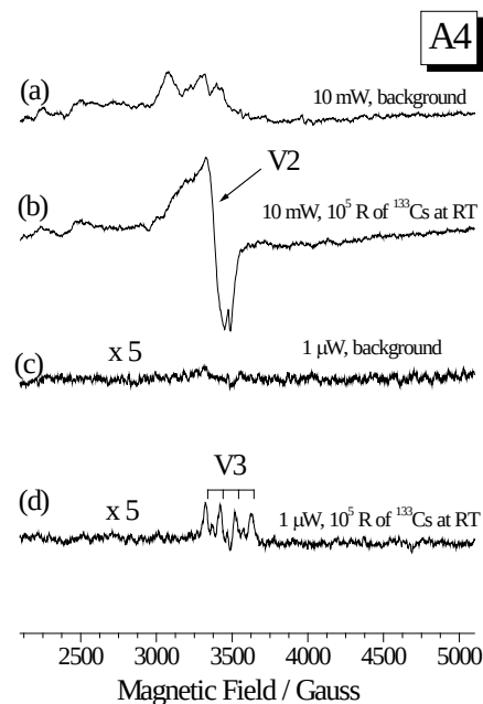
図 2-20 4Kで異なるマイクロ波出力(10mW(a, b), 1\ \mu\text{W} (c, d))で測定したEPRのバックグラウンドスペクトル(a, c)と室温で ^{137}\text{Cs} 線源から 10^3\ \text{Gy} の \gamma 線を照射した試料A3 の信号(b, d)
