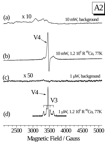
図 2-23 4 K で異なるマイクロ波出力で測定した、77 Kで ^{60}\text{Co} からの 1.2 \times 10^4 Gyの線量を照射した試料A2 のEPRスペクトル (a) 10 mWのマイクロ波出力でのバックグラウンド, (b) \gamma 線照射、10 mW, (c) 1 \mu Wのマイクロ波出力でのバックグラウンド, (d) \gamma 線照射、10 mW
