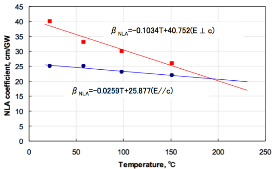
図 3-15 E \perp c 偏光及び E // c 偏光の flux-grown BBO 結晶の 10kHz、262nm における温度と NLA との関係
