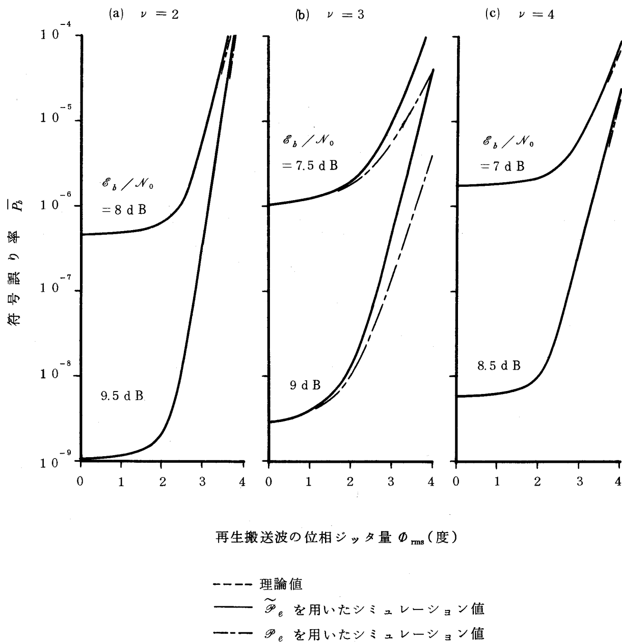
図 6.8 再生搬送波の位相ジッタ量 \phi_{\text{rms}} に対する符号誤り率
