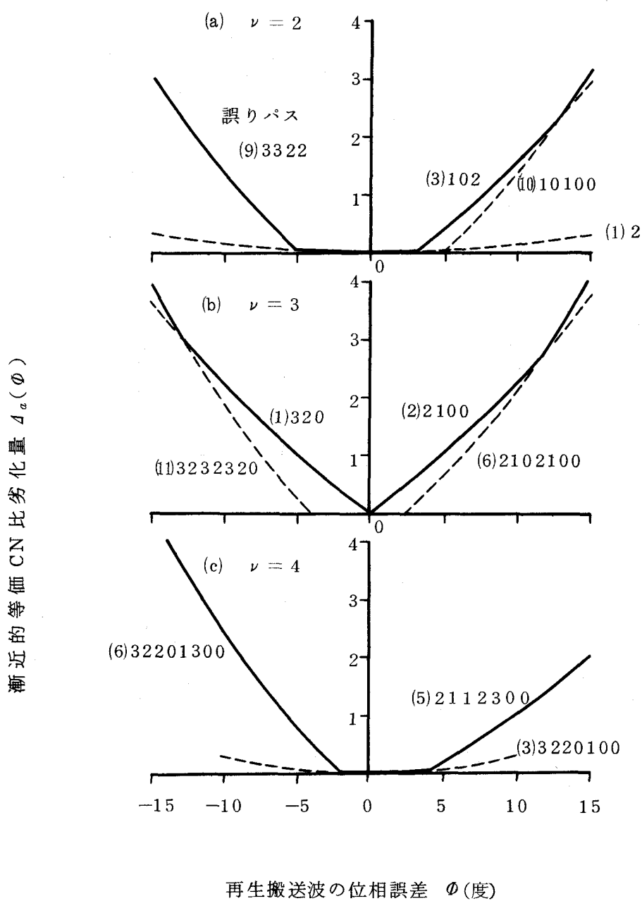
図 6.11 再生搬送波の位相誤差 \phi に対する漸近的等価 CN 比劣化量 A_e(\phi)
