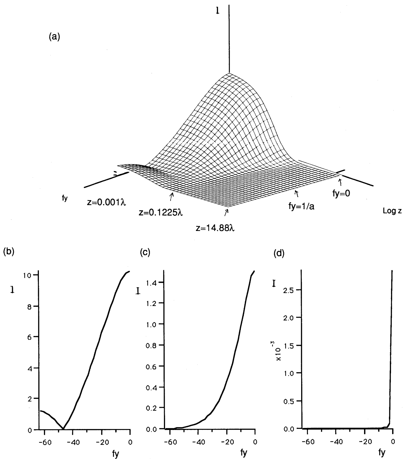
図 3-13 Betheの理論で計算した円形開口による回折場の磁場のAngular Spectrum (垂直入射、 開口半径 a: \lambda / 100 、 \Delta f = 125 / 16 \lambda 、 z = \text{Exp}[(j-1) \cdot 0.3 - 6.9] ) . (a) y z 面での振幅分布のAngular Spectrumの変化. (b) z = 0.001 \lambda での y 軸上のAngular Spectrum. (c) z = 0.1225 \lambda での y 軸上のAngular Spectrum. (d) z = 14.88 \lambda での y 軸上のAngular Spectrum.
