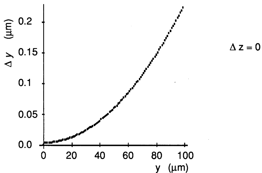
図 5-9 収差の計算結果.
