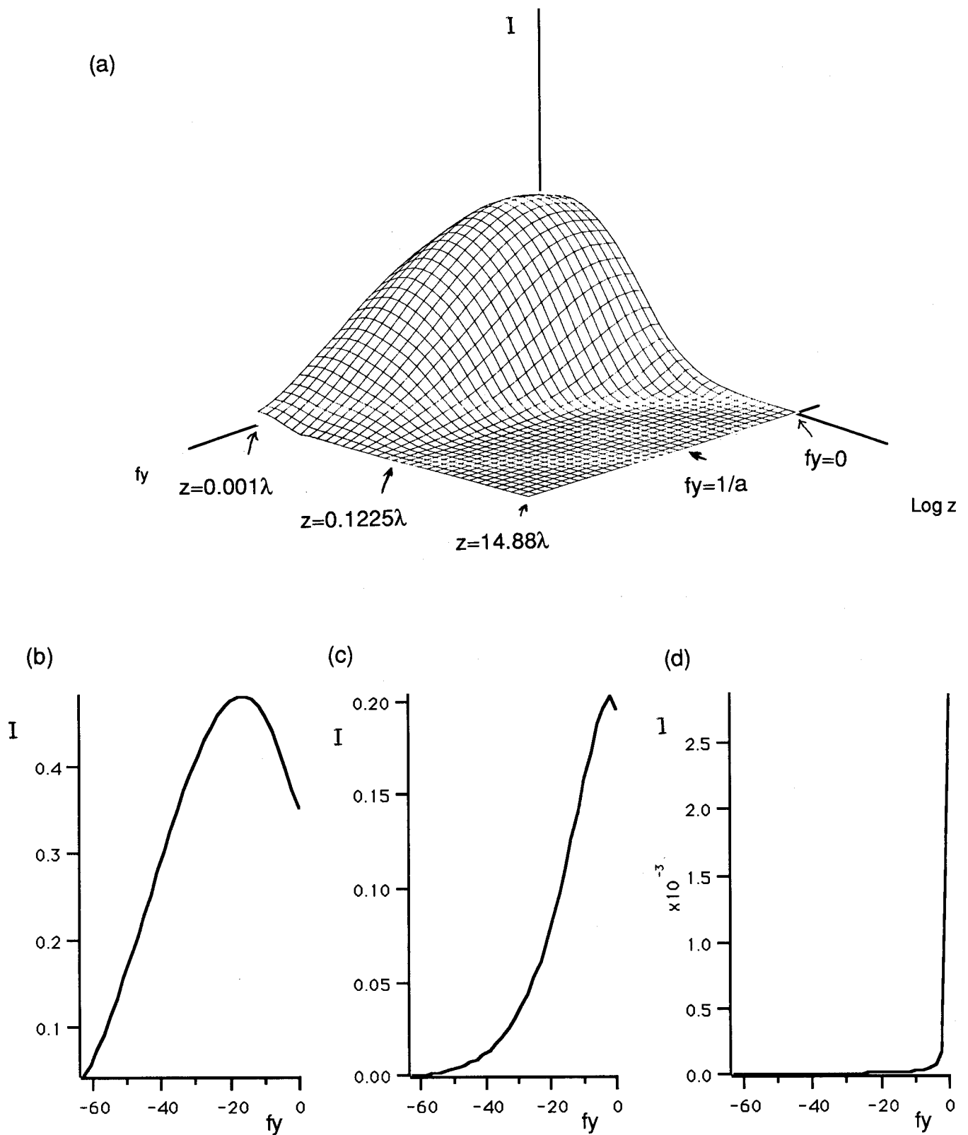
図 3-10 Betheの理論で計算した円形開口による回折場の電場のAngular Spectrum (垂直入射、 開口半径 a: \lambda / 100 、 \Delta f = 125 / 16 \lambda 、 z = \text{Exp}[(j-1) \cdot 0.3-6.9] ) . (a) y z 面での振幅分布のAngular Spectrumの変化. (b) z = 0.001 \lambda での y 軸上のAngular Spectrum. (c) z = 0.1225 \lambda での y 軸上のAngular Spectrum. (d) z = 14.88 \lambda での y 軸上のAngular Spectrum.
