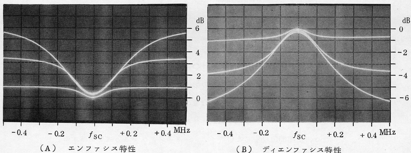
図 3.38 ダイナミックディエンファシス特性 (入力 0, -10, -20dB)
