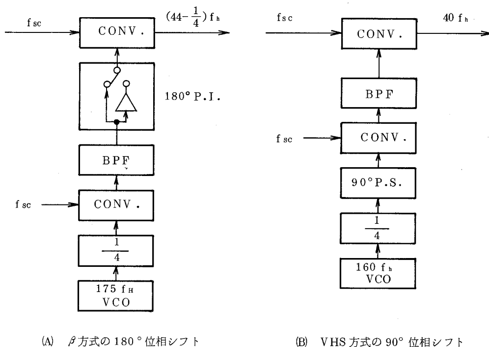
図3.43 従来の周波数変換回路
