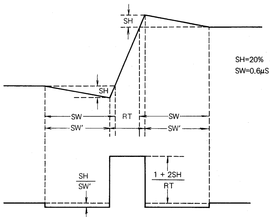
図 2.12 インパルス応答
