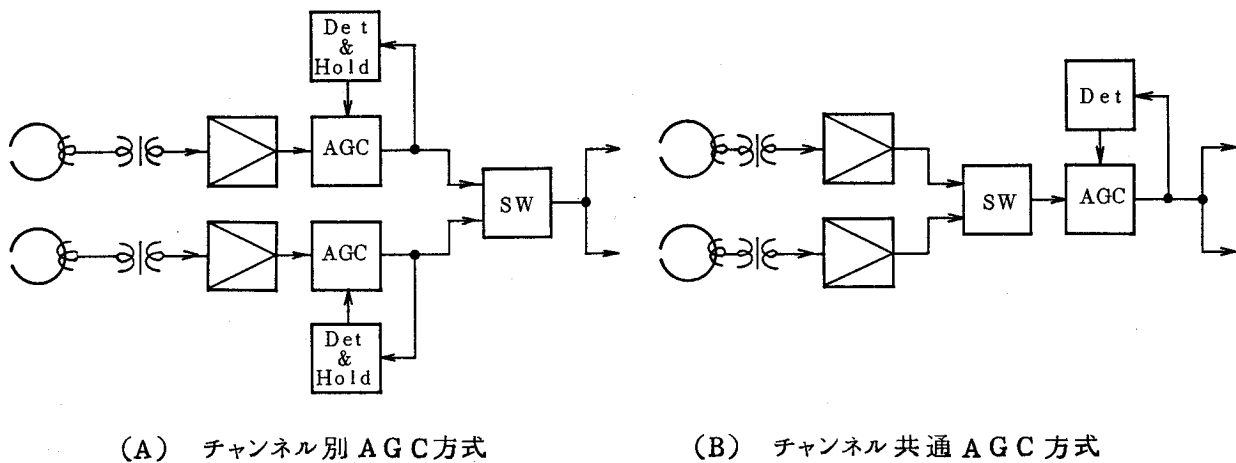
図3.11 FM信号用AGC回路
