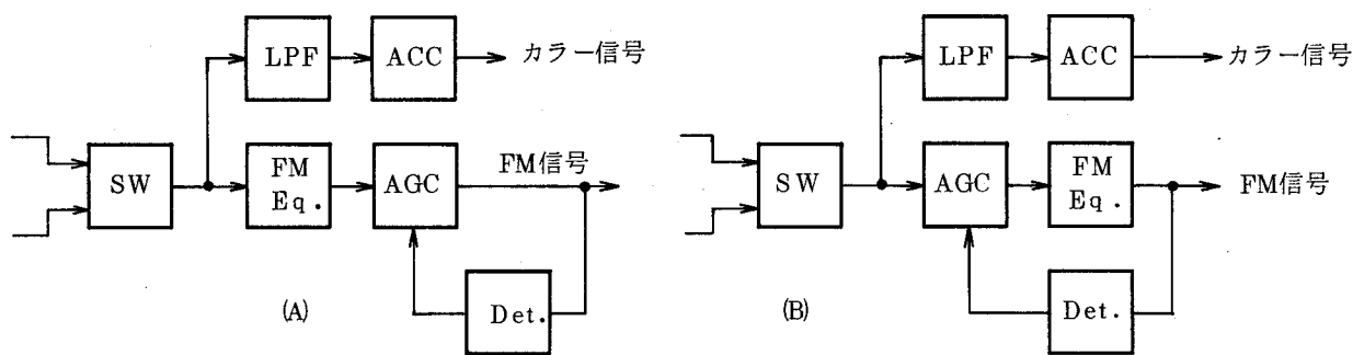
図 3.20 再生等化回路 (FMEq.) の配置
