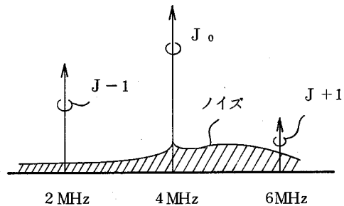
図3.7 再生FM信号のS/N
