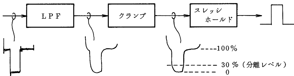
図3.26 同期分離回路
