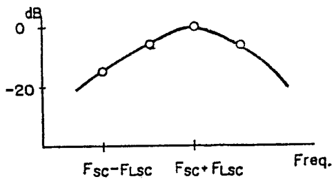
(B) 8ミリビデオ180° 位相シフト用
