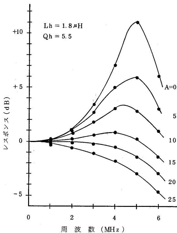
図3.17 フィードバックダンピング特性
