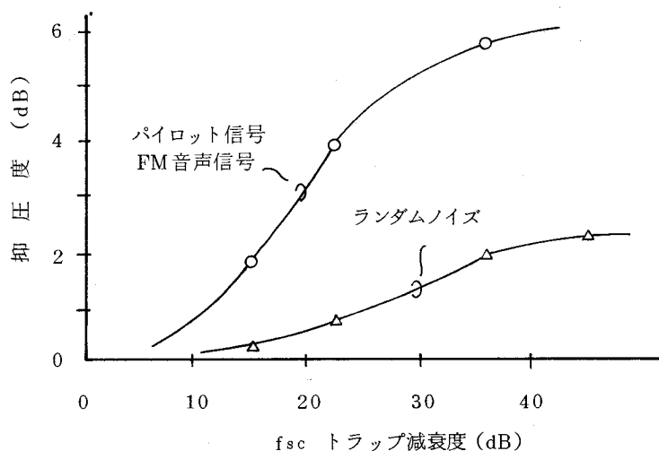
図3.42 ディエンファシス回路の効果
