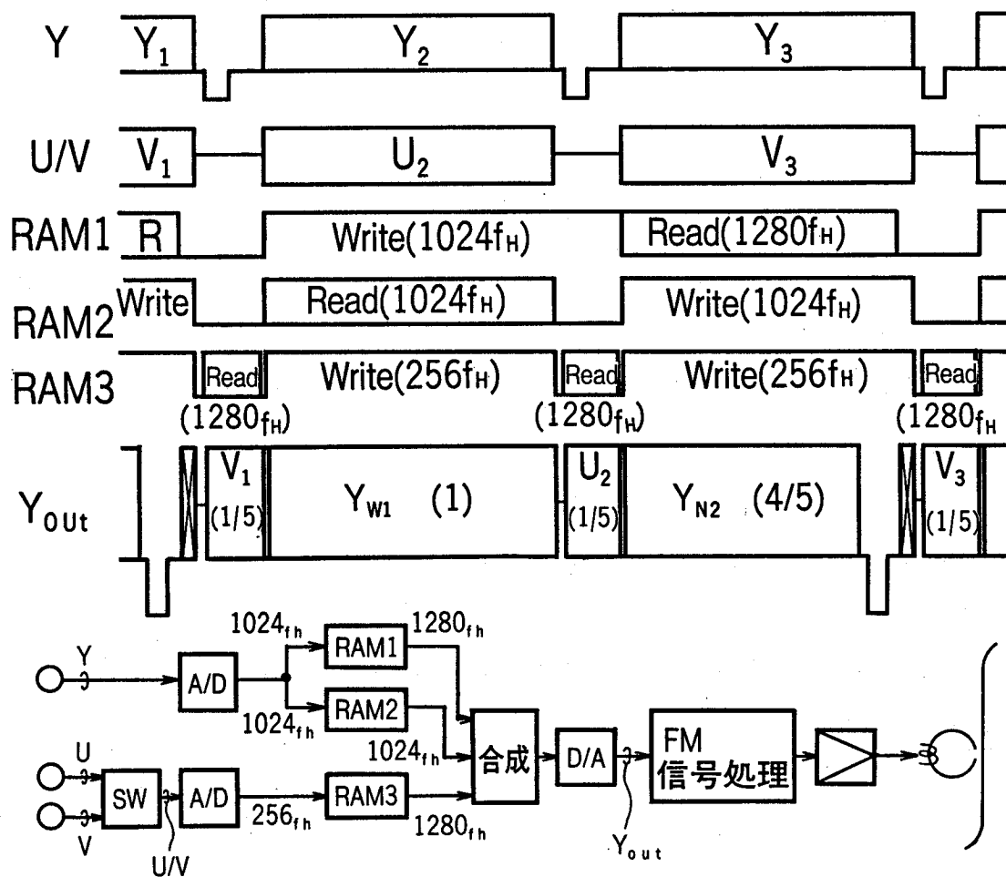
図 3.50 新時分割多重方式の概要
