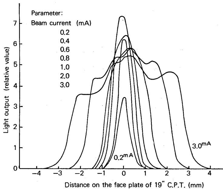
図 2.3 電子ビームの密度分布
