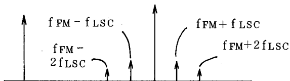
(B) AGC 出力スペクトル
