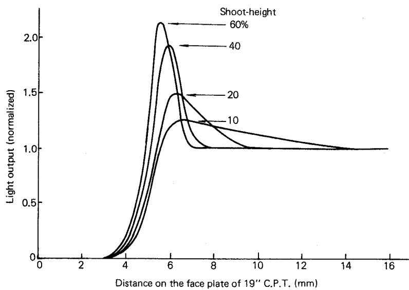
(B) 輝度分布 ( I_b = 0.2 \text{ mA} )
