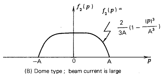
図 2.5 輝度分布の近似
