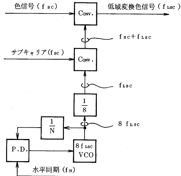
図 3.35 色信号周波数変換回路の基本構成
