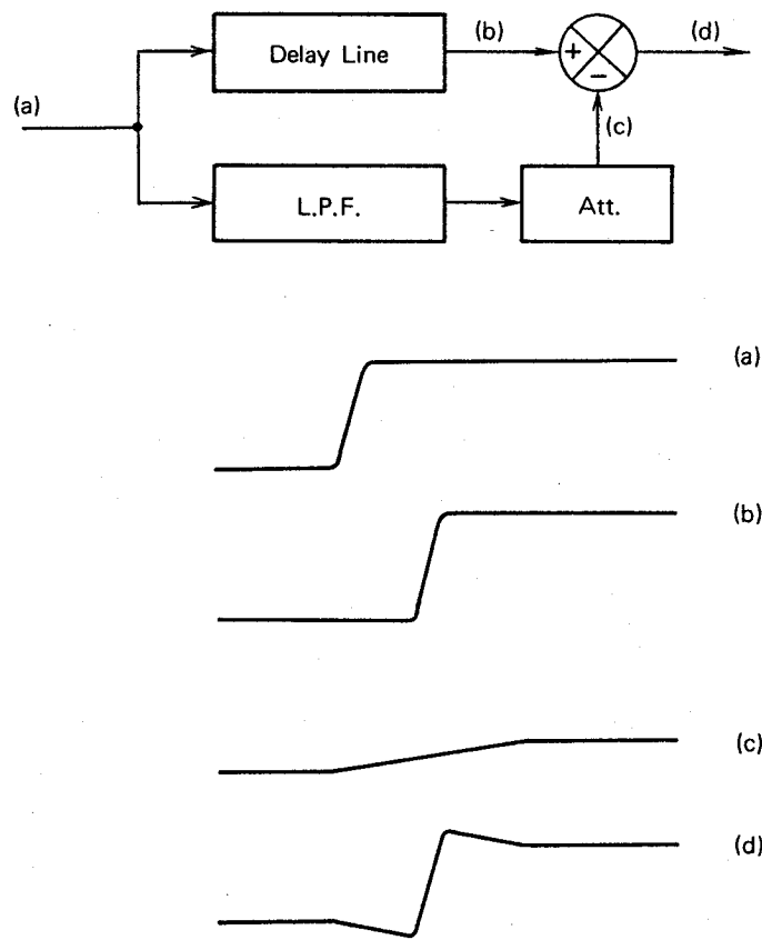
図2.14 鮮鋭度補償回路
