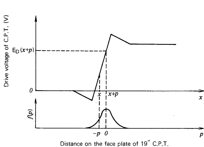
図 2.4 畳み込み積分
