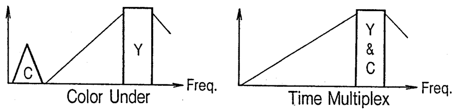
図 3.48 記録帯域幅の比較
