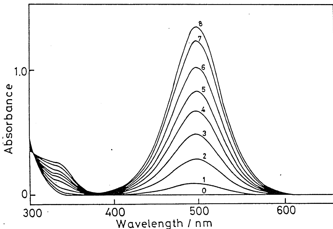
Figure 4-1. Absorption spectra of 18E -Et 2 NH system in benzene. [18E]= 3.4 \times 10^{-5} mol dm -3 , 0: [Et 2 NH]=0 mol dm -3 ; 1: [Et 2 NH]= 3.4 \times 10^{-2} mol dm -3 ; 2: [Et 2 NH]= 6.8 \times 10^{-2} mol dm -3 ; 3: [Et 2 NH]= 1.0 \times 10^{-1} mol dm -3 ; 4: [Et 2 NH]= 1.4 \times 10^{-1} mol dm -3 ; 5: [Et 2 NH]= 1.7 \times 10^{-1} mol dm -3 ; 6: [Et 2 NH]= 2.4 \times 10^{-1} mol dm -3 ; 7: [Et 2 NH]= 3.4 \times 10^{-1} mol dm -3 ; 8: [Et 2 NH]= 5.1 \times 10^{-1} mol dm -3 .
