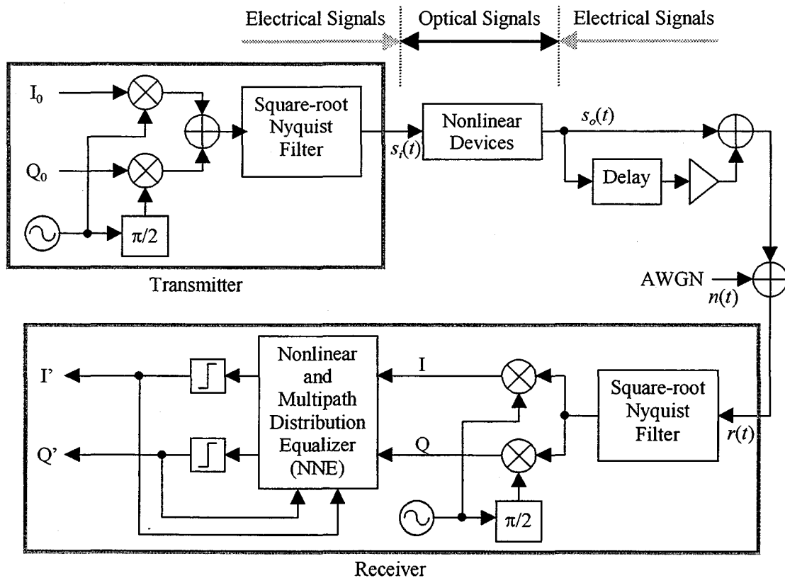
図 2-2-2 等価低域系での FTTA システム・モデル
