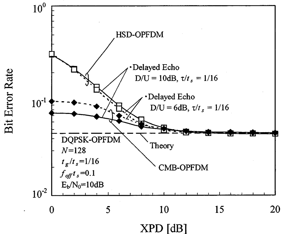
図3-5-1 XPD-BER特性
