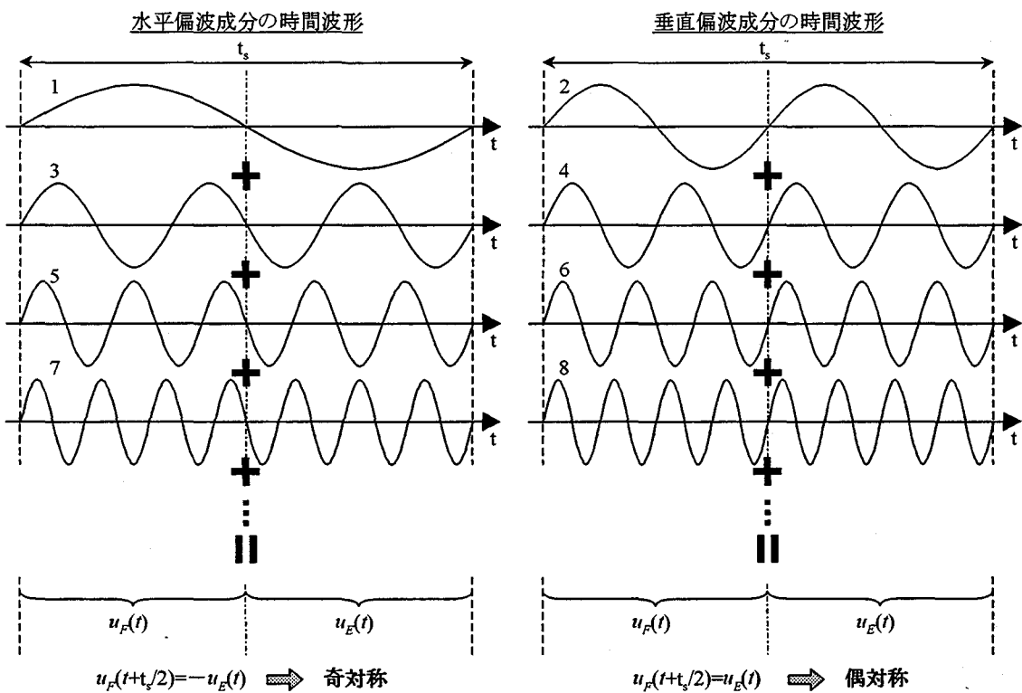
図 1-1-5 OPFDM の特徴
