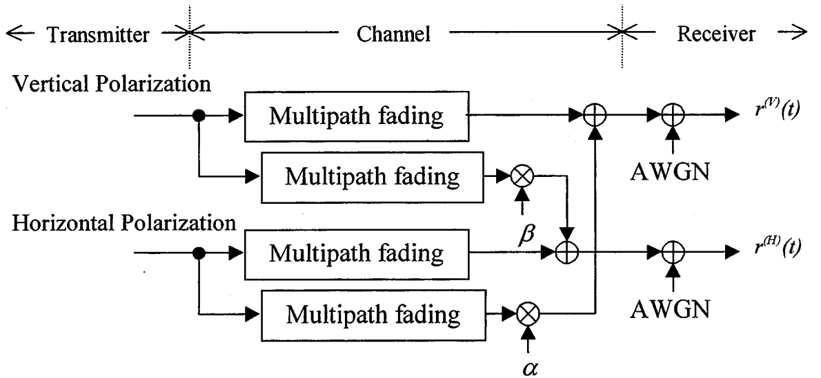
図 3-4-1 伝送路モデル
