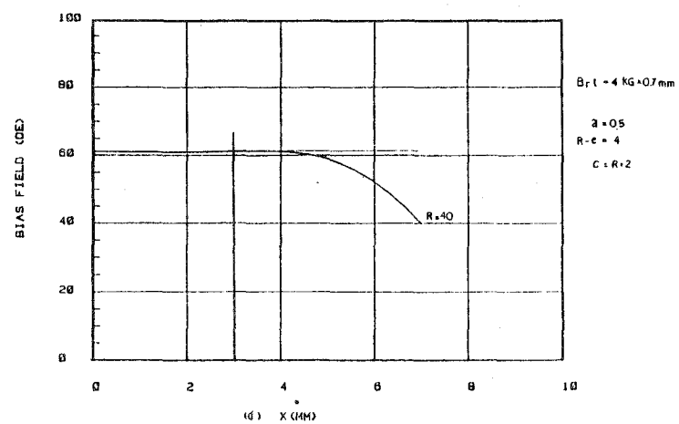
第6-17図 各条件における半円弧状永久磁石からの磁界分布
