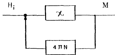
第6-21図 磁性体の磁化に伴うフィードバック・ループ
