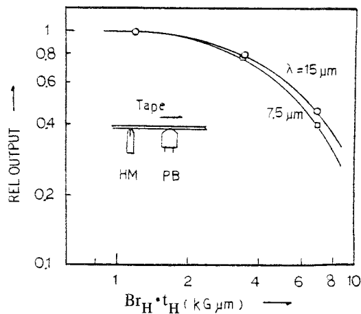
第 6 - 14 図 硬磁性膜の B_H \cdot t_H と磁化媒体信号の消磁 \gamma\text{-Fe}_2\text{O}_3 テープの実測値 (相対比較)
