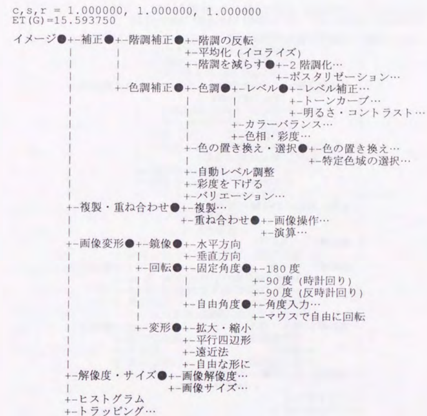
図 2.8: seed 階層構造
