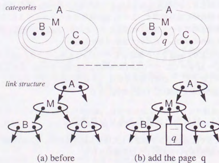
図 3.6: ページの追加
