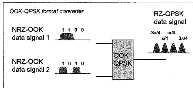
Fig. 4.1: Illustration of OOK to QPSK converter.
