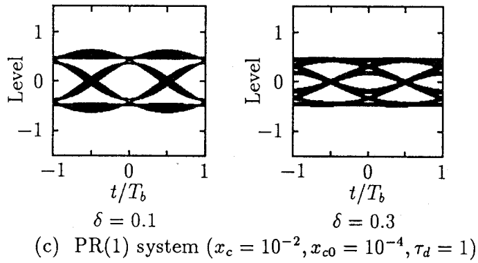
図 2.11 スペース増大の影響を受けたアイパターン ( \beta = 0.5 , \eta = 1 )
