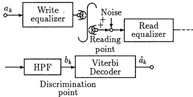
図 5.13 記録・再生等化に対するビタビ復号器を備えた記録再生系ブロック図
