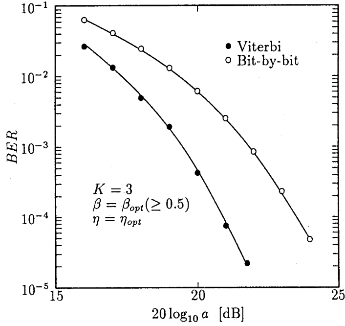
図 5.6 誤り率特性
