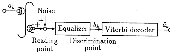
図 5.1 ビタビ復号器を備えた I 方式の記録・再生系ブロック図
