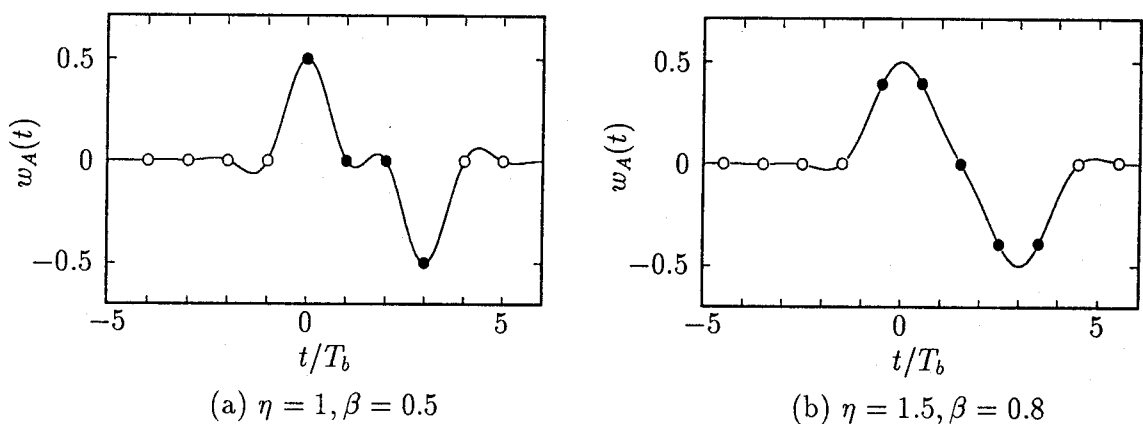
図 2.14 PR(1, 0^{m-1} , -1) 方式の再生等化器出力波形 ( m = 3 )
