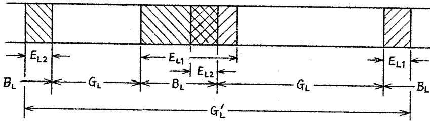
図 2 . 6 B_L \leq E_{L1} の場合
