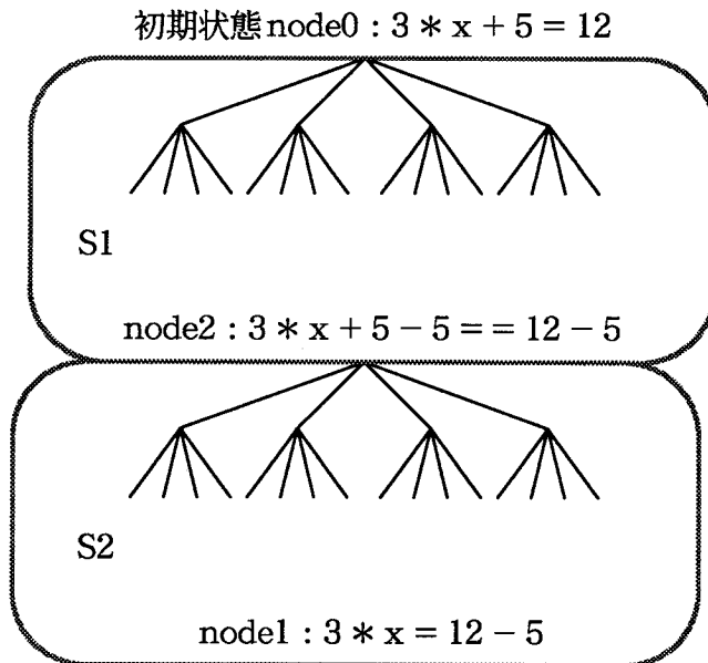
Fig.3.7 解法例の入力
