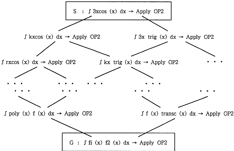
Fig.2.3 バージョン空間
