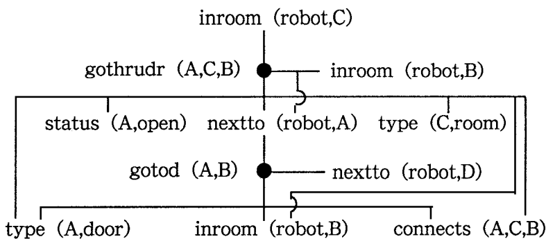
Fig.5.7 一般化された説明木
