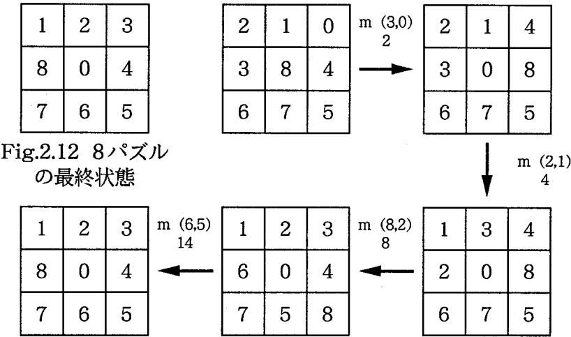
Fig.2.13 マクロによる問題解決
