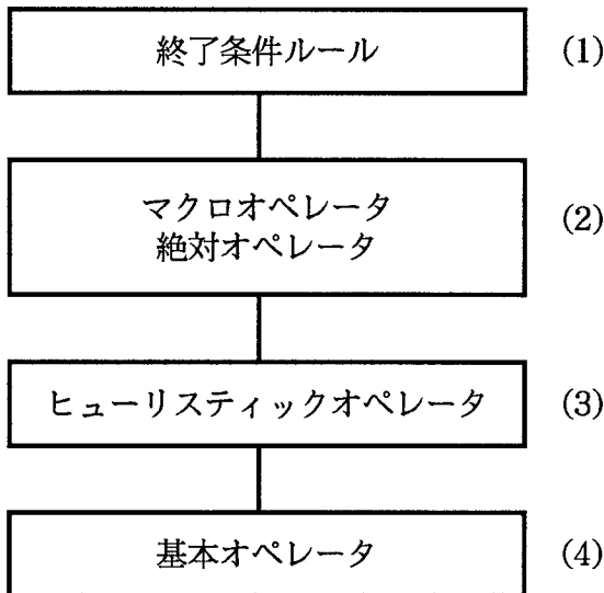
Fig.3.6 オペレータの階層
