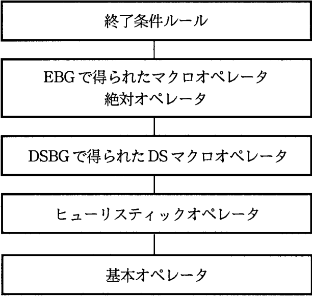
Fig.4.6 知識ベースの階層構造
