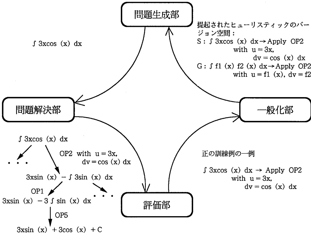
Fig.2.2 LEXの学習サイクル
