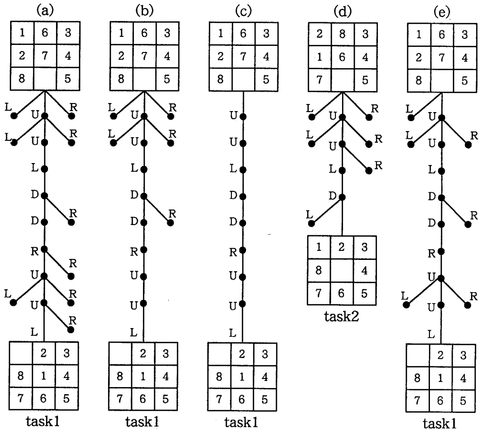
Fig.2.11 Soarでの8パズルの学習
