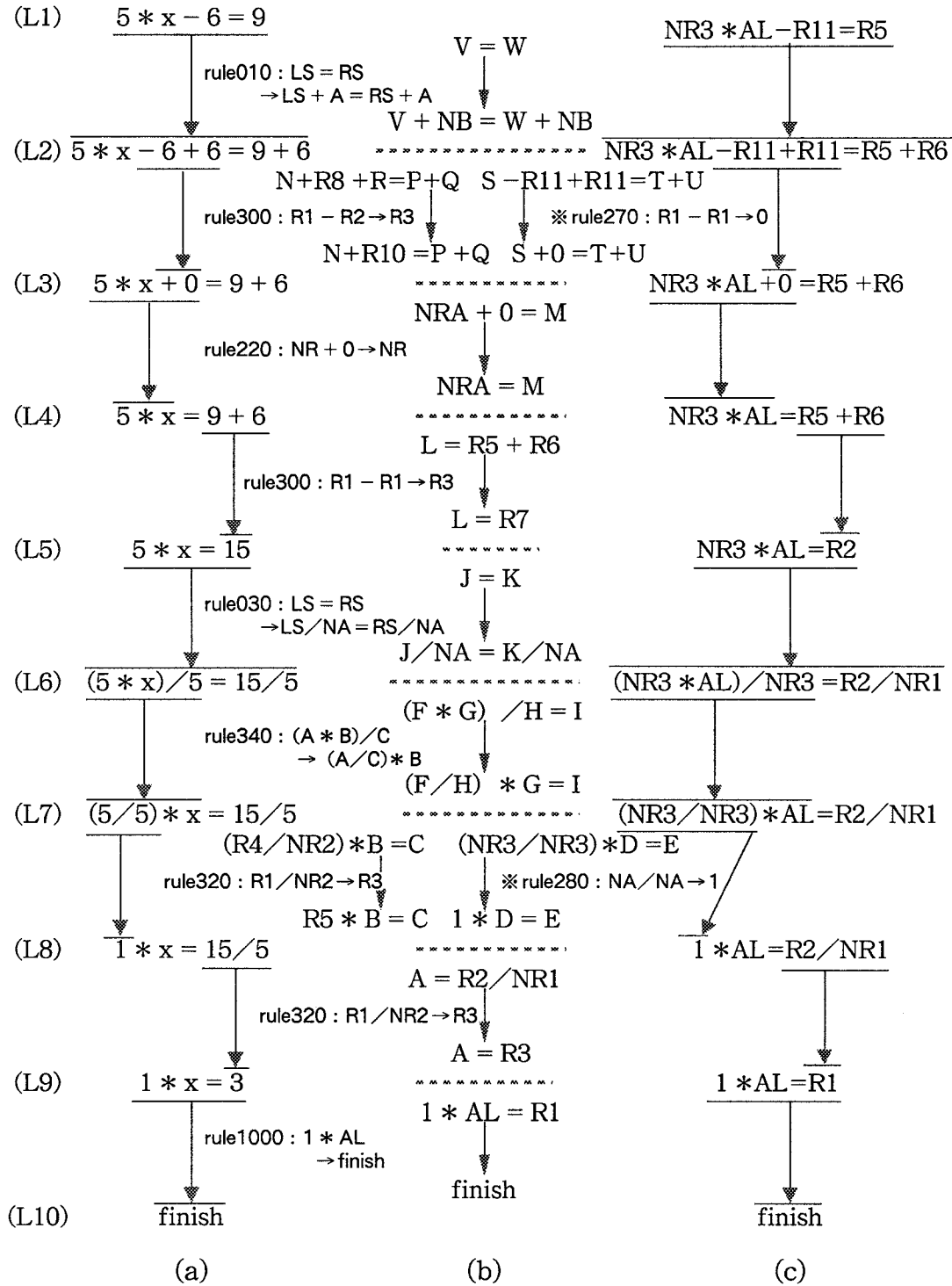
Fig.3.10 一般化の具体的処理過程
