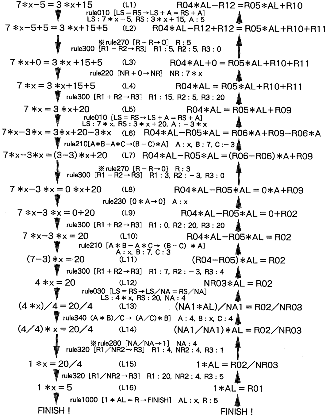
Fig.3.8 解法例
