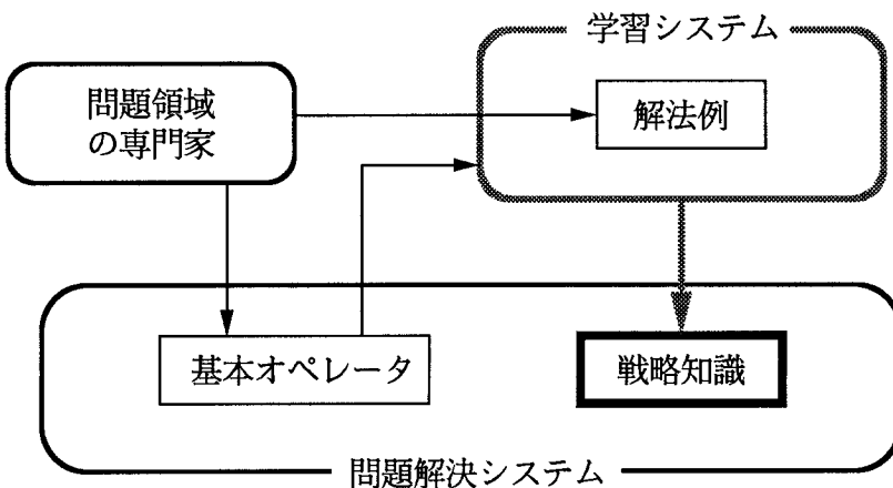
Fig.3.1 戦略知識の獲得
