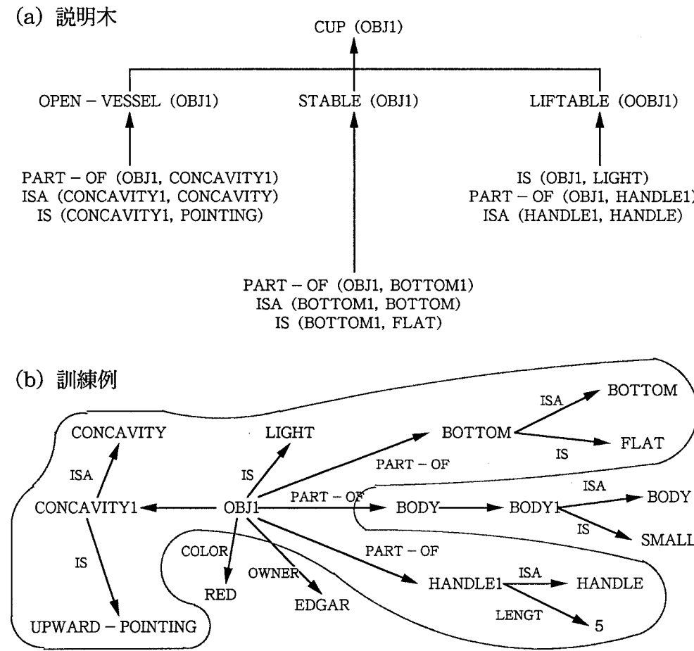
Fig.2.6 CUP の説明木と訓練例
