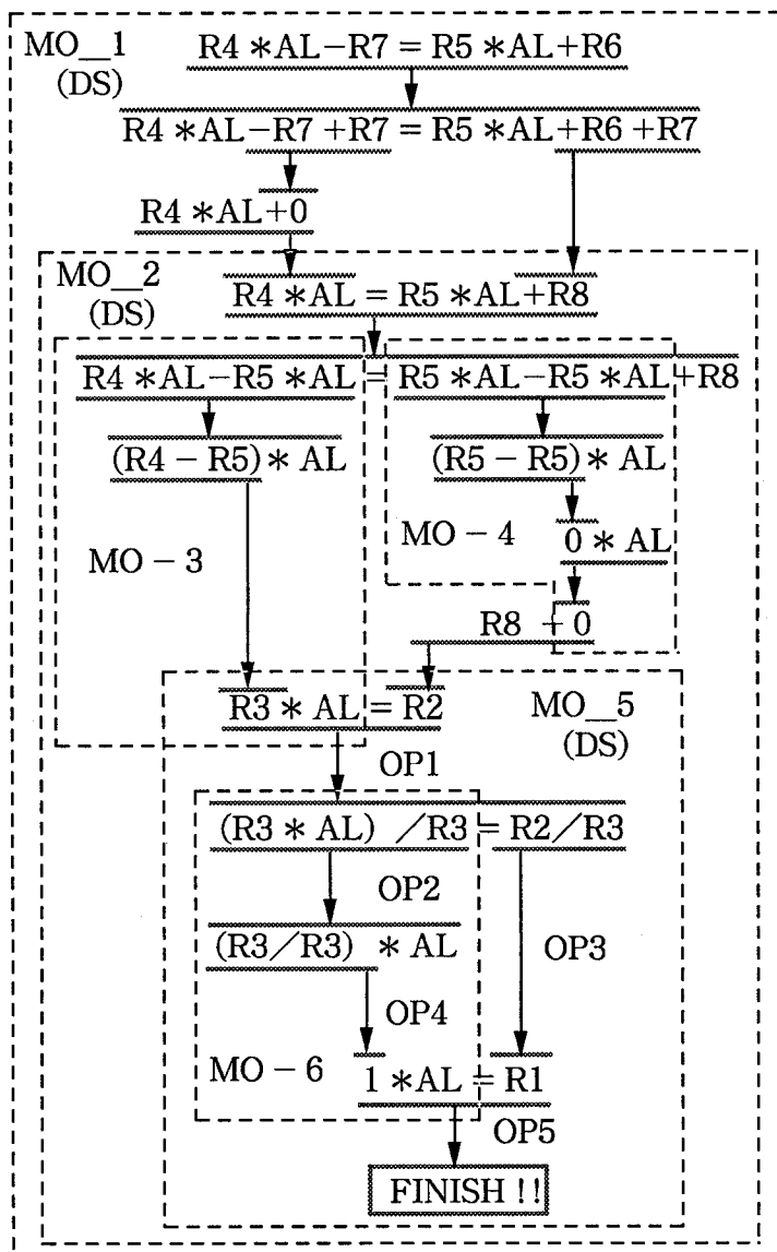
Fig.3.15 マクロオペレータの抽出
