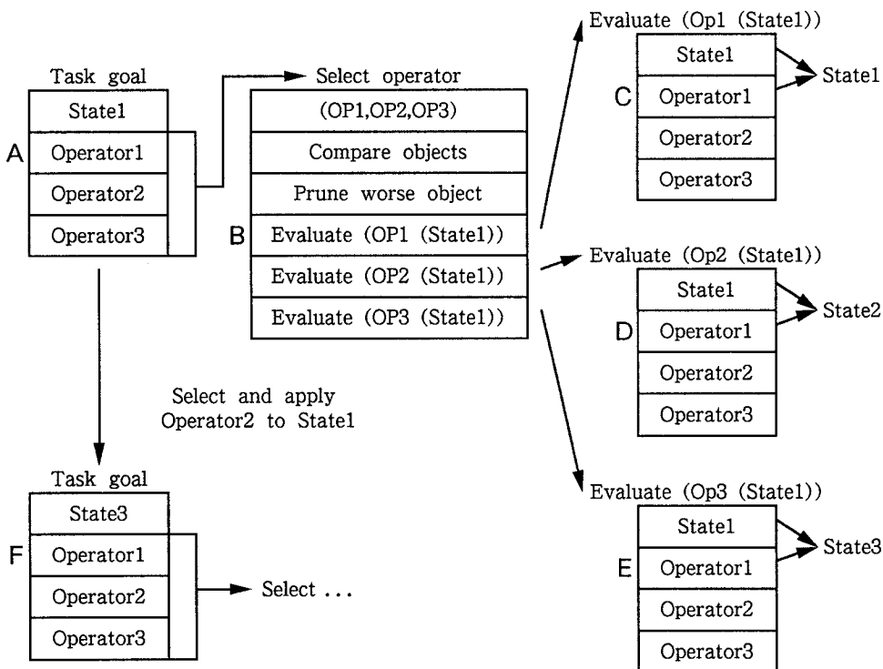
Fig.2.10 Soar でのサブゴール構造
