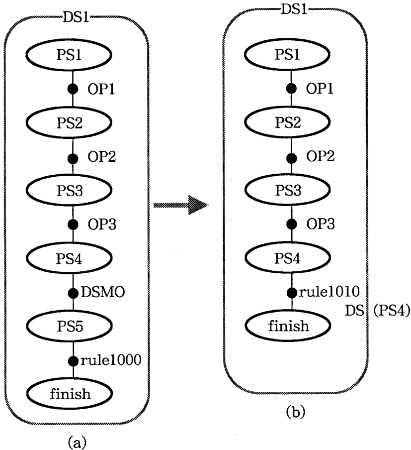
Fig.4.3 解法例(説明木)の変化
