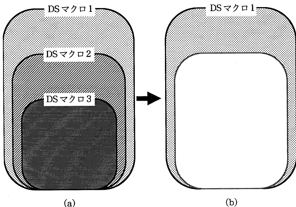
Fig.4.9 複数の DS マクロが包含される場合
