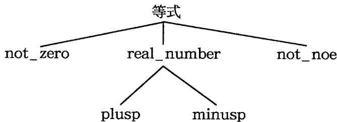
Fig.3.5 概念述語のハイアラーキ
