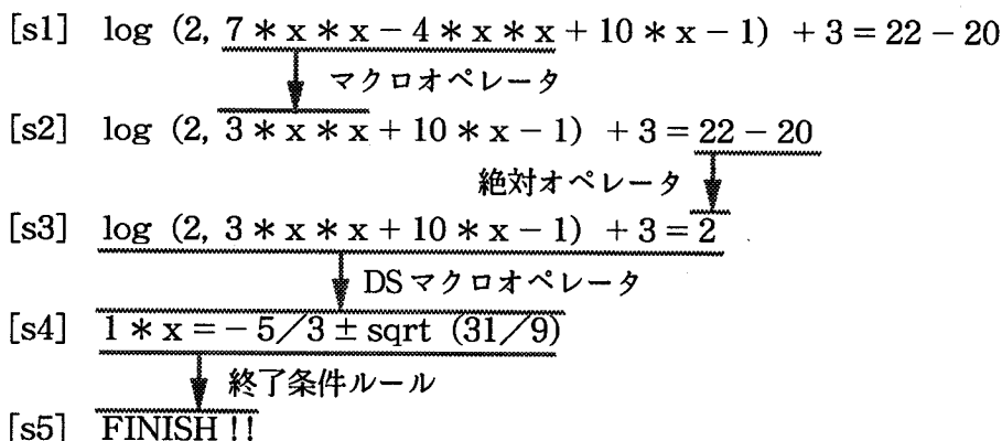
Fig.3.18 学習後のPiLの問題解決 (対数方程式)
