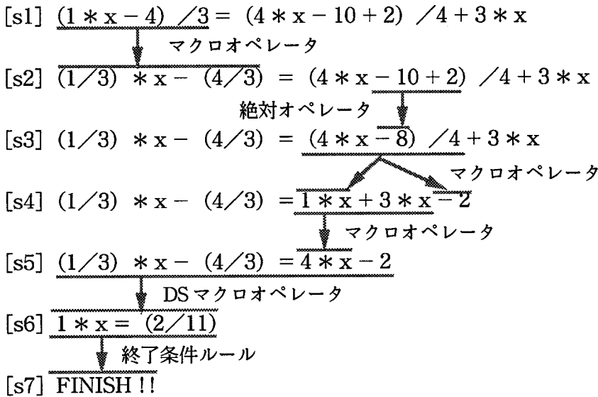
Fig.3.17 学習後のPiLの問題解決 (1次方程式)
