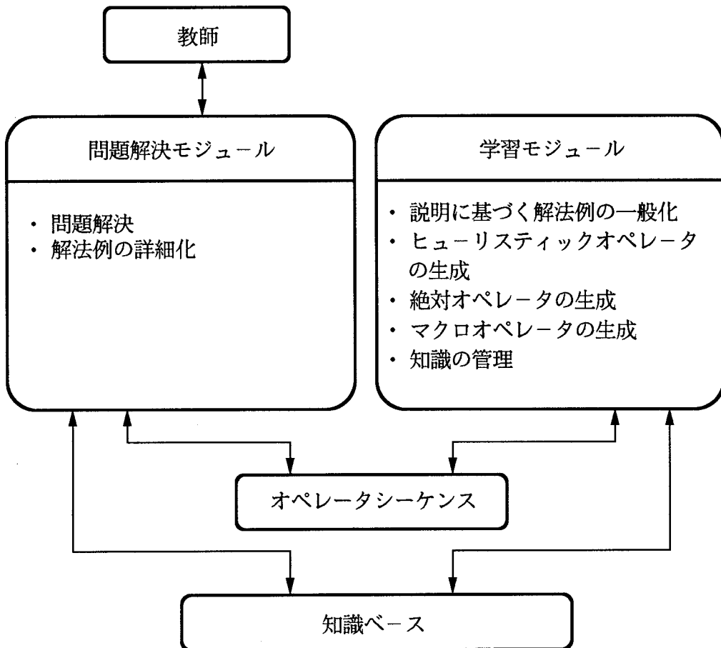
Fig.3.2 PiLのシステム構成
