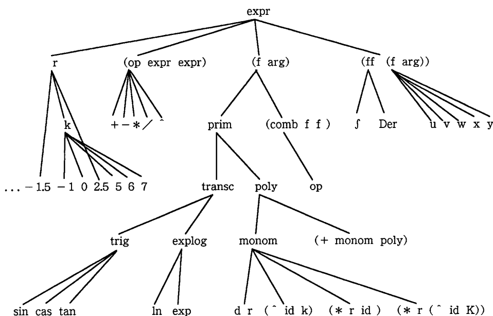
Fig.2.5. LEXでの概念記述言語の文法
