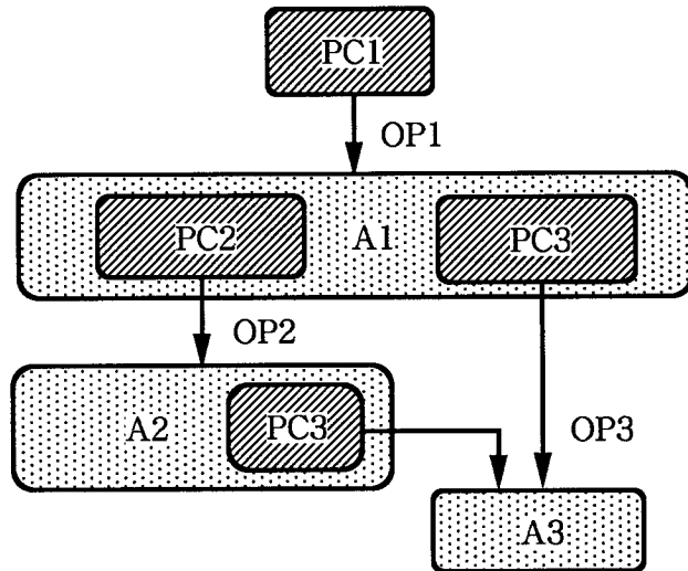
Fig.3.13 完全因果性
