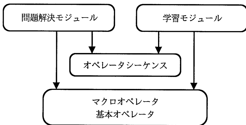
Fig.5.1 PiL2 構成図
