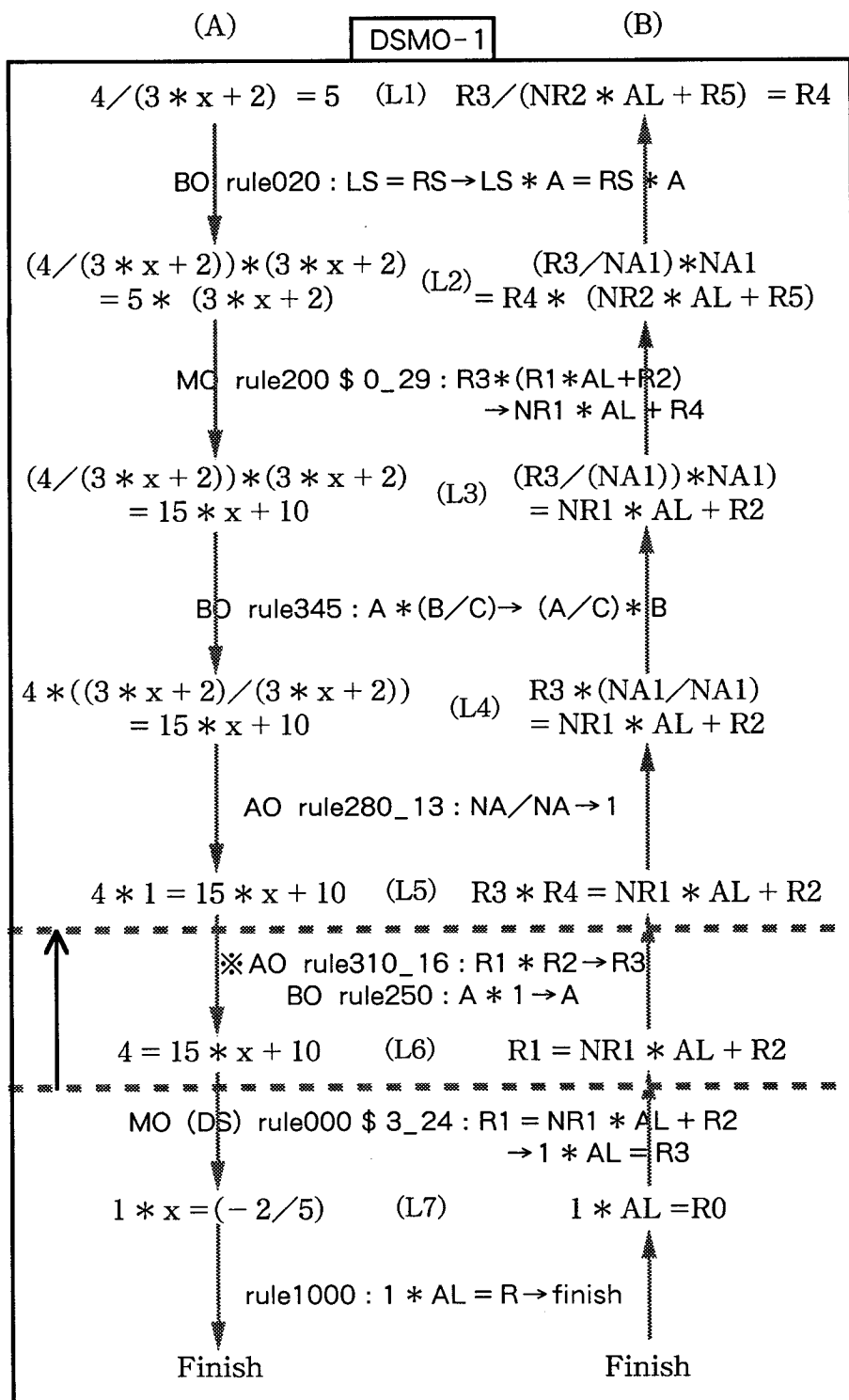
Fig.4.1 分数方程式の解法例
