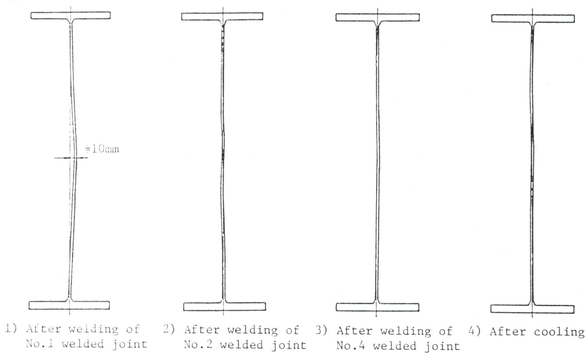
図-4.8 無応力下補修溶接後(Case 2 , 試験体S-2B) における変形の経時変化
