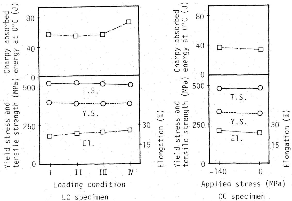
図-2.25 引張試験およびシャルピー衝撃試験結果
