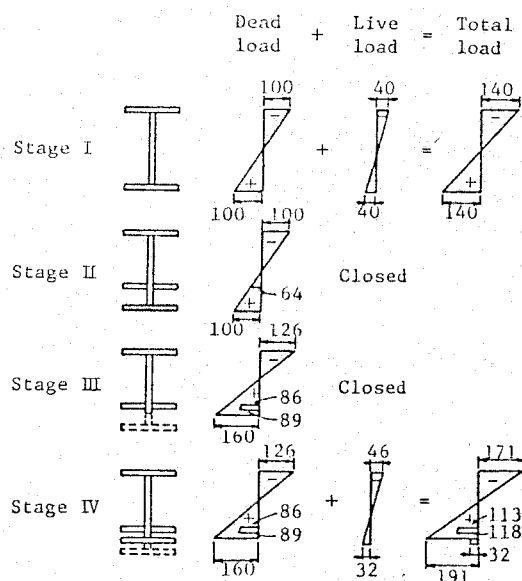
図-3.25 実橋における応力
