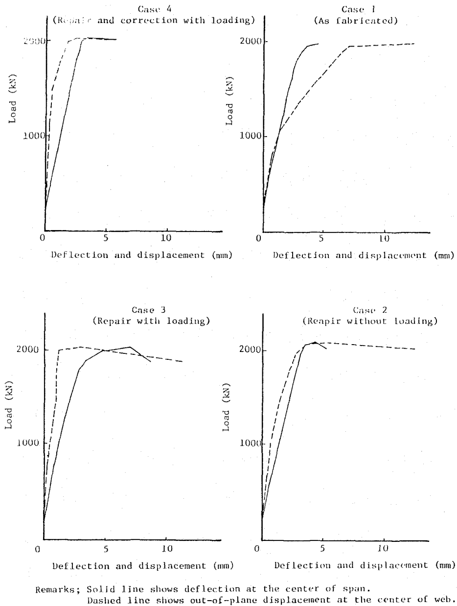
図-4.9 P - \delta 曲線
