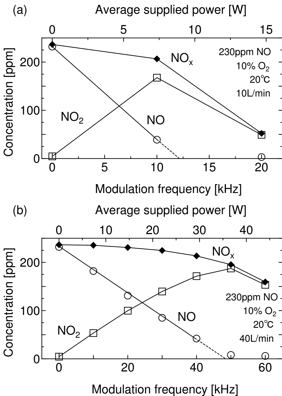
図 6-3. NO, NO 2 , NO x 濃度のプラズマ変調周波数に対する依存性. ガス流量は, (a) 10 L/min, (b) 40 L/min とした. 瞬間的な供給電力は 734 W, パルス幅は 1 \mu s とした.
