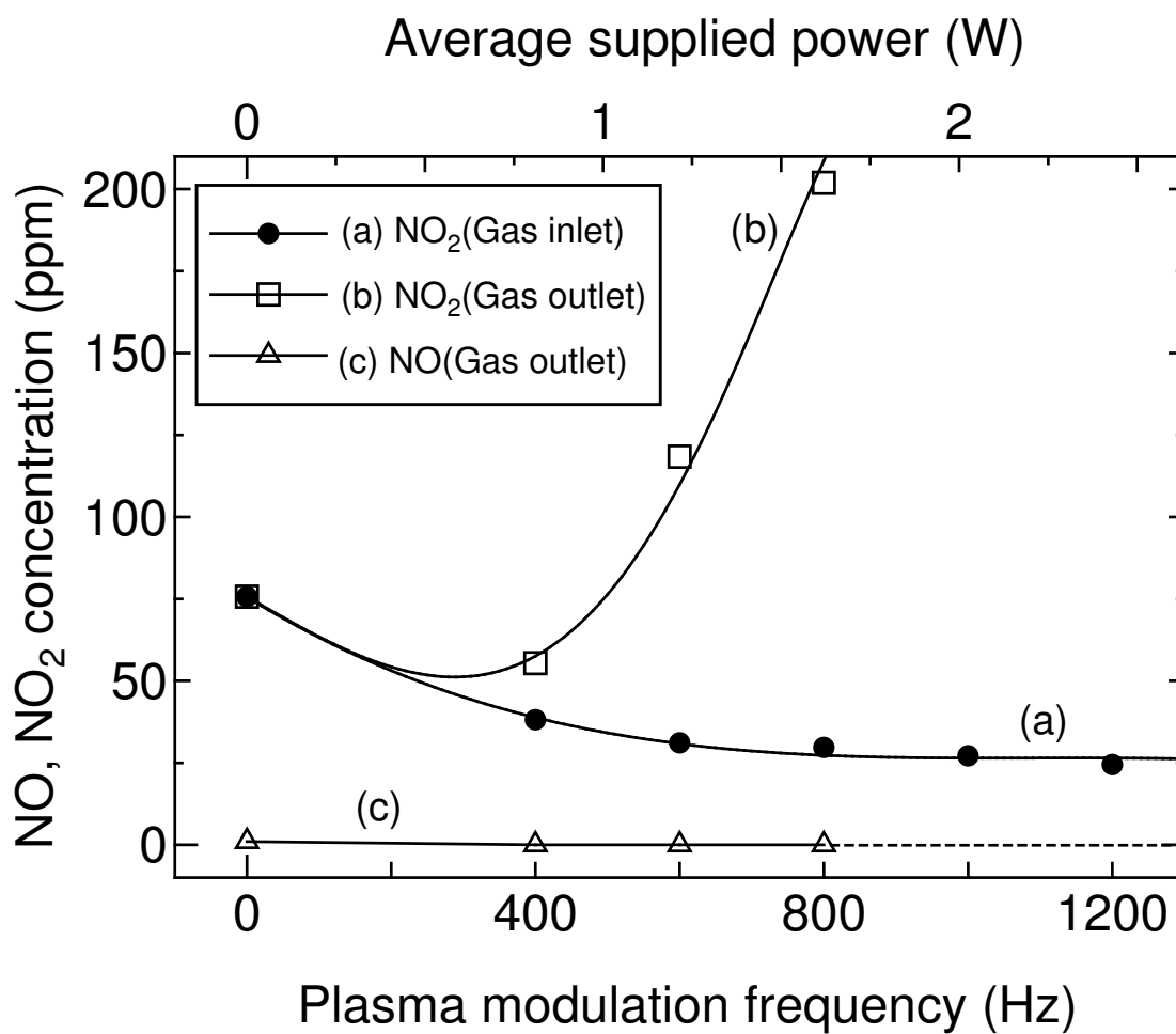
図 7-10. プラズマ装置の入口と出口で測定した NO 2 および NO 濃度のプラズマ変調周波数依存性. (a) (プラズマが生成されている)ガス入口で, QCL 吸収分光法を用いて測定した NO 2 濃度. (b) ガス出口で, 定電位電解法を用いて測定した NO 2 濃度. (c) (b)と同じ場所での NO 濃度. ガス流量は 1.2 L/min である.
