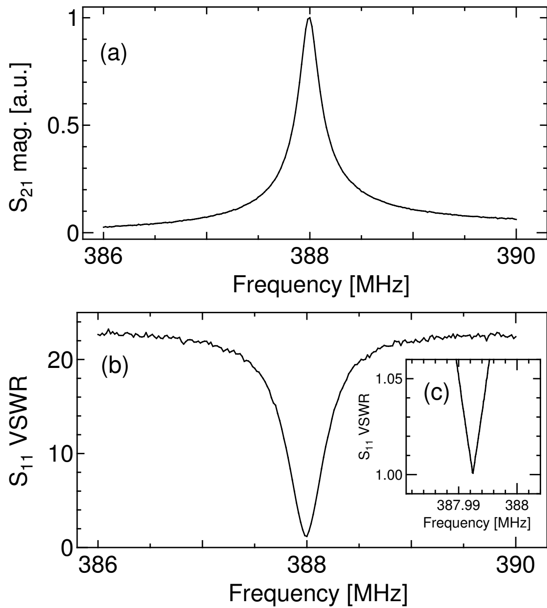
図3-5. 共振型プラズマリアクターにおけるSパラメータの周波数依存性; (a) S_{21} , (b) S_{11} , (c)共振周波数周辺の S_{11} .
