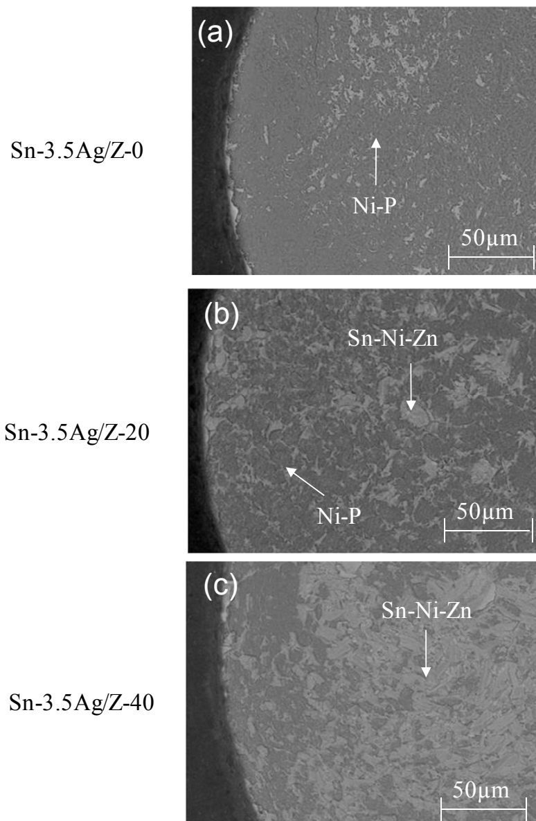
図6.6 マイクロインパクト試験における各接合サンプルの破壊面SEM写真. (衝撃の方向: 左から右)
