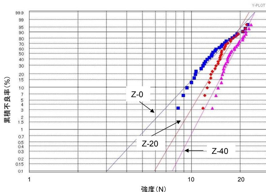
図6.2 各接合サンプルの初期プル強度に関するワイブルプロット。
