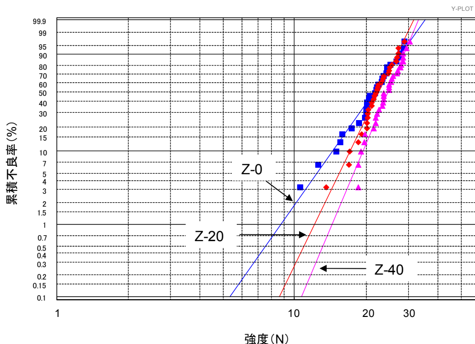
図6.4 各接合サンプルの初期衝撃強度に関するワイブルプロット。
