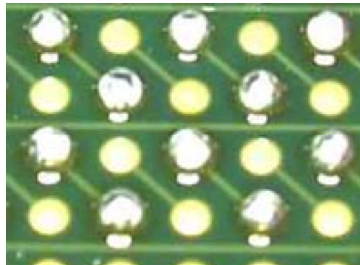
図3.2 BGA接合サンプルの外観写真.
