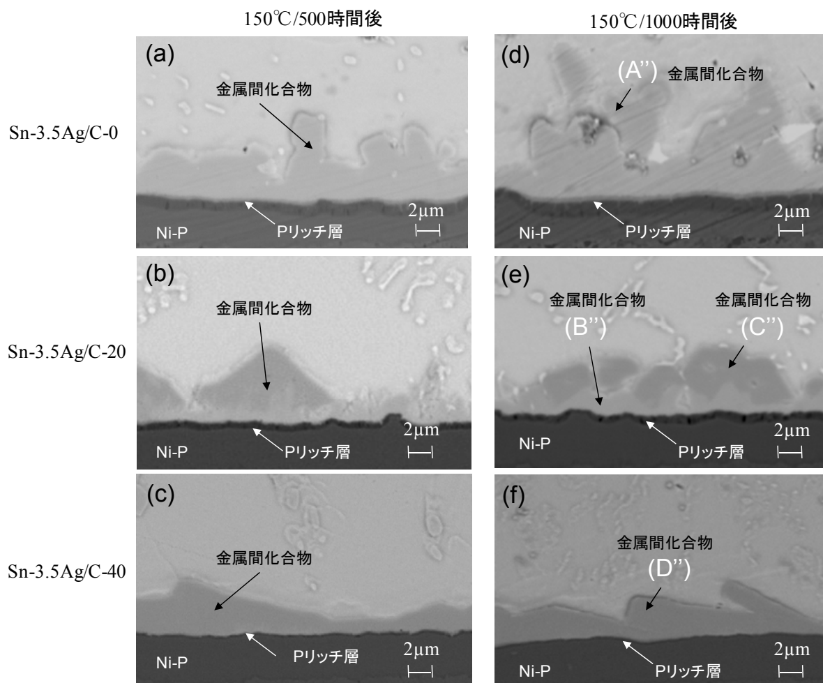
図3.11 150℃エージング処理を施した各接合サンプルの断面SEM観察写真.
