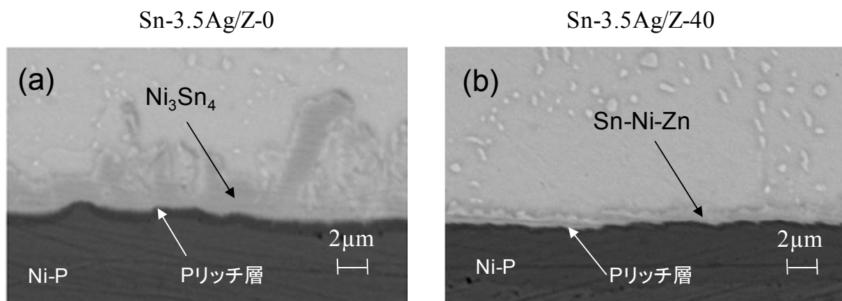
図5.8 85°C/85% RH / 500時間放置後の各接合サンプルの断面SEM観察写真.
