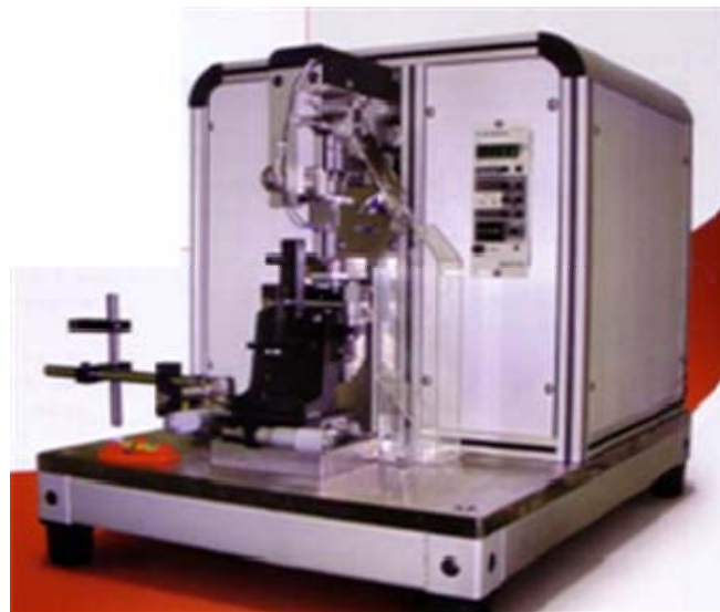
図4.3 マイクロインパクト試験装置の外観写真.
