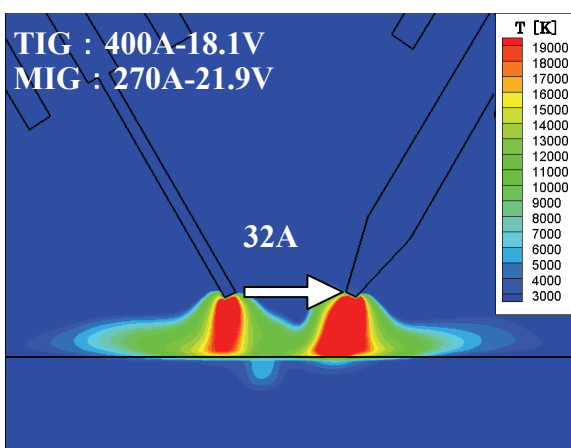
(5) TIG 400A
