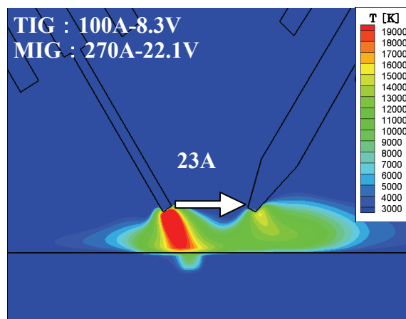
(2) TIG 100A
