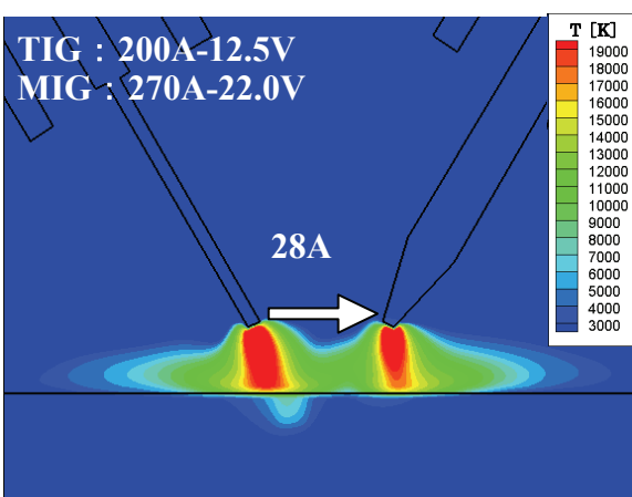
(3) TIG 200A
