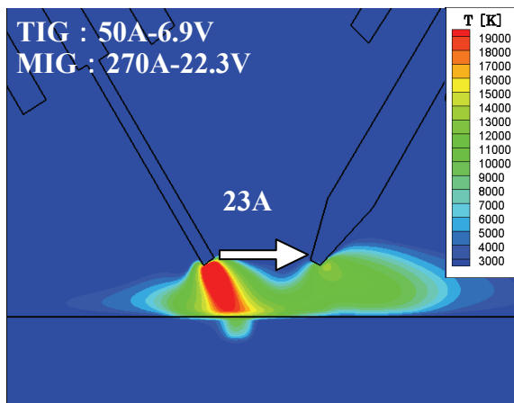
(1) TIG 50A
