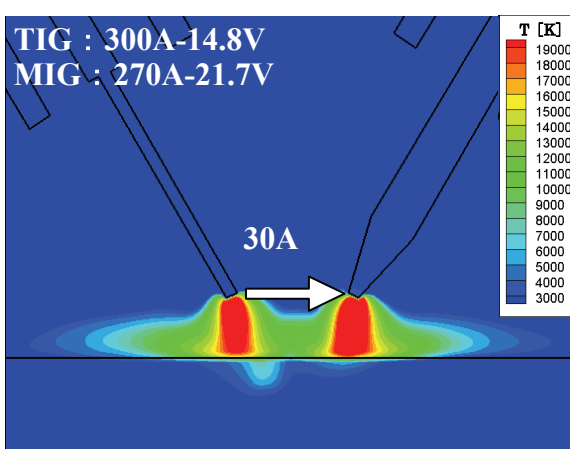
(4) TIG 300A
