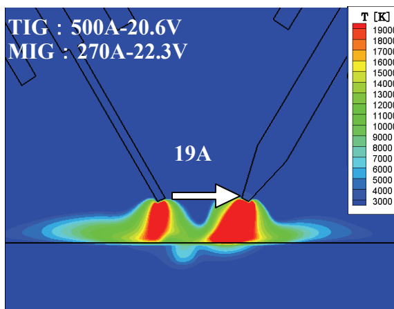
(6) TIG 500A
